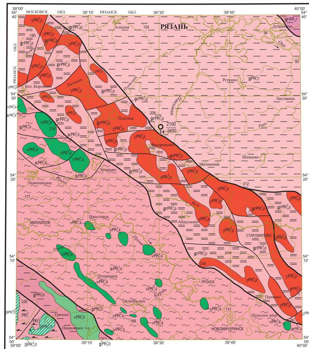
СХЕМА ГЕОЛОГИЧЕСКОГО СТРОЕНИЯ КРИСТАЛЛИЧЕСКОГО ФУНДАМЕНТА (составлена по геофизическим данным ФГБУ "ВСЕГЕИ")
