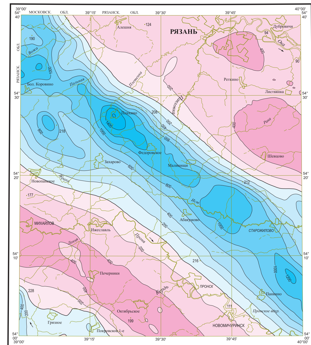
КАРТА АНОМАЛЬНОГО МАГНИТНОГО ПОЛЯ
