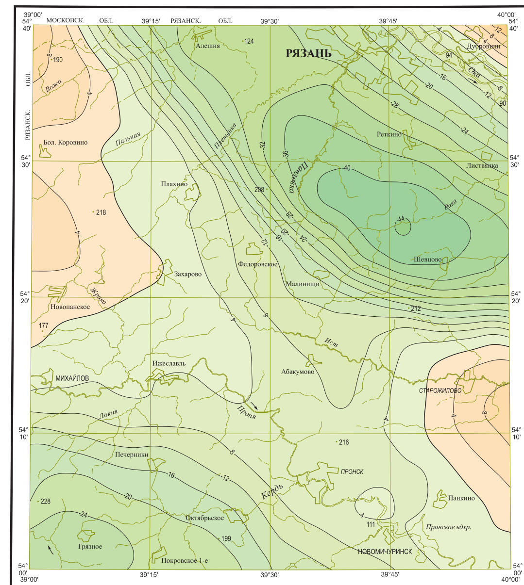
СХЕМА ГРАВИТАЦИОННЫХ АНОМАЛИЙ (оцифровка условная)
