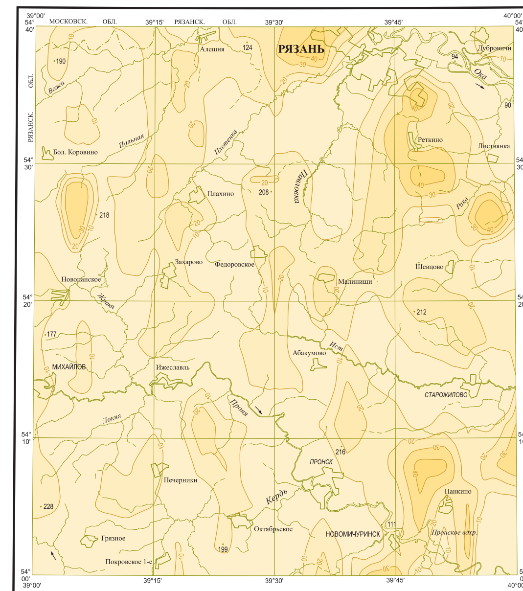
АЛЬПИЙСКИЙ (СЕНОМАНСКО-ГОЛОЦЕНОВЫЙ) СТРУКТУРНЫЙ ЯРУС
