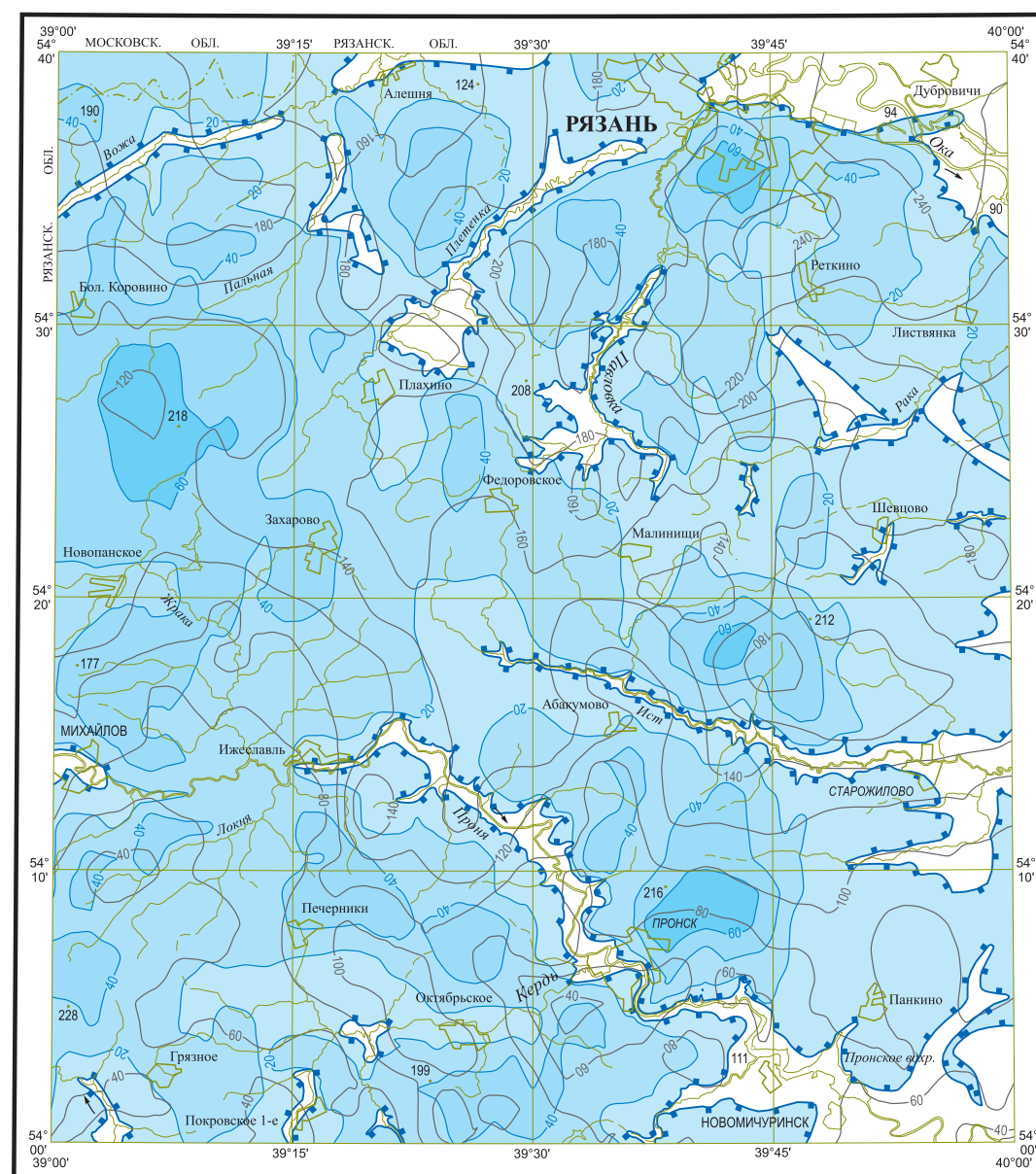
КИММЕРИЙСКИЙ (ВЕРХНЕБАЙОССКО-СРЕДНЕАПТСКИЙ) СТРУКТУРНЫЙ ЯРУС
