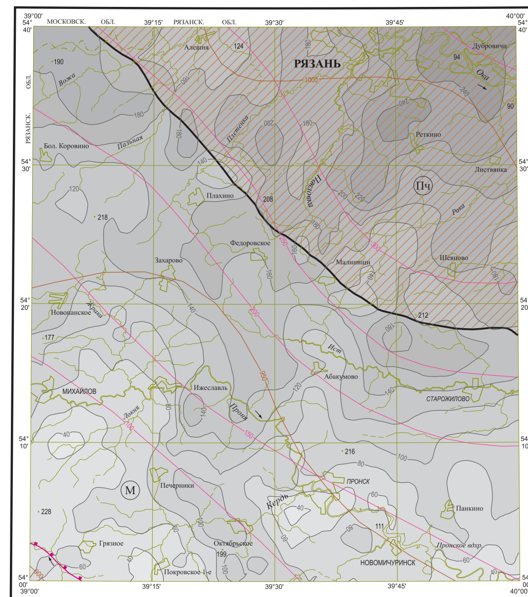
НИЖНЕБАЙКАЛЬСКИЙ (РИФЕЙ-НИЖНЕВЕНДСКИЙ) – ВЕРХНЕГЕРЦИНСКИЙ (ВЕРХНЕВИЗЕЙСКО-МОСКОВСКИЙ) СТРУКТУРНЫЕ ЯРУСЫ
