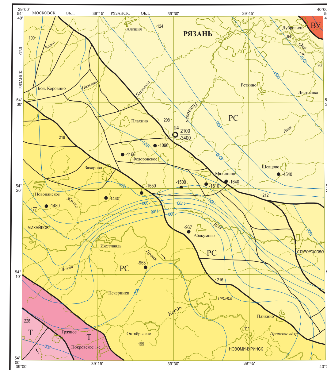
СХЕМА ТЕКТОНИЧЕСКОГО РАЙОНИРОВАНИЯ КРИСТАЛЛИЧЕСКОГО ФУНДАМЕНТА (составлена по геофизическим данным ФГБУ "ВСЕГЕИ")
