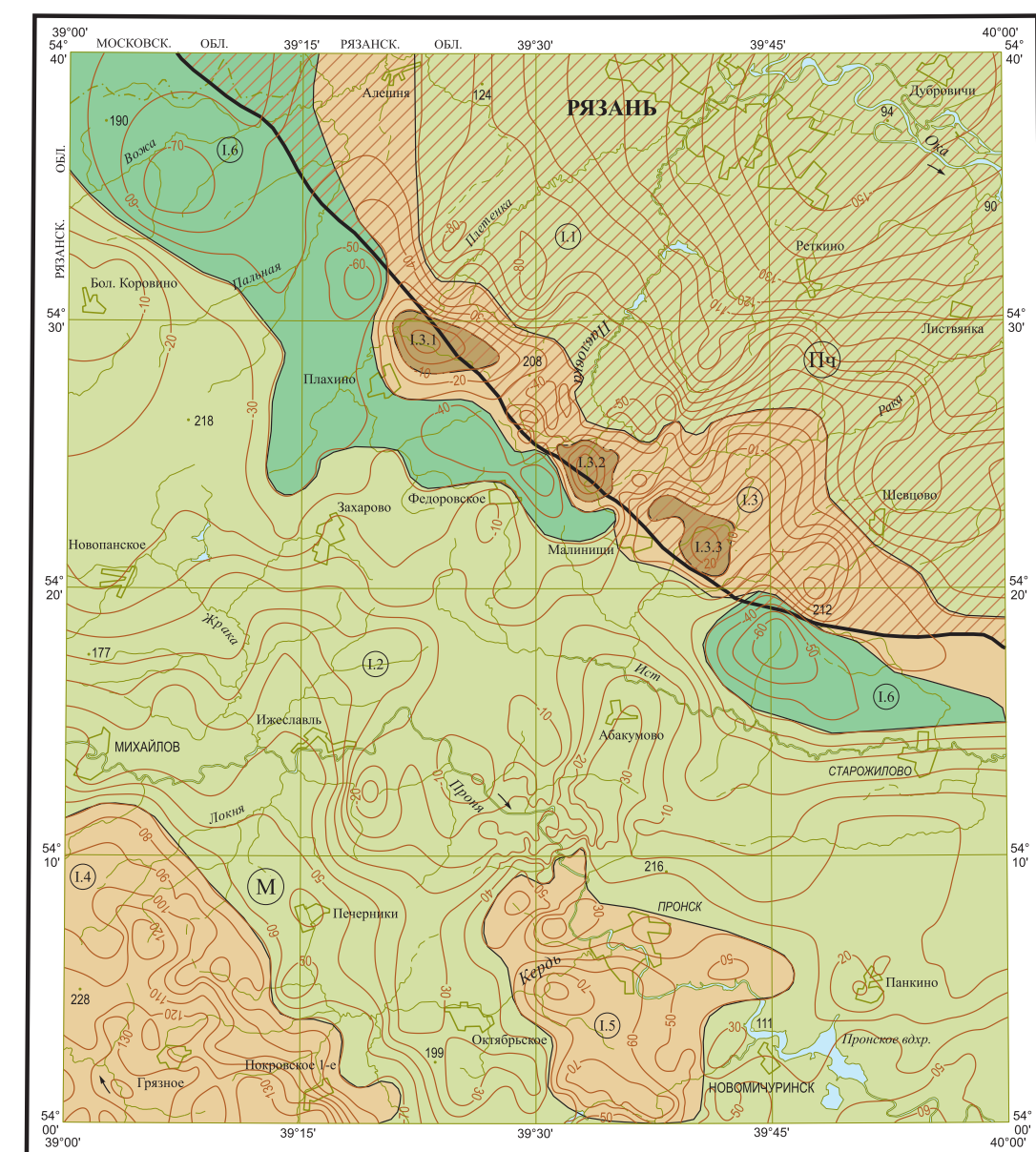
СХЕМА ТЕКТОНИЧЕСКОГО РАЙОНИРОВАНИЯ ОСАДОЧНОГО ЧЕХЛА
