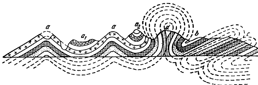
Рис. 6. Формы складок:
