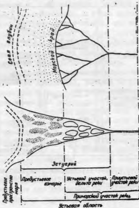
Рис.9. Районирование устьевой области реки (по И.В.Самойлову, 1952)
