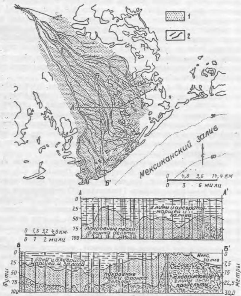
Рис. 12. Покровные пески фронта дельты р. Миссисипи (по Х. Н. Фиску, 1955)
