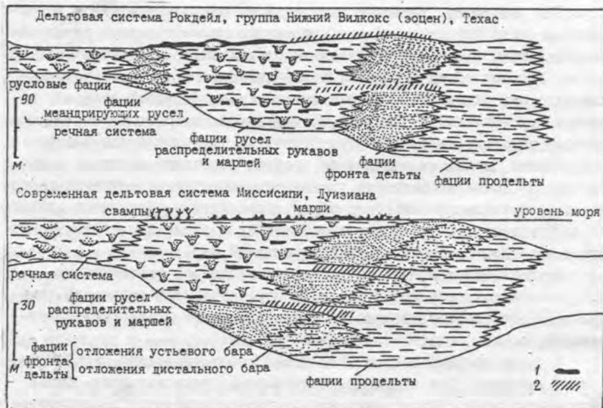
Рис.2. Сравнение фаций современной дельты р.Миссисипи и эоценовой дельтовой системы Рокдейл [19]
