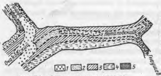
Рис.10. Схема распределения донных отложений в узле разветвления водотоков Очаковский - Потаповский - Прорва (Кикийская дельта Дуная) в августе 1973 г. (по В.Н. Михайлову и др., 1977)
