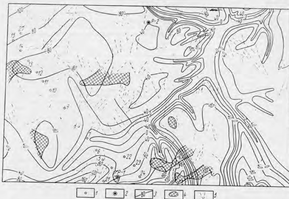
Рис. 3. Схематическая гипсометрическая карта поверхности дочетвертичных отложений с контурами газобиохимических аномалий (составил В. А. Демидов по материалам ГУЦР и ВНИИЯГГ)
