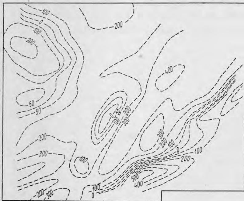
Рис. 1. Карта изодинам \Delta T_{\alpha} (по данным В. Н. Мосина и Н. С. Никитина)
