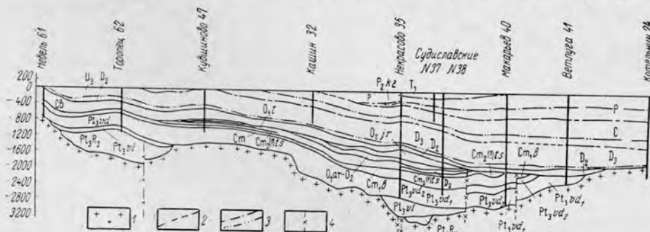
Рис. 2. Геологический разрез по линии Невель — Котельнич (составили Б. А. Яковлев, В. И. Пилишкина)
