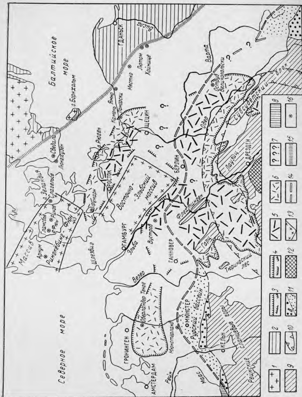
Рис. 1. Схема тектоники северной части Средней Европы.
