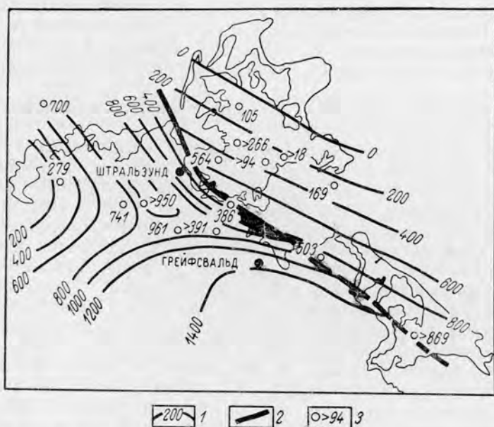
Рис. 2. Схема мощностей эффузивов ротлигендеса в северной части ГДР (по В. Росту и В. Шиманскому [27])
