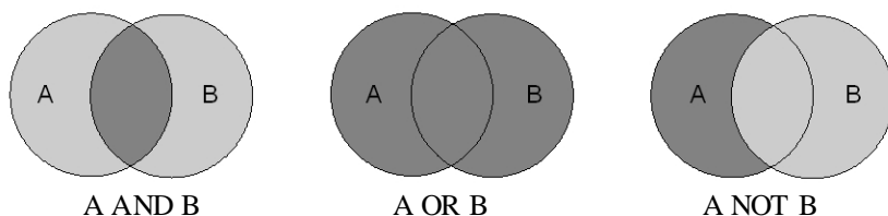
Рис. 5.5.3 – Диаграммы Венна
