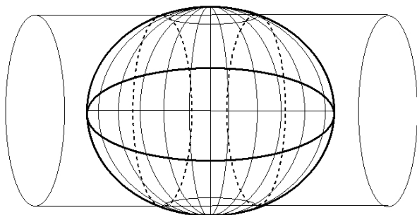
Рис. 3.3.14 - Проекция UTM
