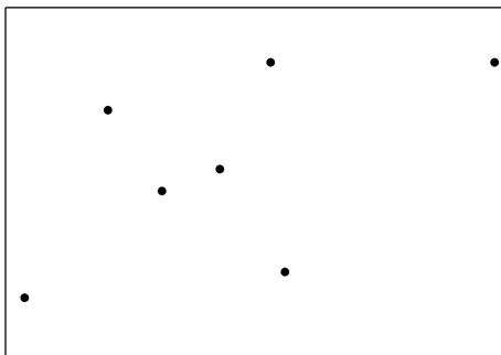
Рис. 2.5.6 - Множество точек
