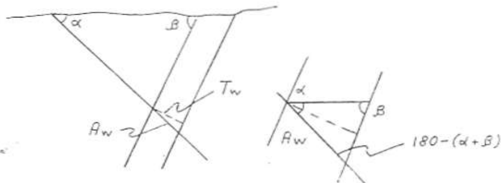
Рис. 2. Бурение перпендикулярно простиранию
