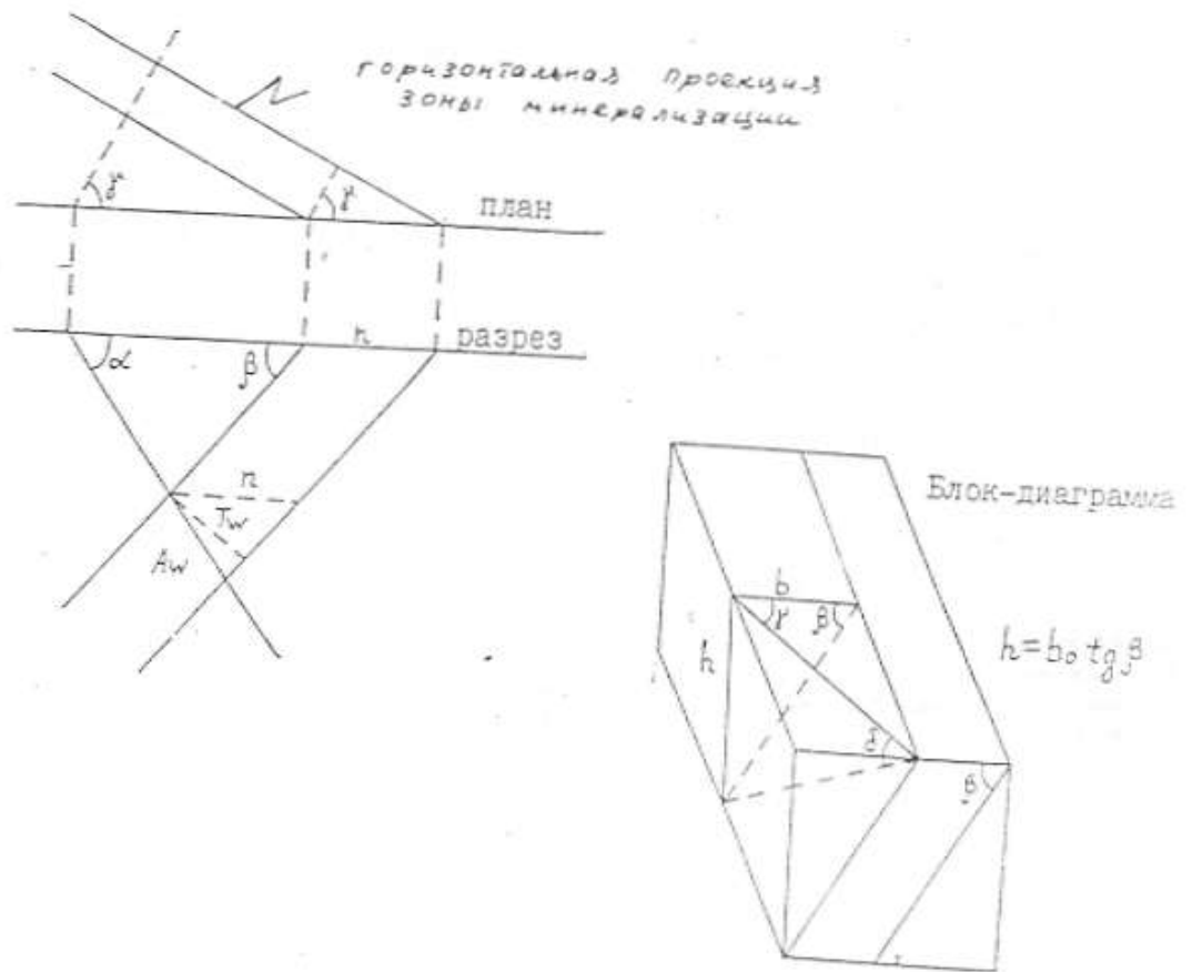
Рис. 3 Бурение под углом к простиранию
