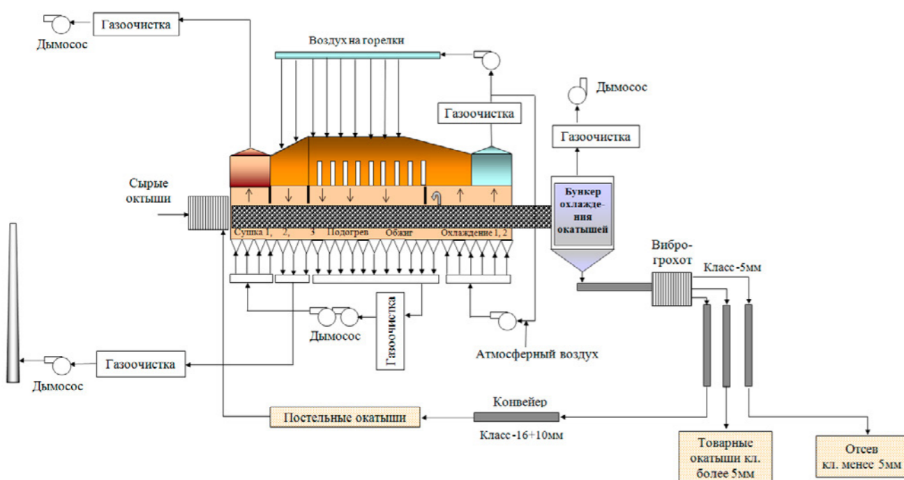
Рисунок 2.18 — Обобщенная схема термической обработки окатышей на обжиговой машине конвейерного типа
