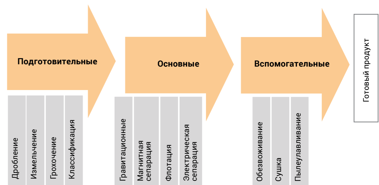
Рисунок 2.6 — Обобщающая схема технологического процесса обогащения
