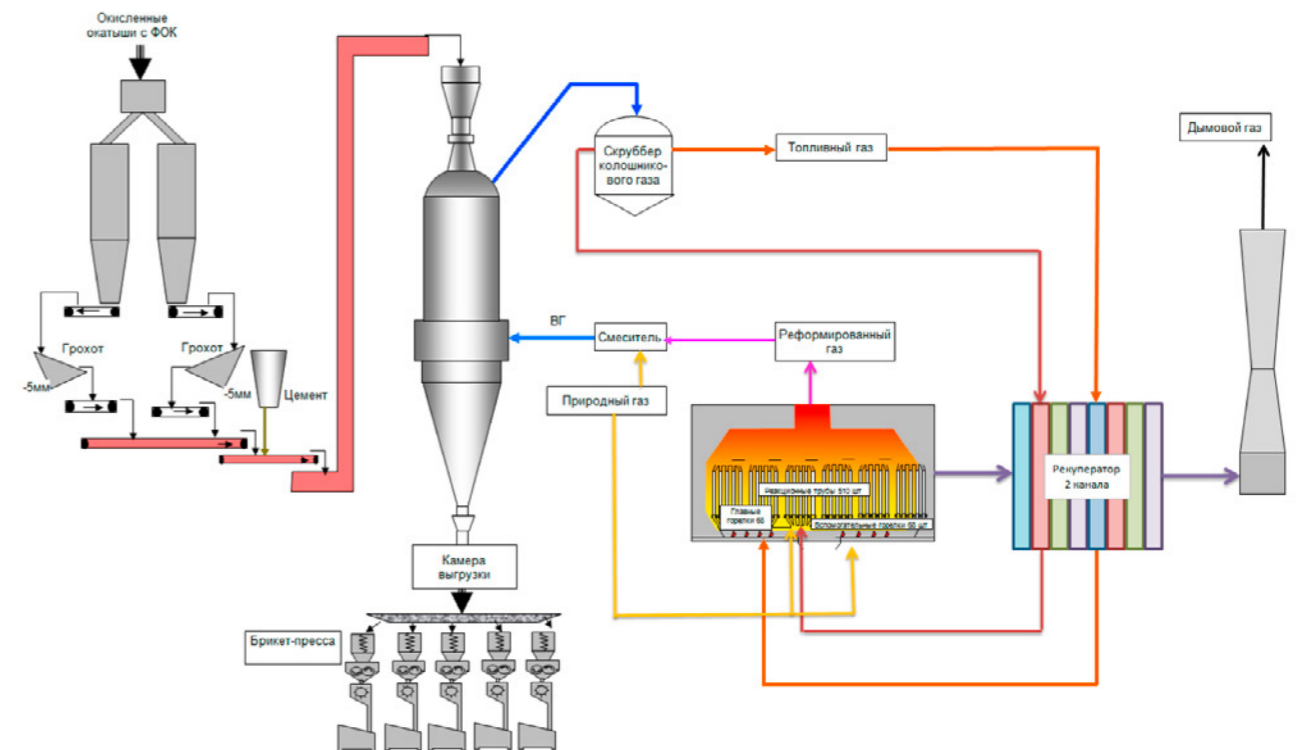
Рисунок 2.34 — Технологическая схема MIDREX
