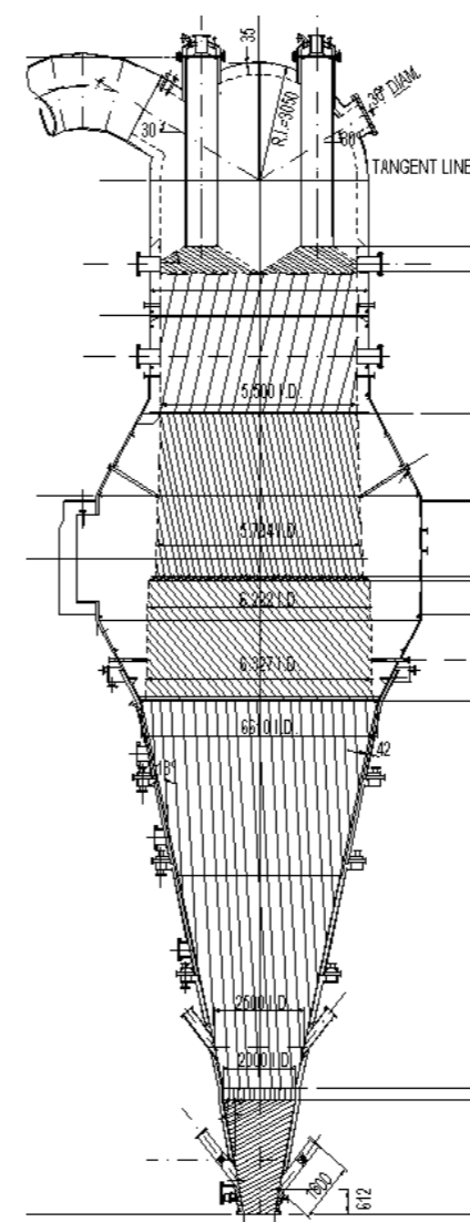
Рисунок 2.35 — Общий вид шахтной печи металлизации HYL III
