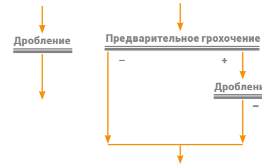
Рисунок 2.8 — Схемы одностадиального дробления в открытом цикле
