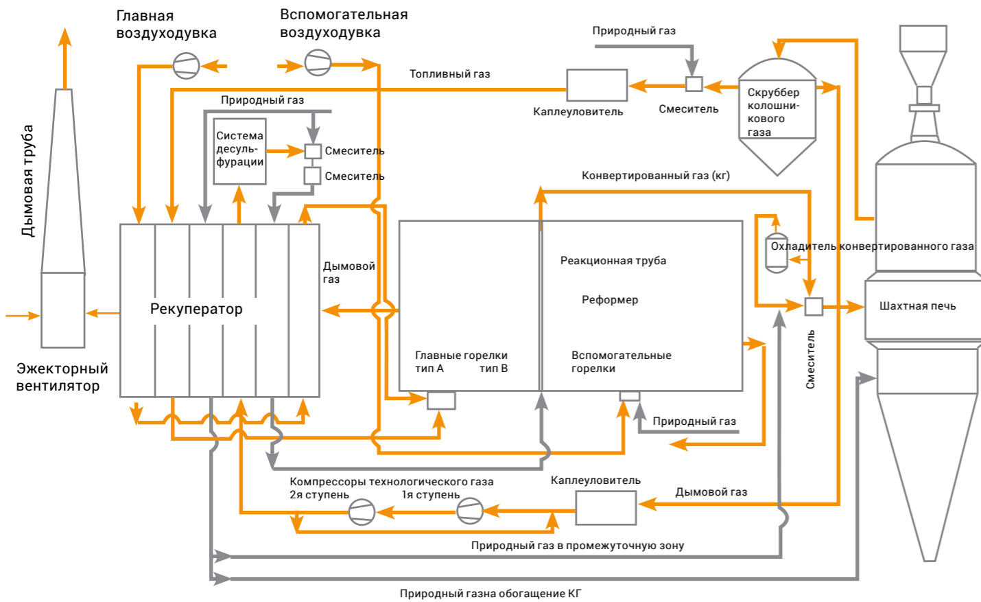
Рисунок 2.45 — Схема потоков технологических газов на установке MIDREX
