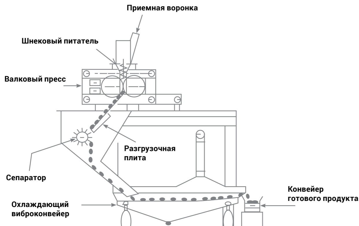
Рисунок 2.50 — Схема установки брикетирования и охлаждения брикетов
