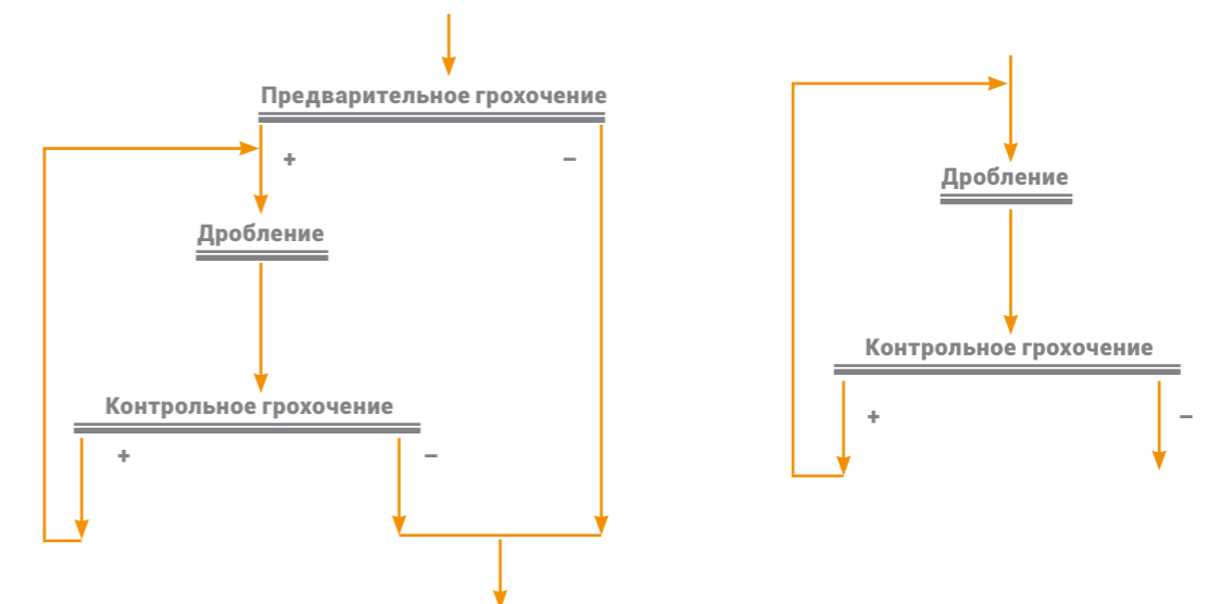
Рисунок 2.9 — Схемы одностадиального дробления в замкнутом цикле
