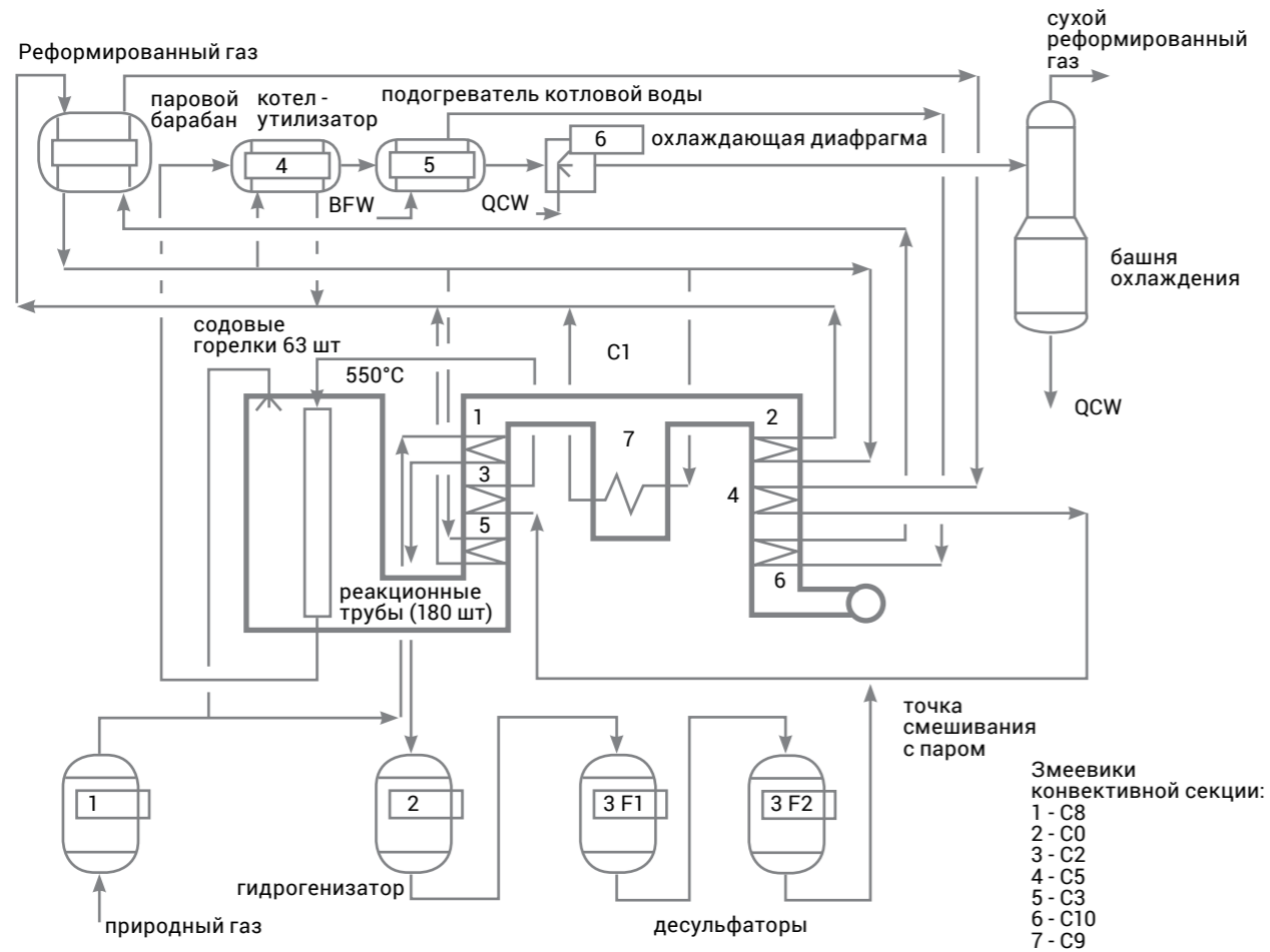
Рисунок 2.40 — Участок по производству реформированного газа на установке HYL III
