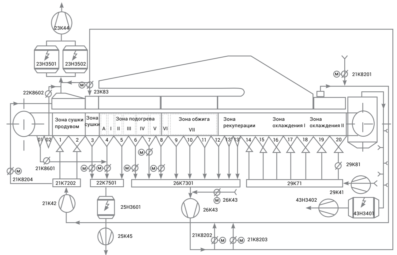
Рисунок 2.25 — Схема газовых потоков обжиговой машины Л 480
