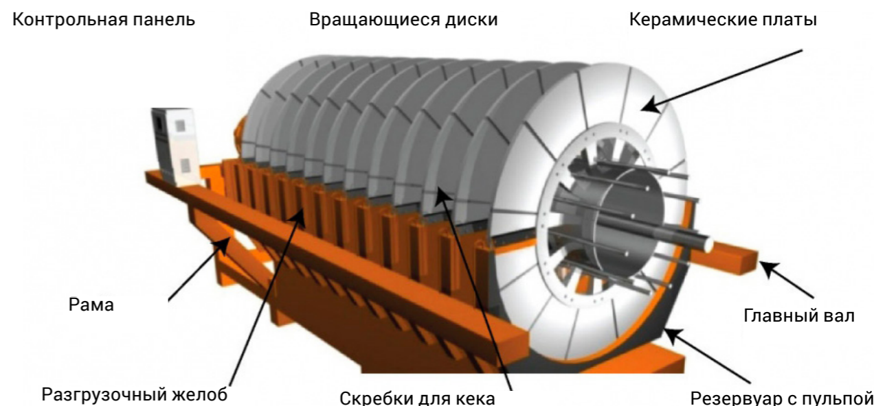
Рисунок 2.12 — Дисковый вакуумный фильтр
