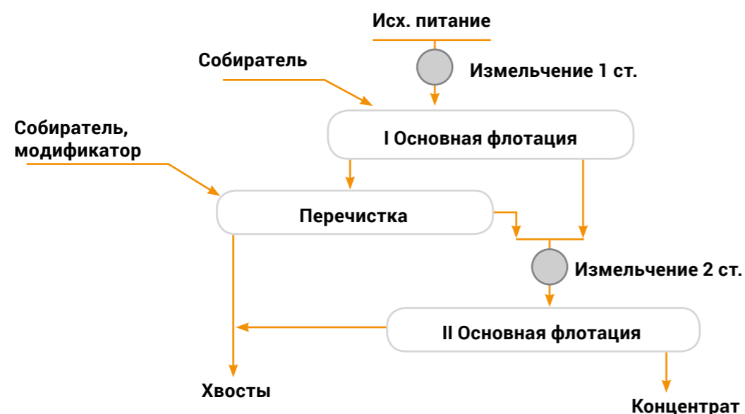
Рисунок 7.10 — Схема двухстадиального флотационного обогащения
