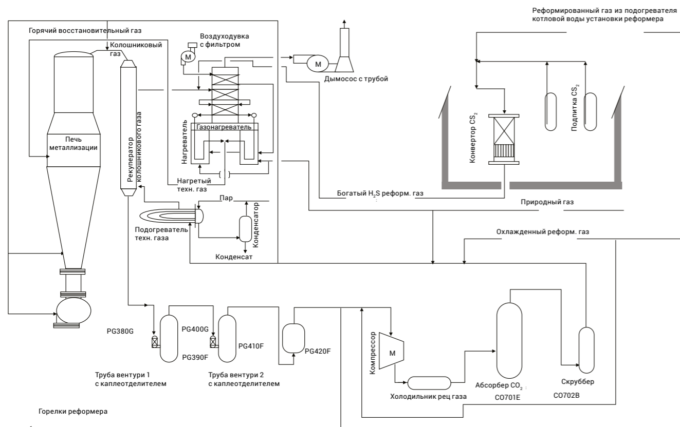
Рисунок 2.43 — Контур технологических газов установки металлзации HYL III
