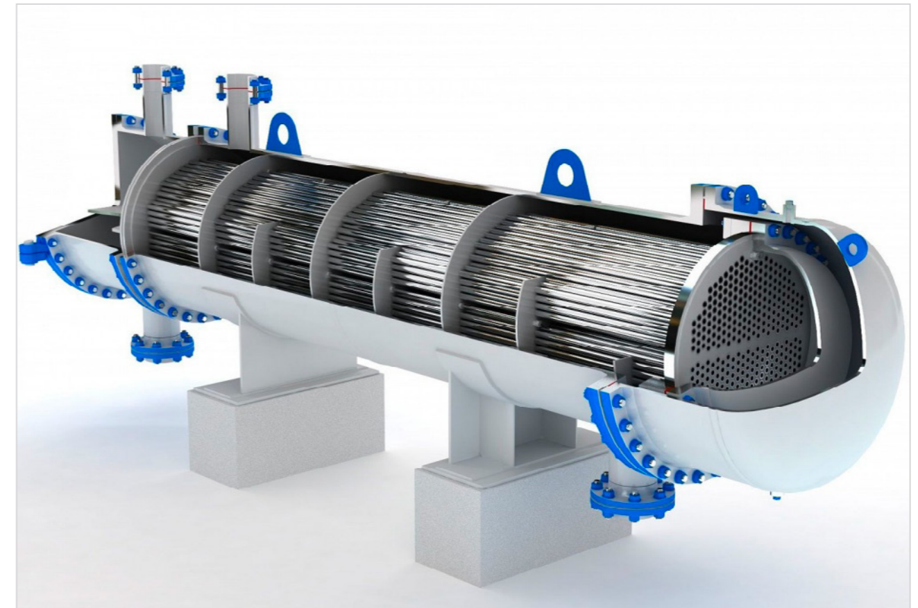
Рисунок 2.46 — Кожухотрубный противоточный рекуператор технологического газа
