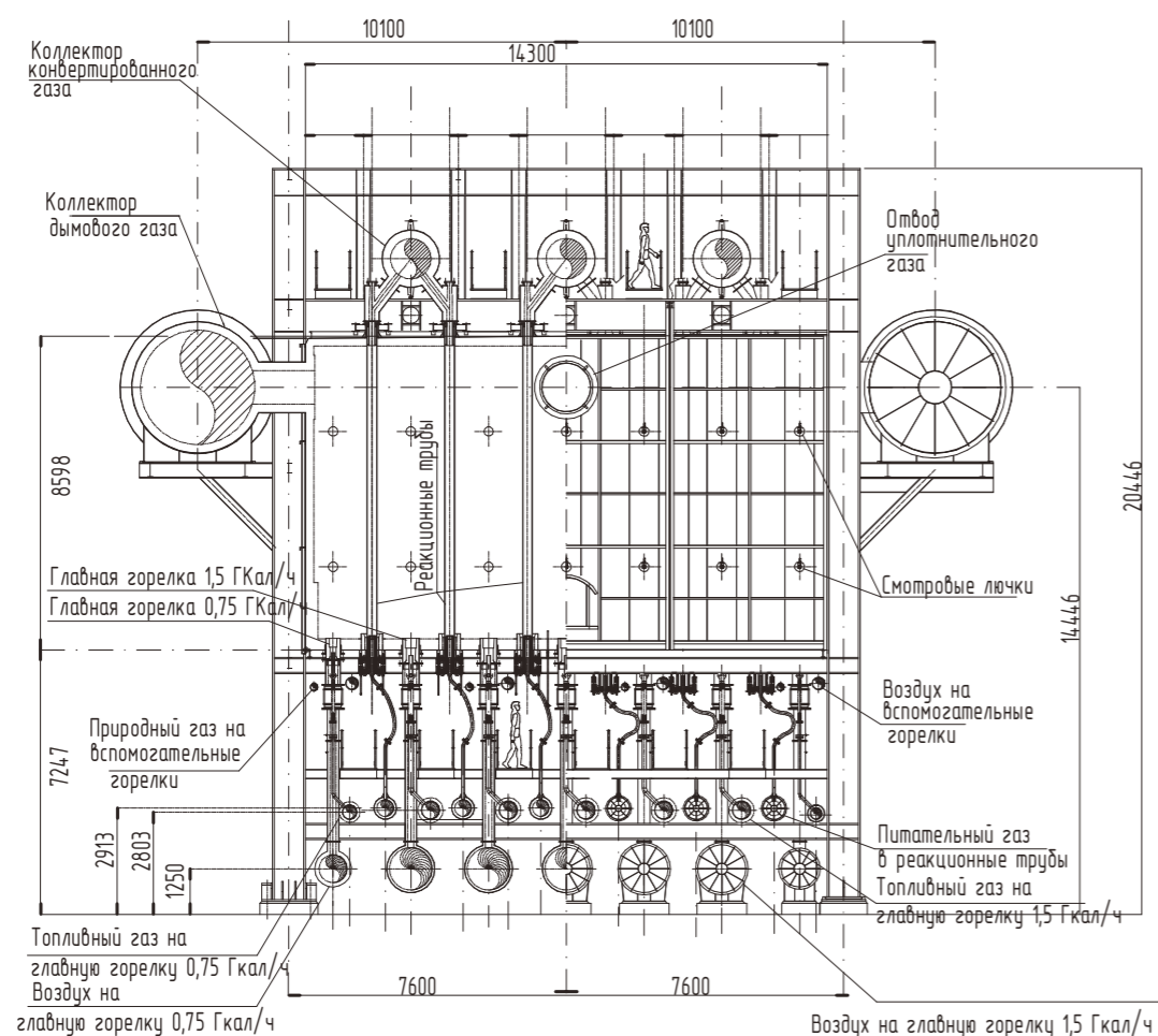
Рисунок 2.41 — Реформер. Фронтальная проекция
