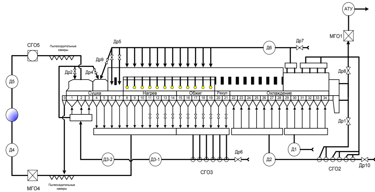
Рисунок 2.22 — Схема газовых потоков обжиговой машины ОК 306
