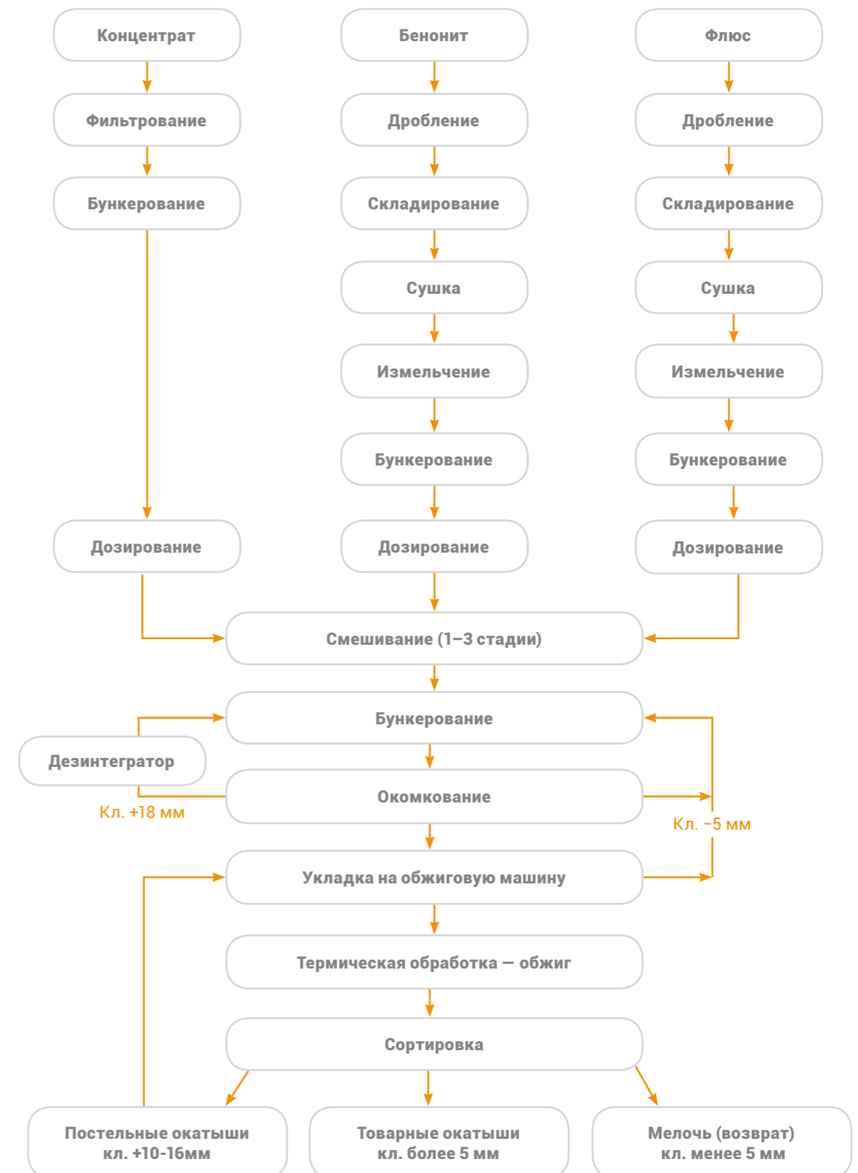
Обобщенная структурная схема производства окатышей
