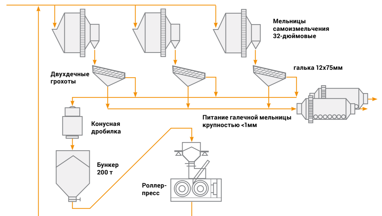
Рисунок 7.9 — Пример размещения роллер-пресса в технологии самоизмельчения
