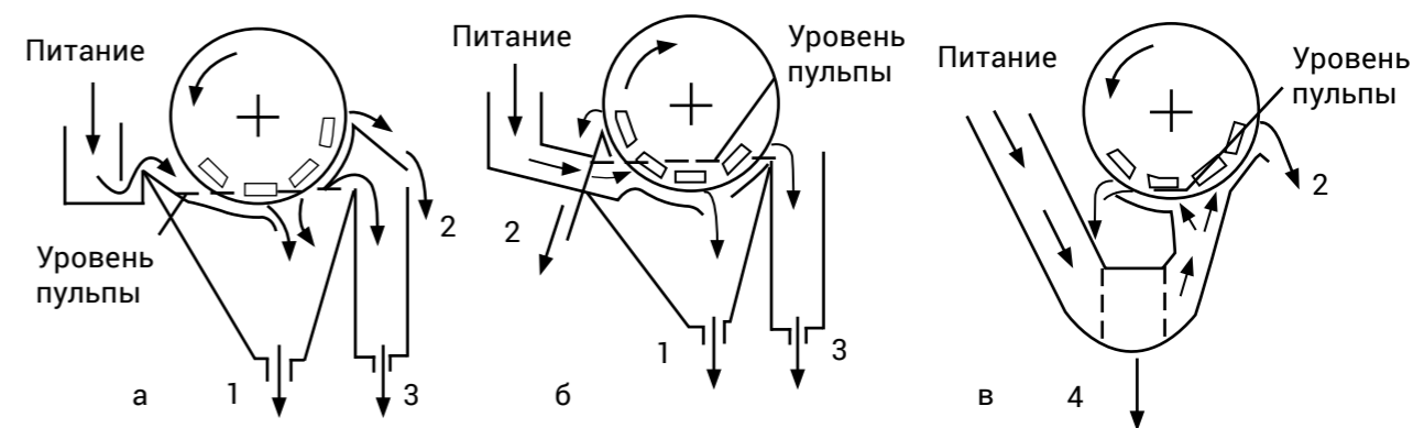
1 — зернистый немагнитный продукт; 2 — магнитный продукт; 3 — тонкозернистый немагнитный продукт; 4 — зернистый и тонкозернистый немагнитные продукты
