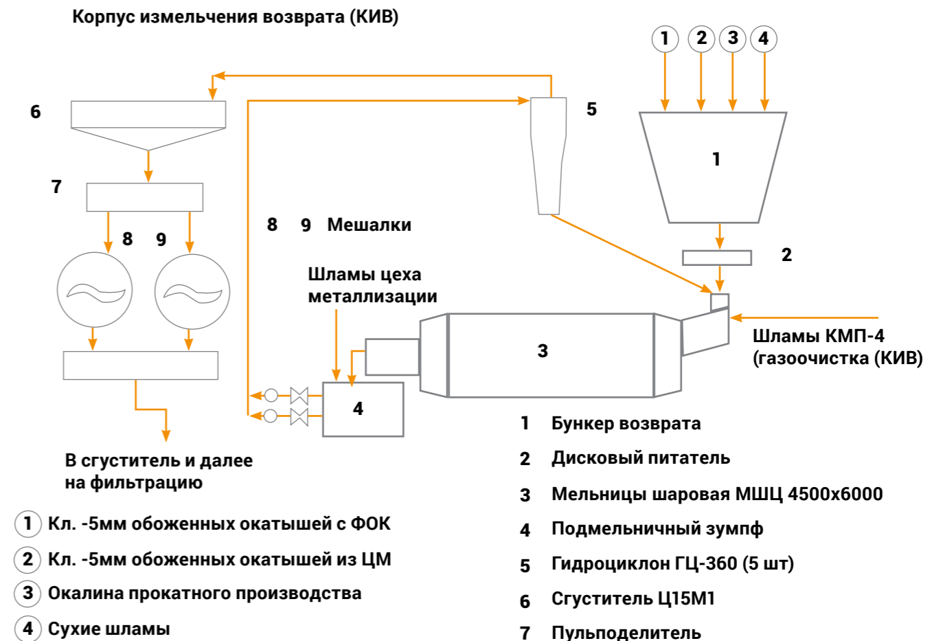
Рисунок 3.6 – Схема использования шламов на ОЭМК
