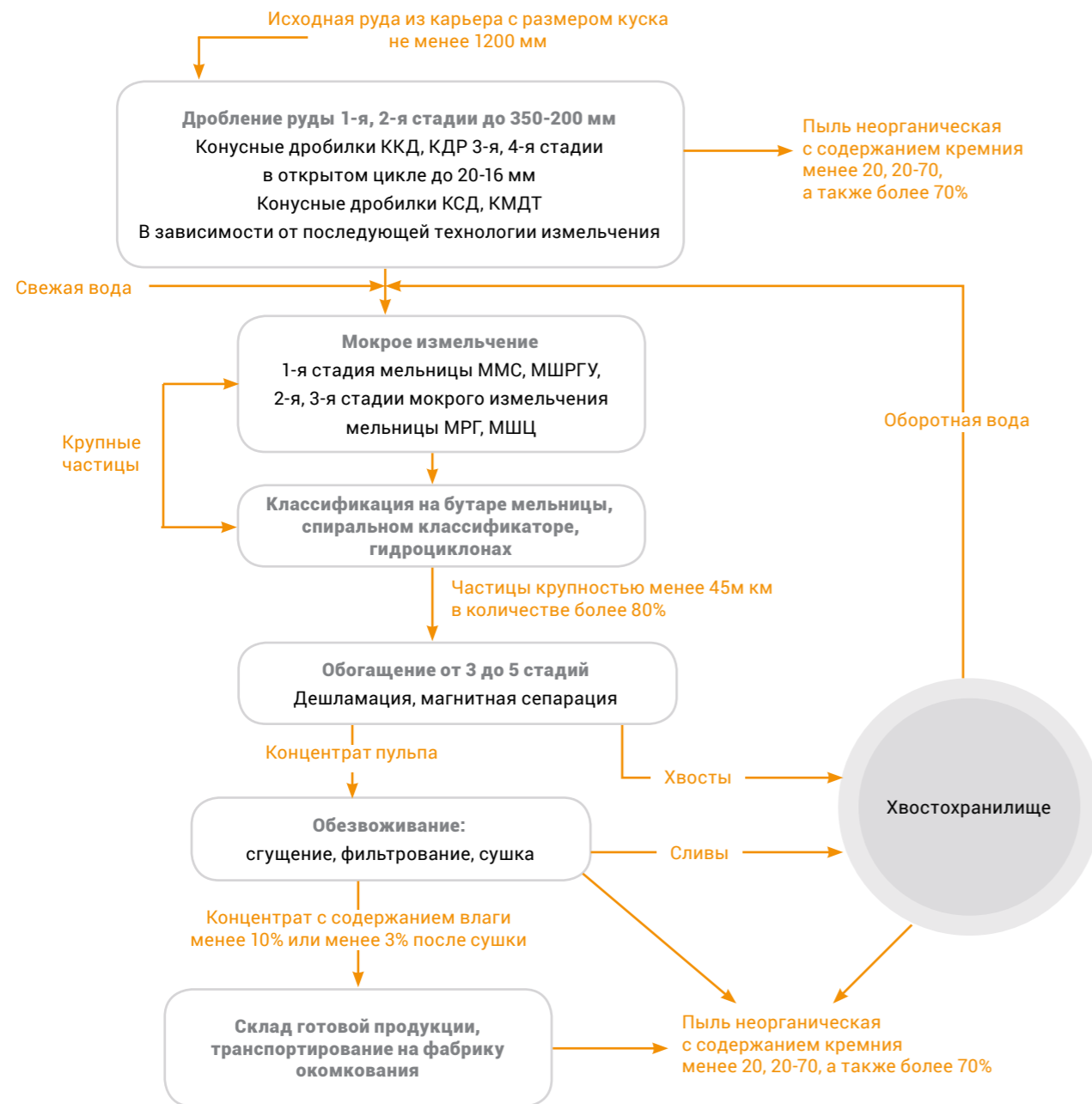
Рисунок 2.7 — Обобщенная структурная схема технологической цепочки обогащения железных руд
