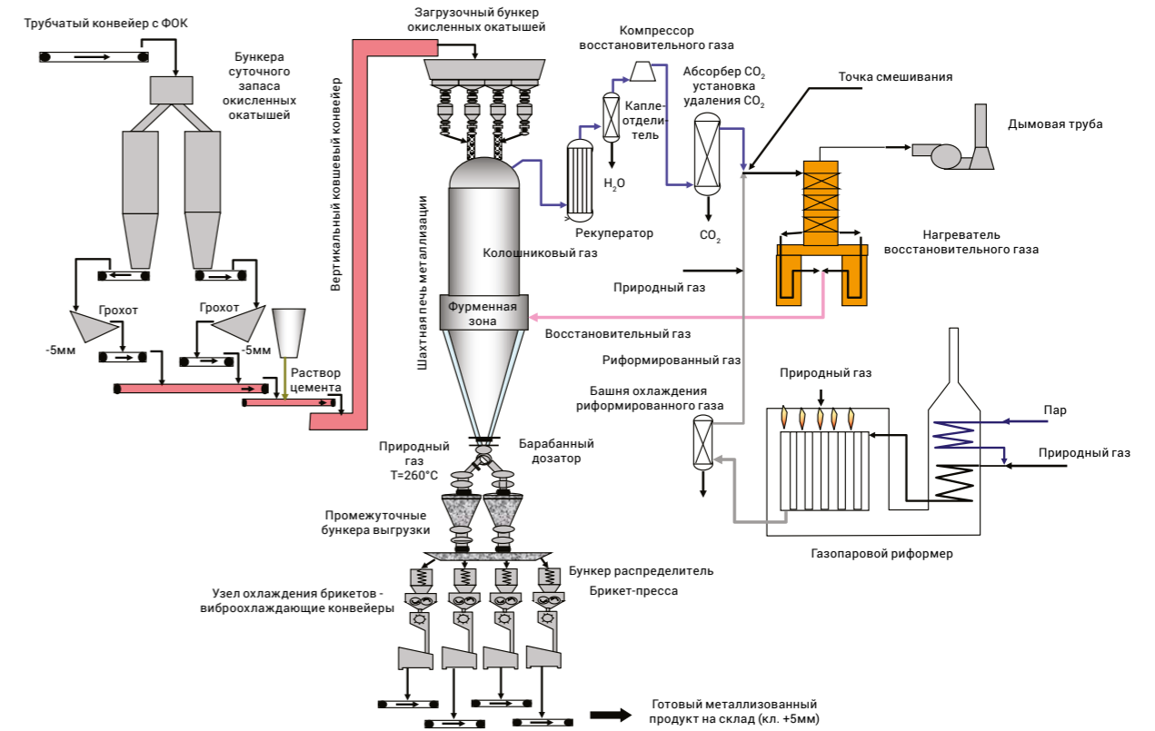
Рисунок 2.33 — Технологическая схема HYL III
