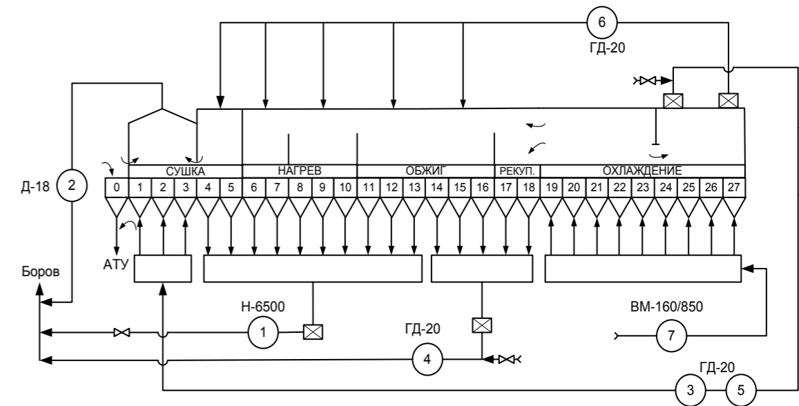
Рисунок 2.20 – Тепловая схема действующей ОК 108
