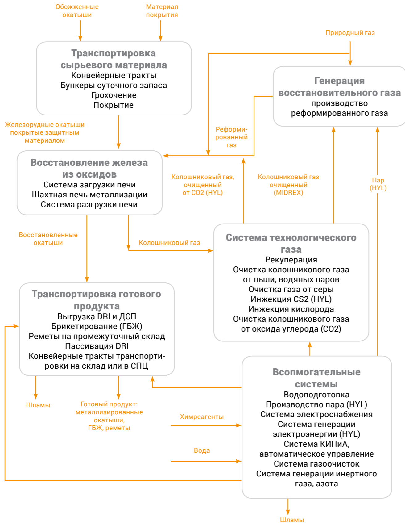
Рисунок 2.32 — Обобщенная технологическая схема производства железа прямого восстановления
