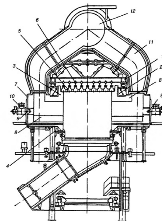
Рисунок 2.27 — Поперечное сечение горна обжиговой машины
