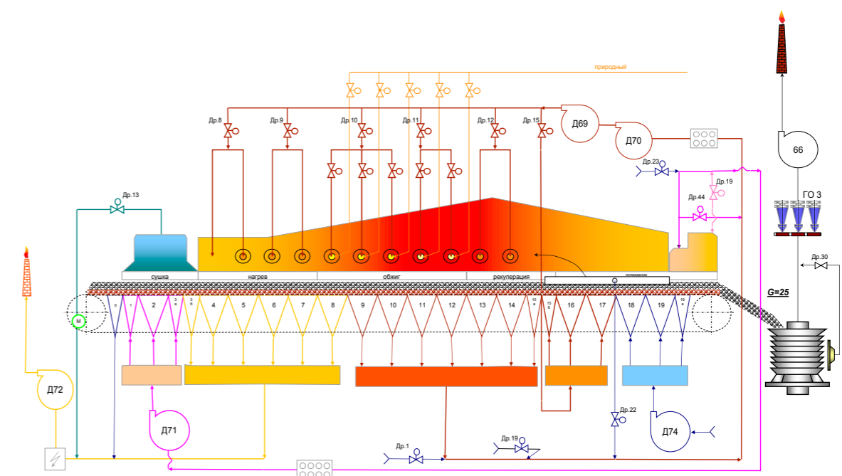
Рисунок 2.21 – Тепловая схема действующей модернизированной ОК 228
