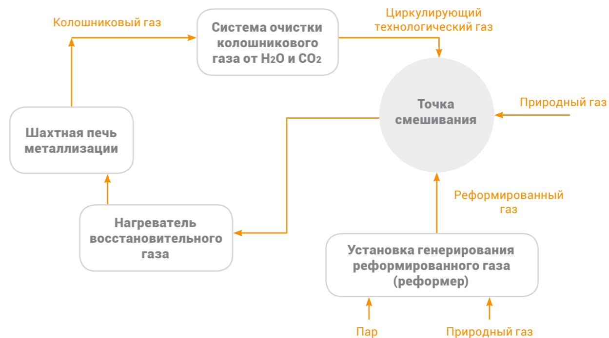
Рисунок 2.44 — Схема циркуляции технологического газа в системе HYL III
