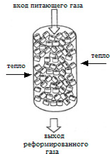
Рисунок 2.42 — Реакционная труба реформера, заполненная катализатором
