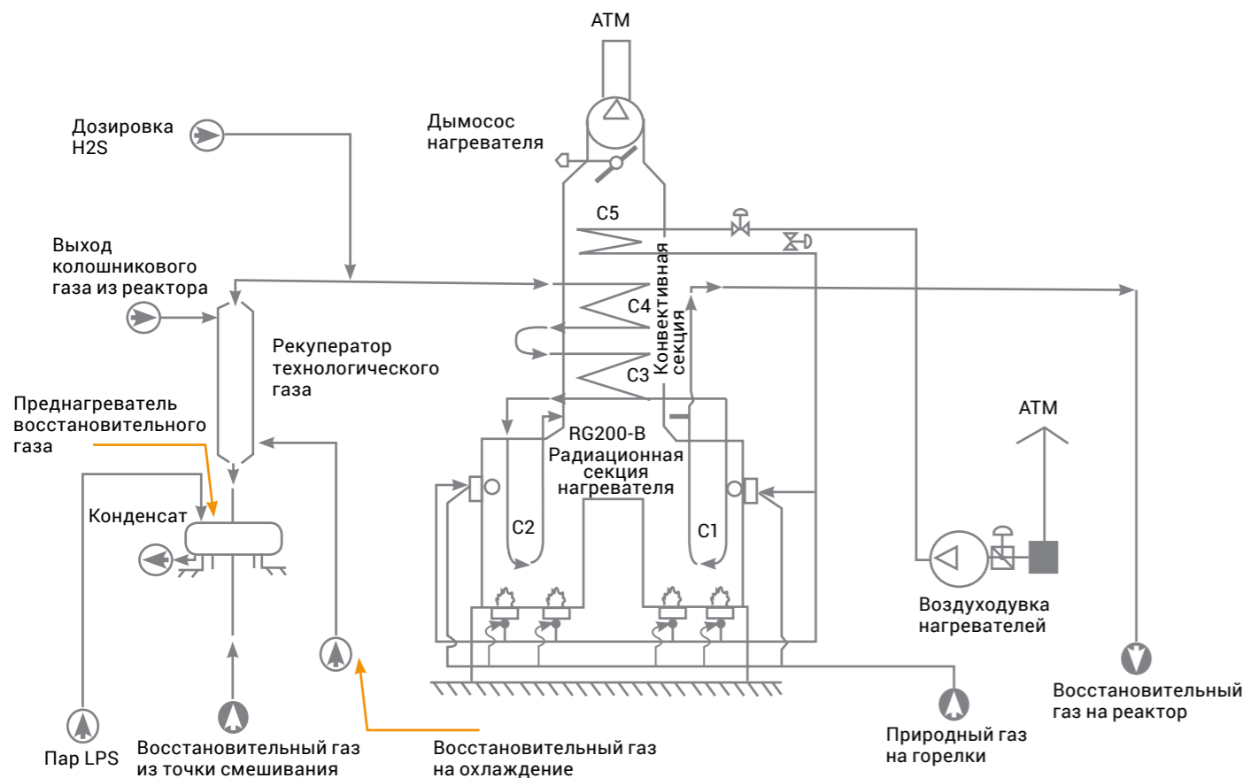
Рисунок 2.47 — Нагреватель восстановительного газа
