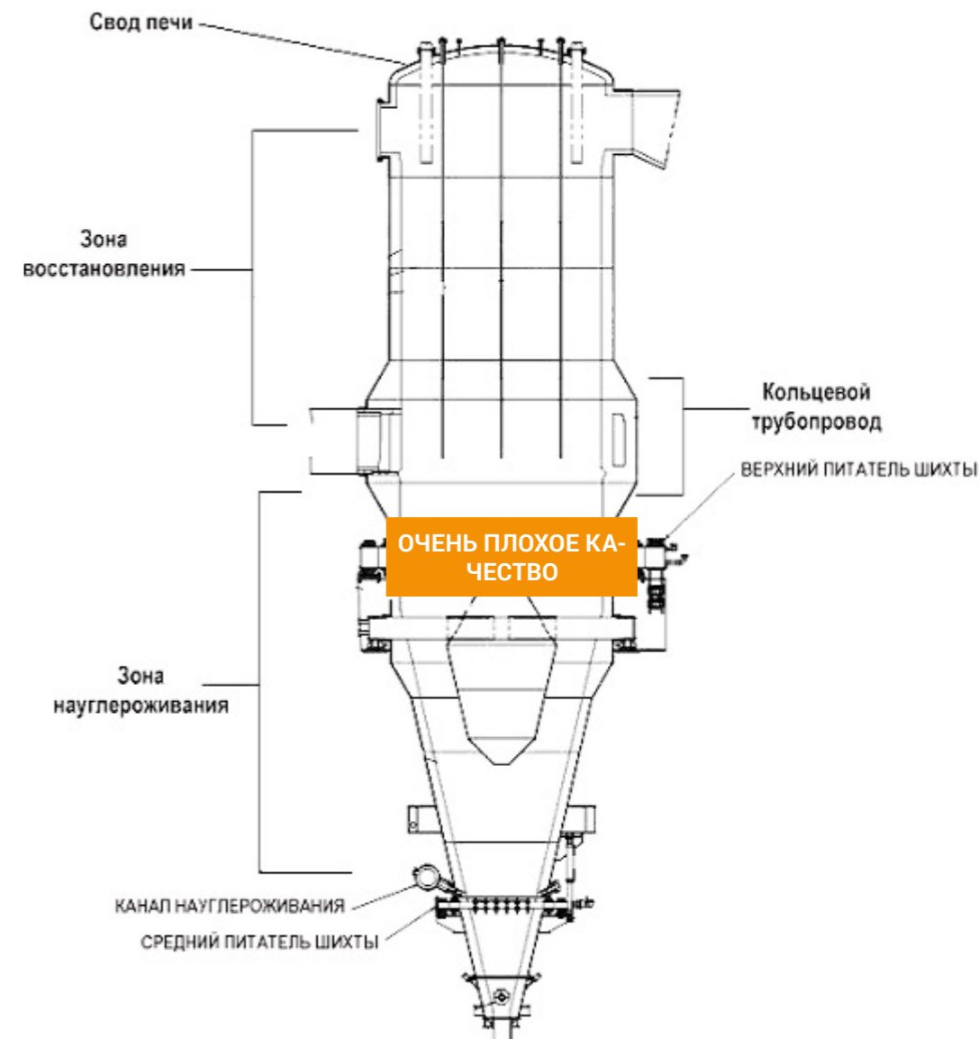
Рисунок 2.37 — Общий вид шахтной печи металлургии MIDREX
