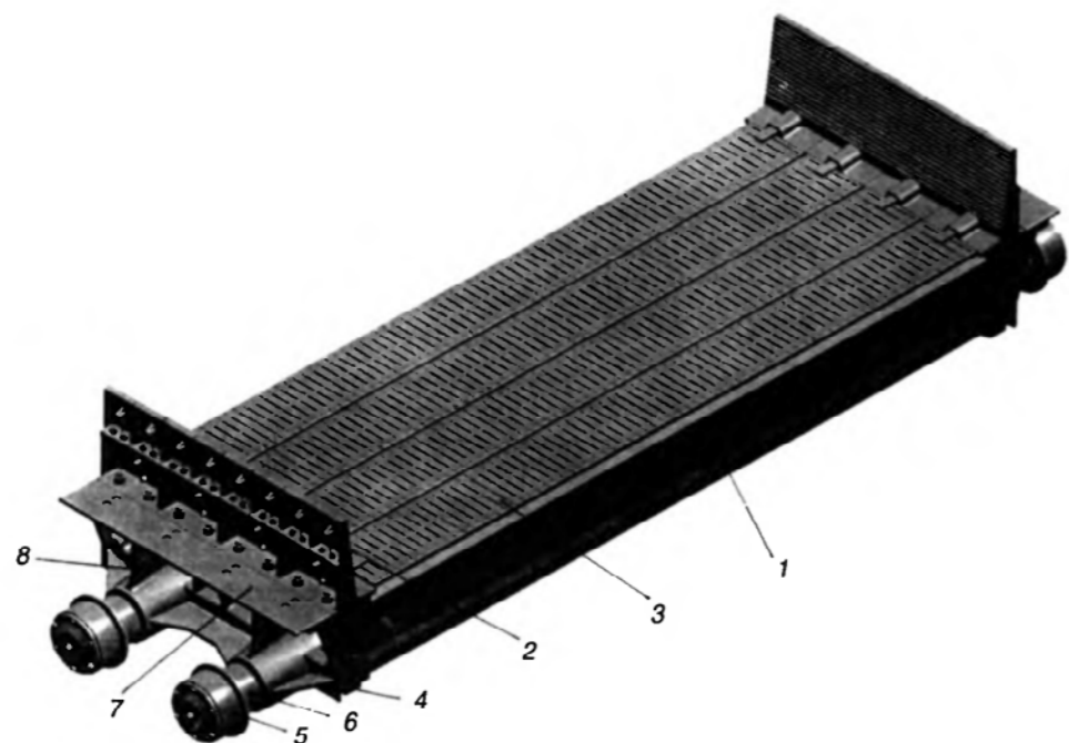
1 — нижняя несущая часть; 2 — борта; 3 — колосники; 4 — отливки боковые; 5 — ходовые ролики; 6 — грузовые ролики; 7 — пластина горизонтальная
