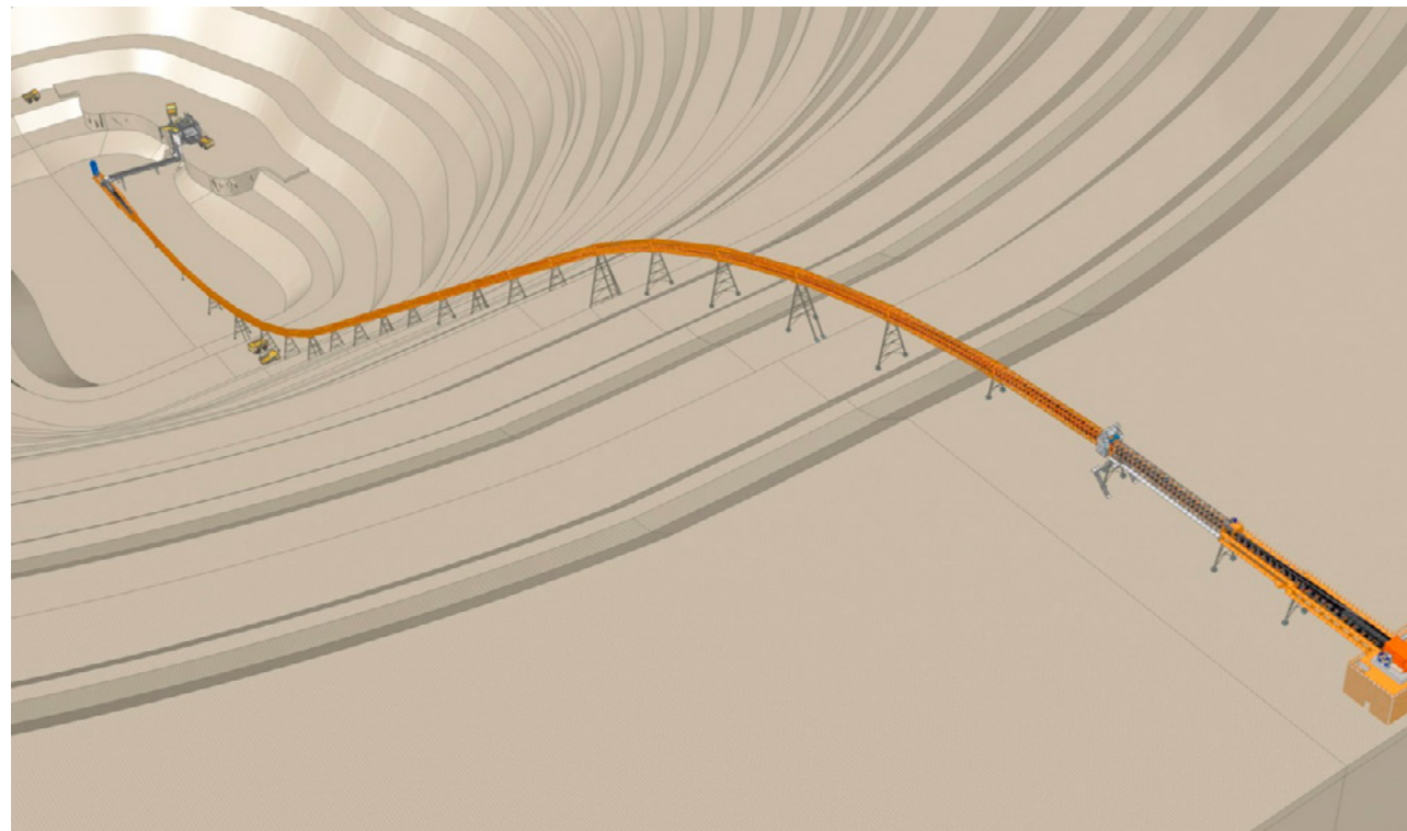
Рисунок 7.2 — Трехмерная схема крутонаклонного конвейера из карьера
