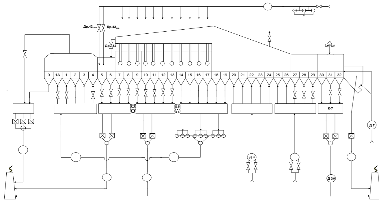
Рисунок 2.23 — Тепловая схема ОК 520
