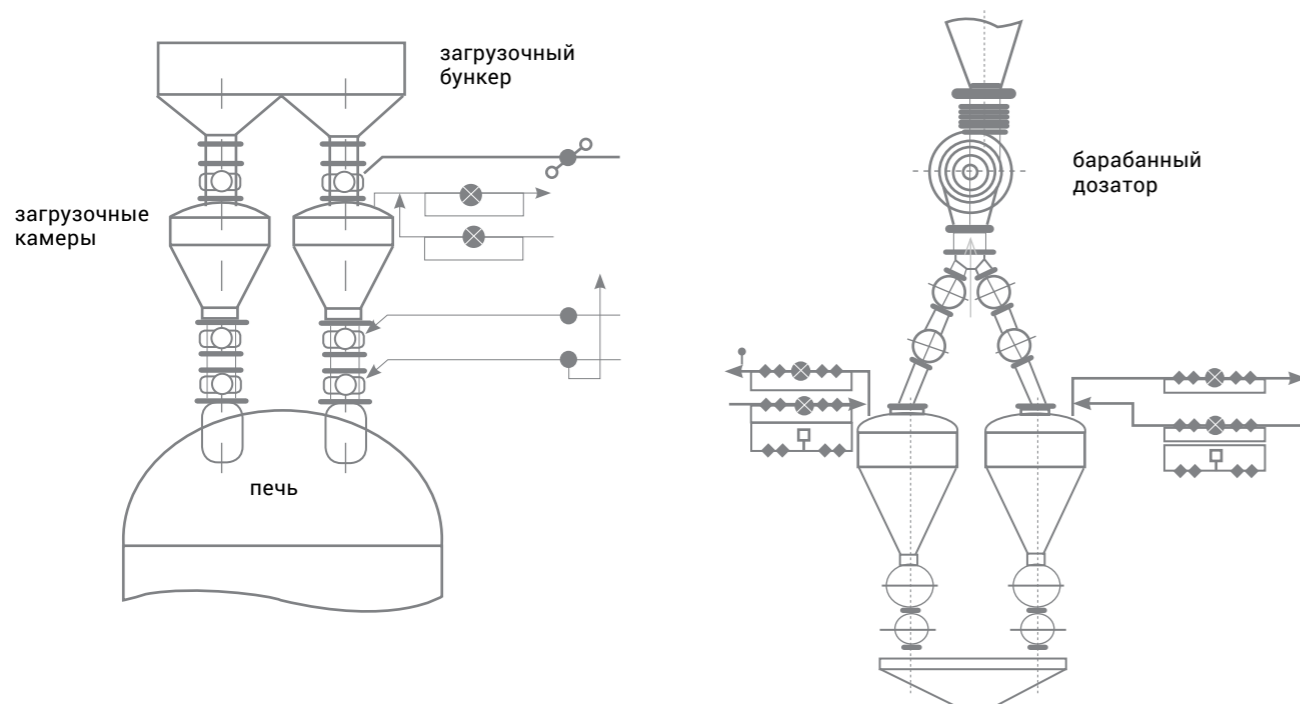
Рисунок 2.36 — Системы загрузки (а) и разгрузки (б) печи
