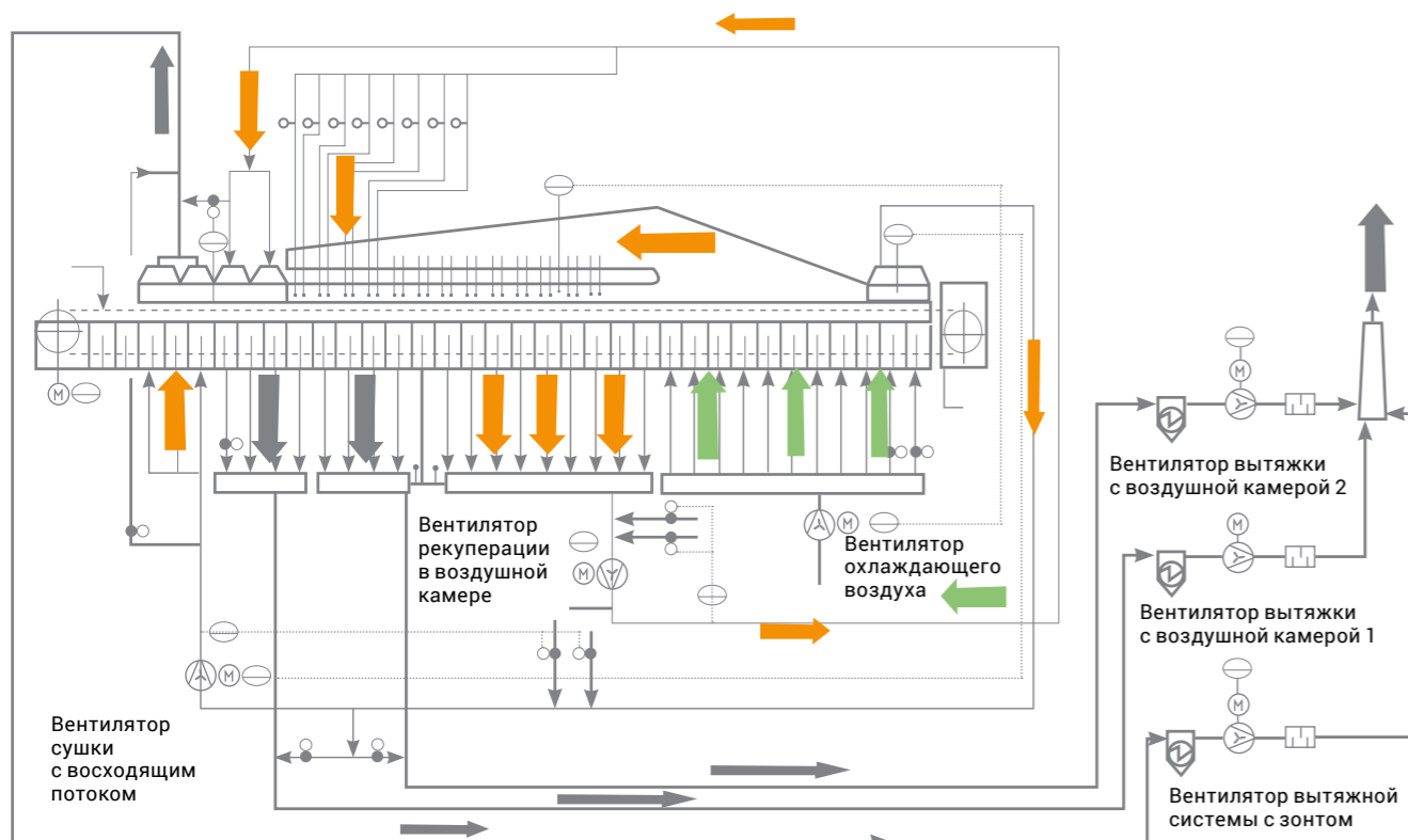
Рисунок 2.26 — Схема газовых потоков обжиговой машины O 768
