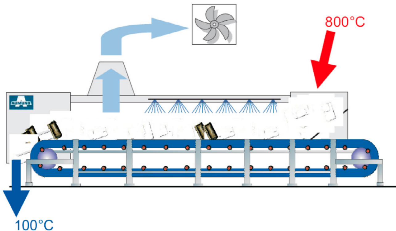
Рисунок 2.51 — Принцип действия конвейера медленного охлаждения
