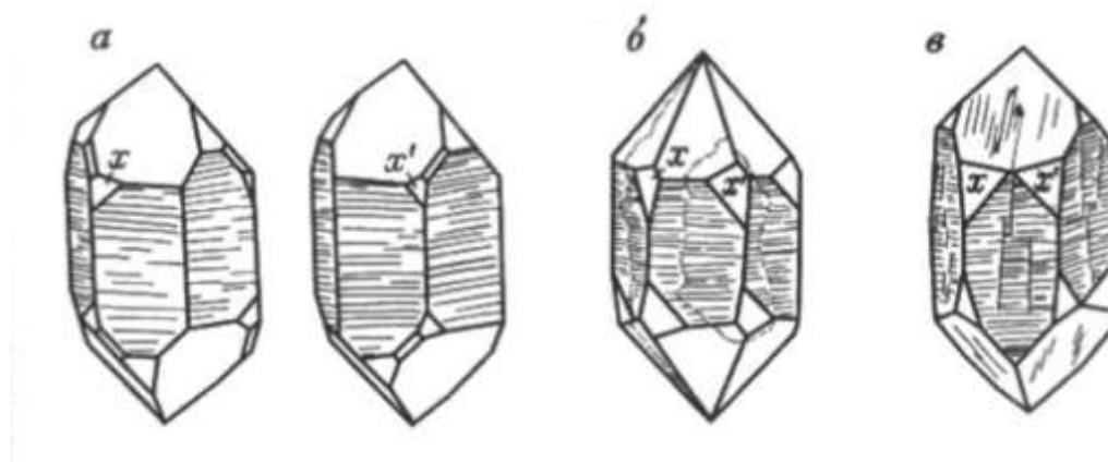
Рис. 22. Двойникование кварца: а – левый и правый кристаллы; б – дофинеиный двойник; в – бразильский двойник
