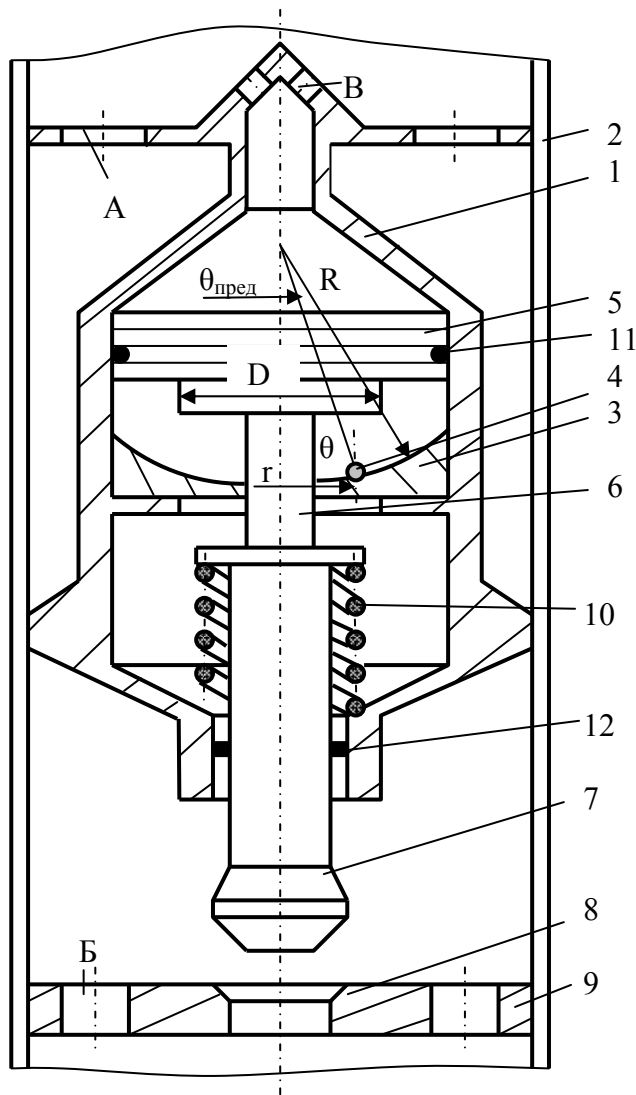
Рис.3.6. Схема сигнализатора-индикатора зенитного угла искривления ствола скважины СПЗУ-1
