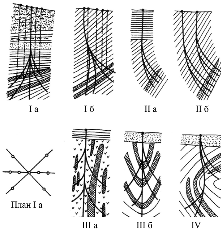
Рис.1.7.Типовые профили многоствольных скважин (по С.С.Сулакшину ):I – конусообразный; II – веерообразный; III – перистого типа; IV – комбинированного типа
