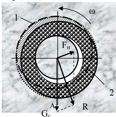
Рис.2. 52. Схема для анализа закономерностей искривления горизонтальных скважин
