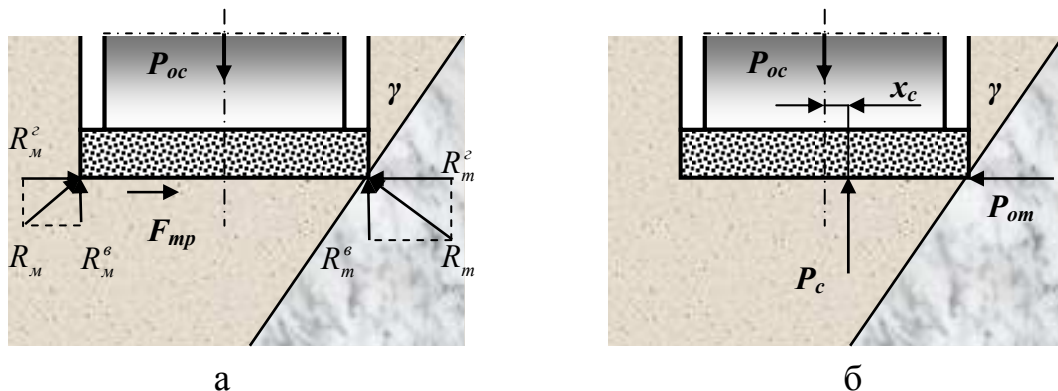
Рис.2.42. Схемы, определяющие закономерности процесса искривления ствола скважины на контакте более твердой горной породы с менее твердой.
