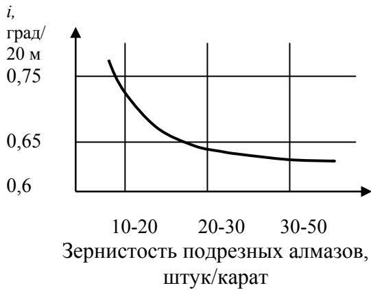
Рис.2.13. Зависимость интенсивности искривления скважин от размера подрезных алмазов (данные В.Е.Копылова)
