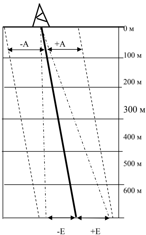
Рис.2.54. Построение «типового» профиля скважины с указанием доверительного интервала
