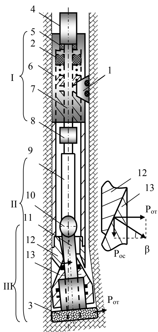
Рис.4. 59. Схема конструкции отклонителя ОКГ
