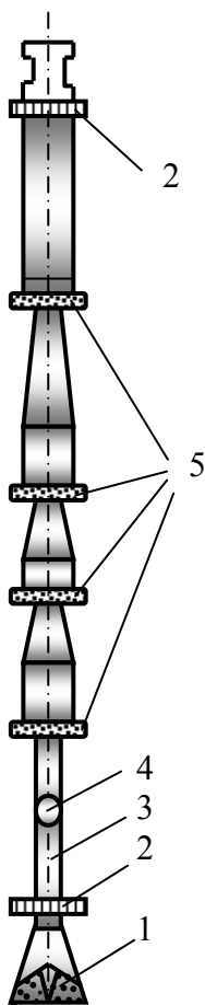
Рис.4.75 Технологический снаряд КУСТ
