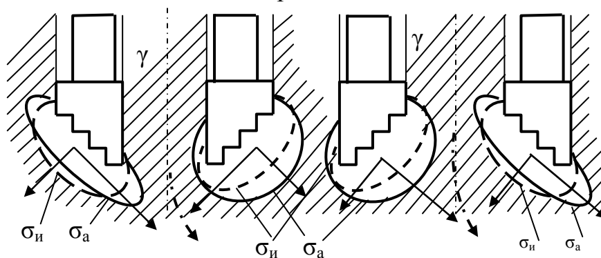
Рис.2.31. Схемы для анализа влияния профиля торца коронки на конфигурацию контура поля деформаций в анизотропной горной породе:
