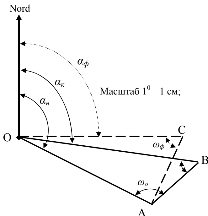
Рис. 5.24. Графо-аналитическая диаграмма для анализа результатов искусственного искривления скважины по расчетным и фактическим значениям угловых параметров
