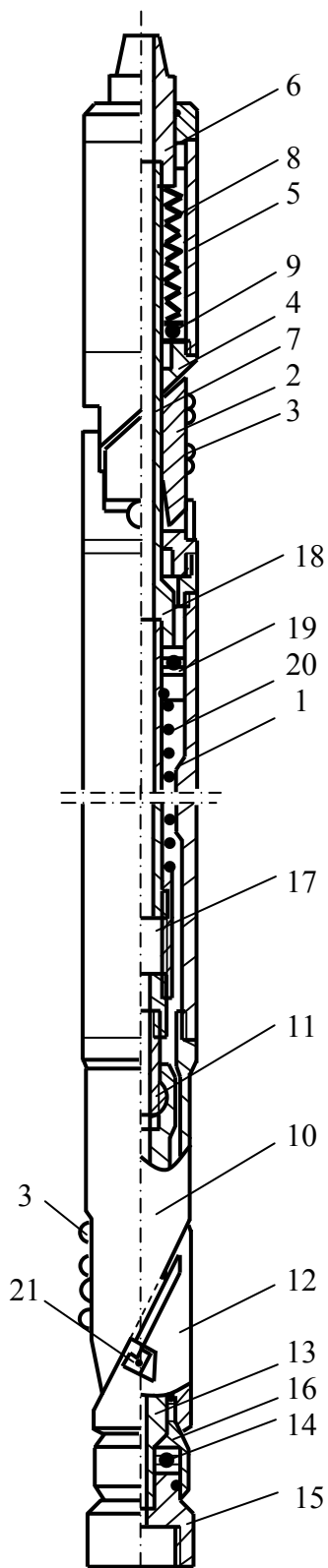
Рис.4.54. Отклонитель СБС
