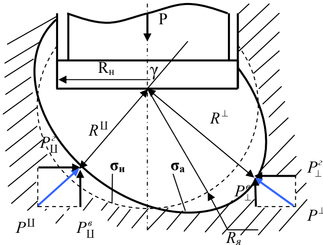
Рис.2.29. Схема для анализа деформаций и напряжений под торцом бурового инструмента
