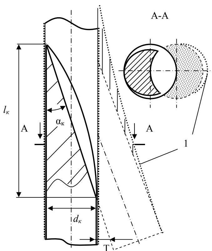
Рис.4. 28. Схема отклонения скважины от клинового отклонителя
