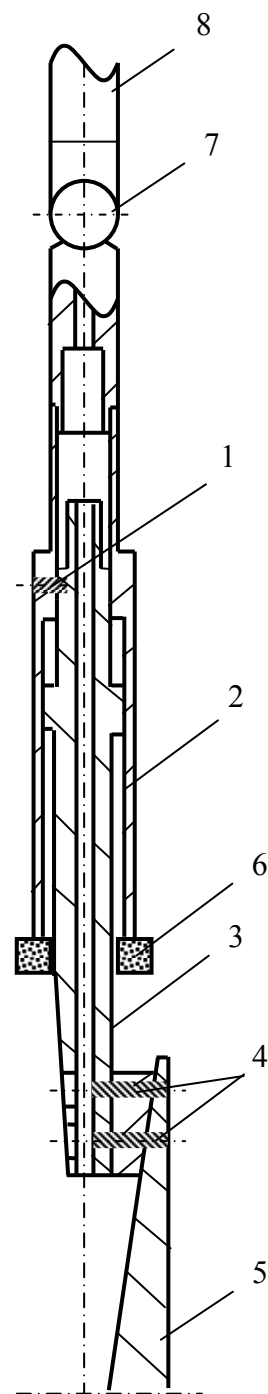
Рис.4.33. Схема клина КС с ОУ
