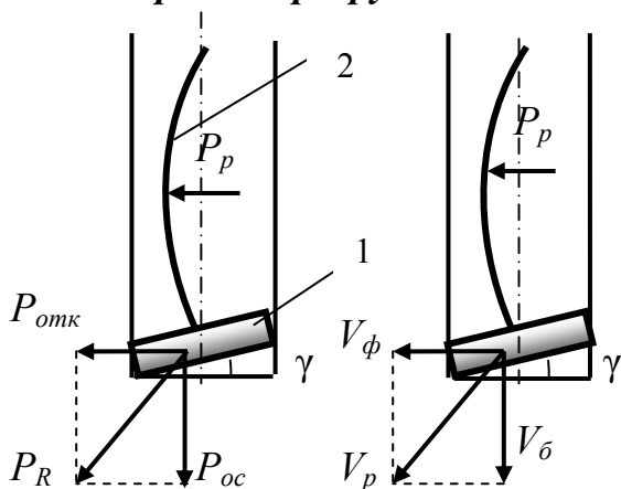
Рис.4.45. Схемы, поясняющие процесс искривления скважины при несовпадении по направлению фрезерования стенки скважины под действием отклоняющего усилия и перекоса породоразрушающего инструмента: 1- породоразрушающий инструмент; 2 – вал ОНД
