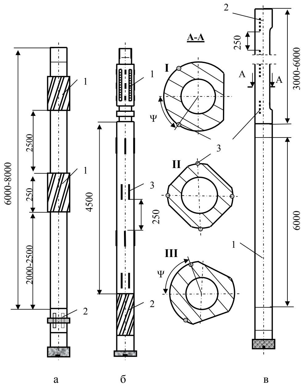
Рис.4.1. Схемы колонковых наборов для снижения интенсивности естественного искривления: а – колонковый набор с центраторами; б – компоновка ТСБИС; в- колонковый набор с четырехгранным стабилизатором или с трубами со смещенным центром тяжести поперечного сечения
