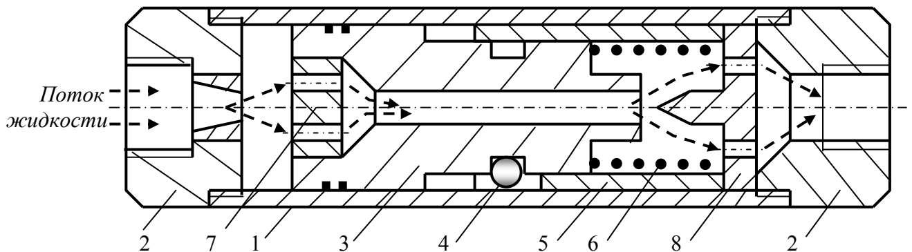
Рис.5.17. Ориентатор ОШГ
