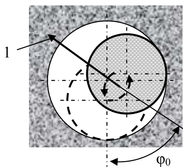
Рис.4.25. Схема для анализа направления набора кривизны шарнирной компоновкой (при накатывании её верхнего конца на стенку скважины: 1 – направление искривления скважины
