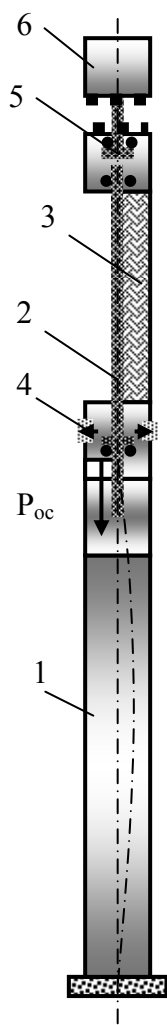
Рис.4.58. Схема колонкового снаряда с отклоняющей системой СиНУС
