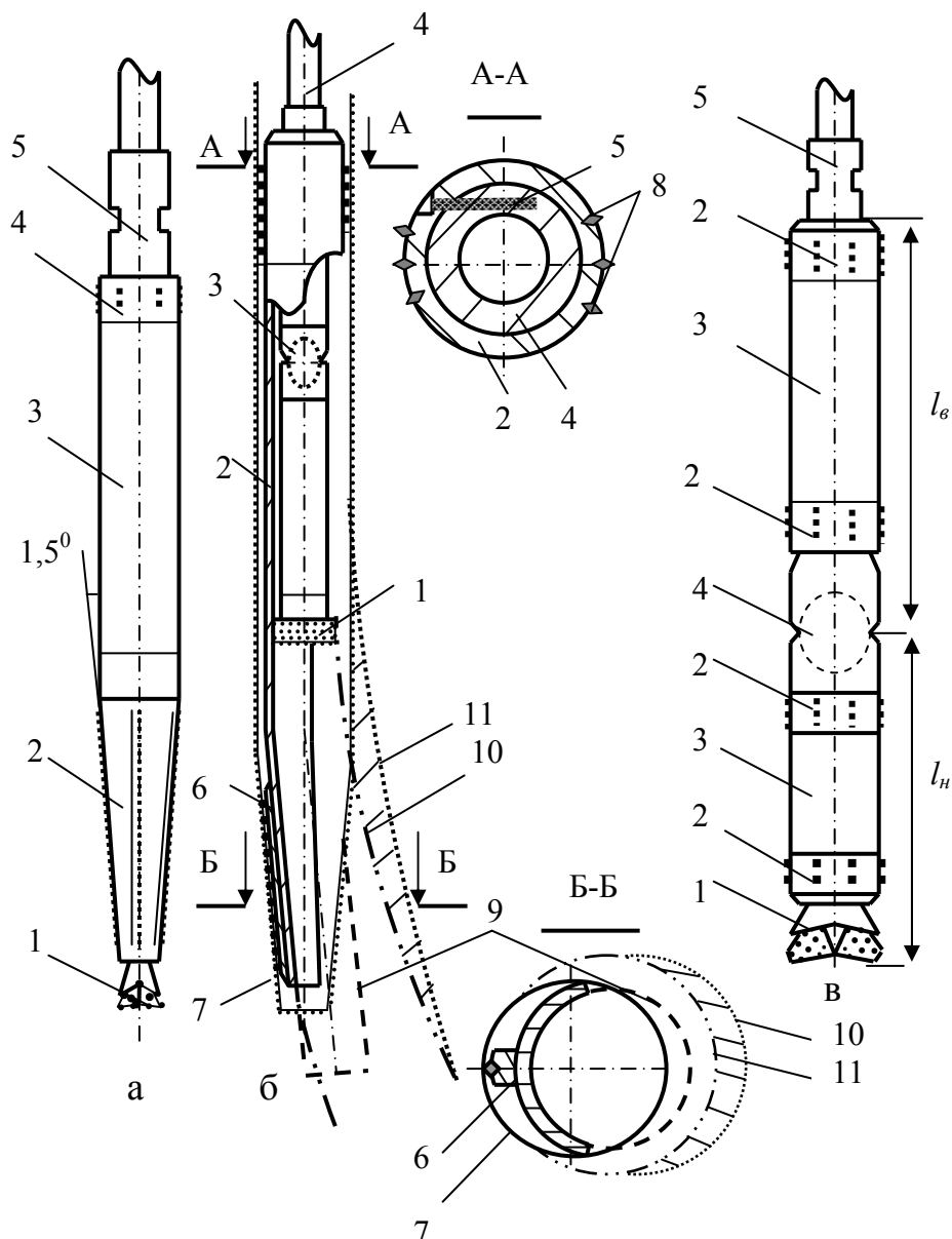
Рис.4.36. Комплект технических средств для искривления скважин клиновым отклонителем СНБ-КО а – конусный отбурник; б – отклонитель СНБ-КО в скважине; в – снаряд плавного искривления (СПИ)
