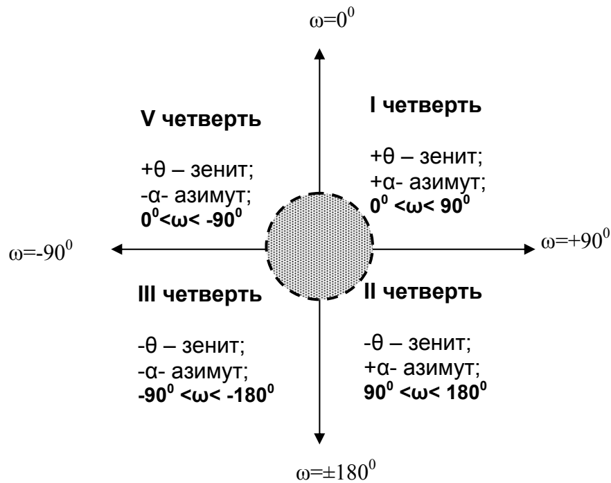
Рис.5.2. Схема отсчета углов установки отклонителя \omega_0
