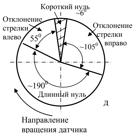
Рис.5.13. Схемы положений датчика ориентатора УШО и соответствующие этим положениям показания наземного миллиамперметра (а-г) и диаграмма, отражающая диапазоны углов поворота ориентатора вокруг своей продольной оси, соответствующие означенным положениям датчика и стрелки миллиамперметра (д)
