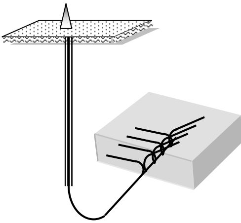
Рис.8.4. Схема радиально-горизонтальной скважины с системой восстающих стволов
