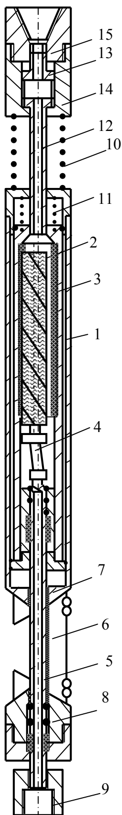
Рис.4. 62. Схема отклонителя на базе ВЗД Д1-54 ДН-54
