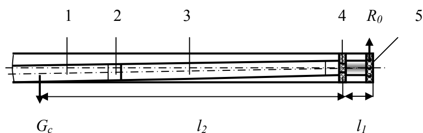
Рис. 4.9. Схема компоновки для бурения горизонтальных скважин: 1 – утяжеленная буровая труба; 2 - переходник; 3 - колонковая труба; 4 - расширитель (опорно-центрирующий элемент); 5 – коронка
