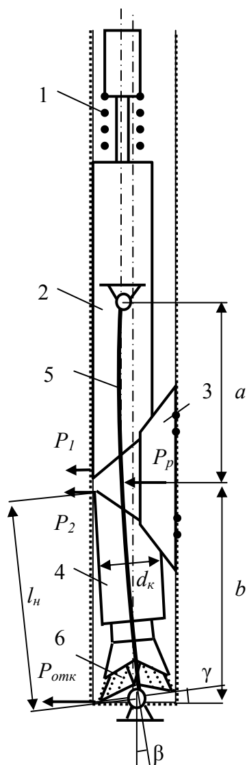
Рис.4.53. Расчетная схема ТЗ-3 в прямолинейном стволе скважины
