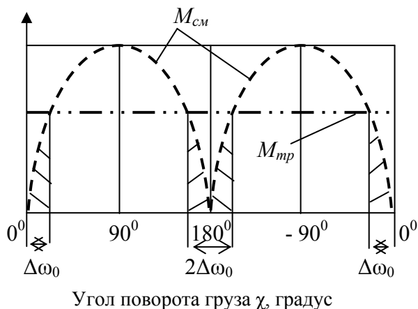
Рис.5.9. Графики M_{см} и M_{тр} от угла смещения эксцентричного груза \chi
