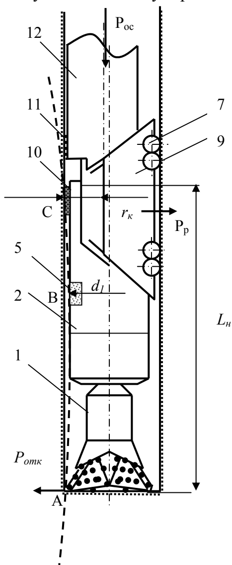
Рис.4.49. Схема отклонителя ТЗ-3П-59 в рабочем положении
