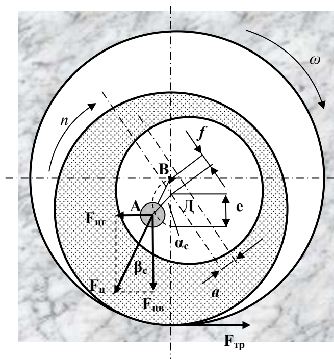
Рис. 4.3. Схемы для анализа работы компоновки со смещенным центром тяжести поперечного сечения
