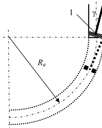
Рис.4.24. Схема набора кривизны шарнирной компоновкой (1), находящейся в состоянии фиксированного перекоса в скважине
