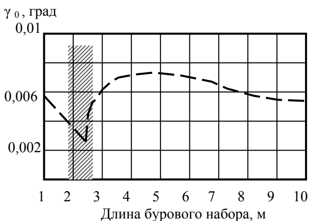
Рис.2.6. Зависимость угла перекоса бурового набора от его длины
