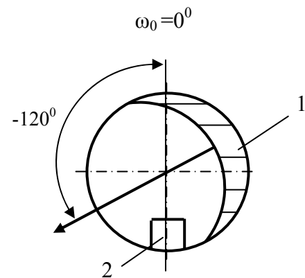
Рис.5.5. Схема установки клина относительно пяты ориентатора ШОК под углом установки 120^\circ
