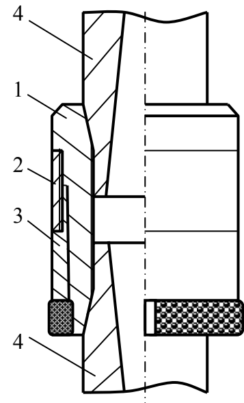
Рис.4.76. Фрезер-расширитель технологического набора: 1 – корпус; 2 – втулка; 3 – алмазная коронка; 4 – труба
