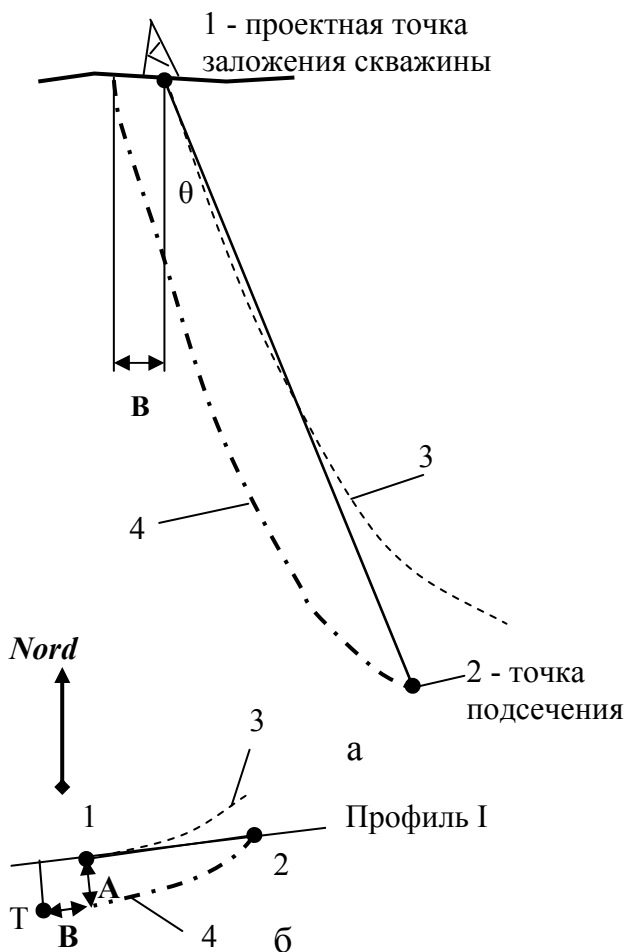
Рис. 2.55. Схема для определения точки заложения скважины на профиле по «типovým» кривым: 1 – проектная точка заложения скважины на профиле I; 2 – проектная точка подсеечения рудного тела на глубине; 3 – линия естественного искривления скважины; 4 – «типové» кривые зенитного (а) и азимутального искривления (б)
