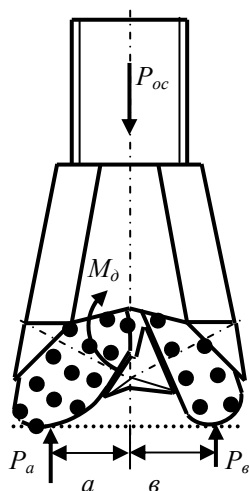
Рис.2.17. Схема сил при бурении асимметричным долотом ДДА
