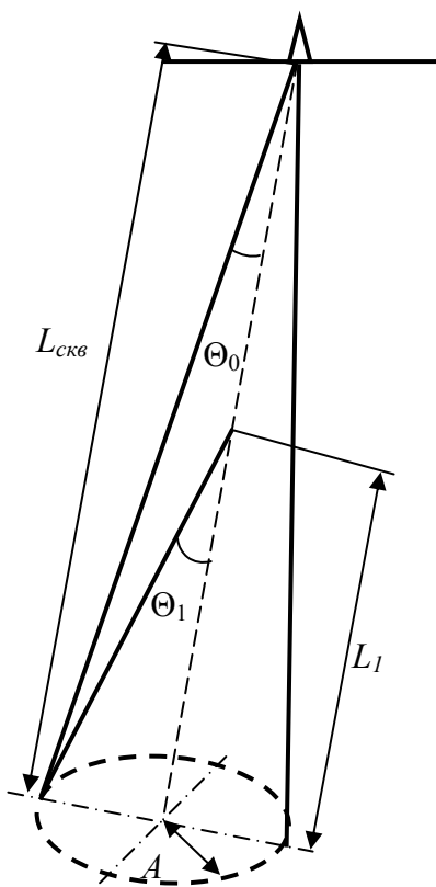
Рис.6.1. Схема для расчета варианта допустимых отклонений забоя скважины
