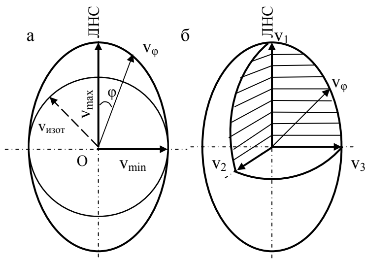
Рис.2.25 . Диаграммы анизотропии горных пород по скорости бурения : а- в зависимости от угла \phi между направлением вектора скорости v_\phi и ЛНС; б- эллипсоид анизотропии по буримости - v_1 = v_{max}
