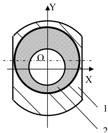
Рис.4.14.Схема эксцентричной установки ЭУБТ в буровой компоновке
