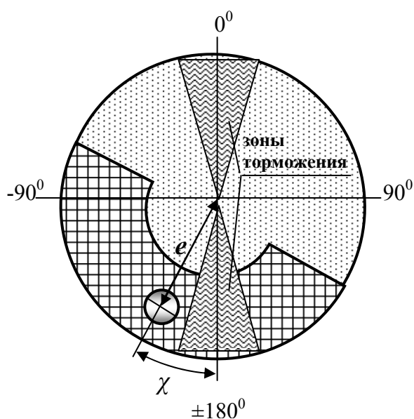
Рис.5. 8 . Схема к определению M_{см} самоориентатора
