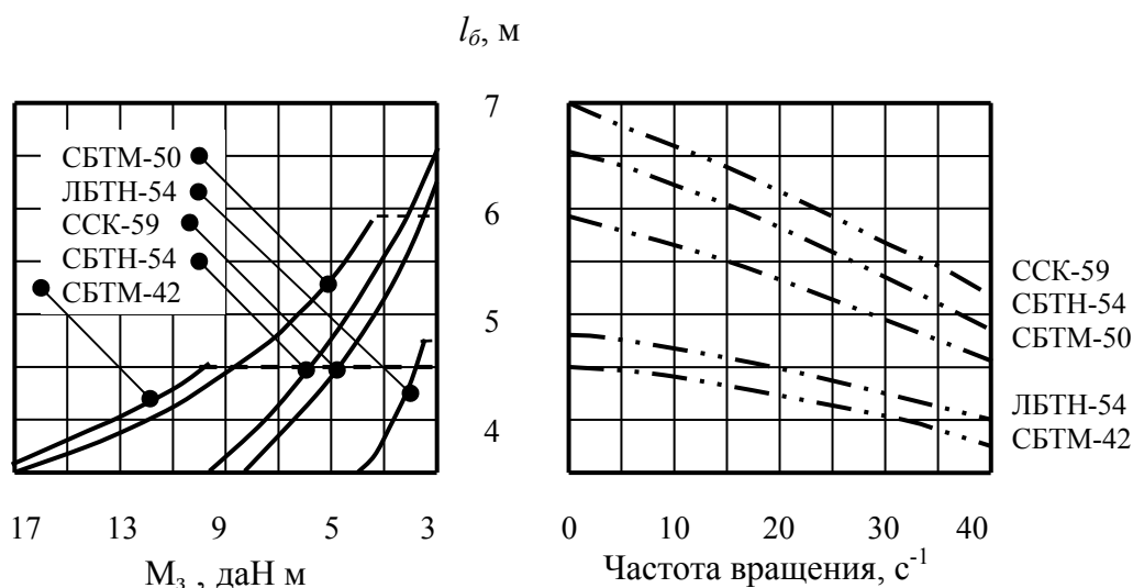
Рис. 2.5. Номограмма для определения величины изгибающего момента M_3 в зависимости от частоты вращения и длины полуволны l_\delta колонны при бурении скважин диаметром 59 мм различными бурильными колоннами при P_{oc} = 20 кН
