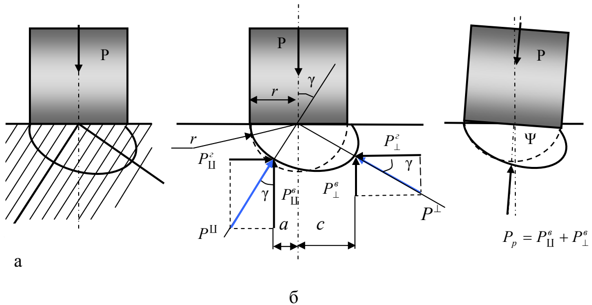
Рис.2.26. Схема для анализа процесса деформирования анизотропной породы плоским цилиндрическим индентором и определения упругих реакций со стороны деформируемой породы: а – формирование эллипсоидного ядра сжатия под торцом индентора; б - схема реакций породы на внедряемый индентор через ядро сжатия породы; в – схема поворота индентора при внедрении в анизотропную породу
