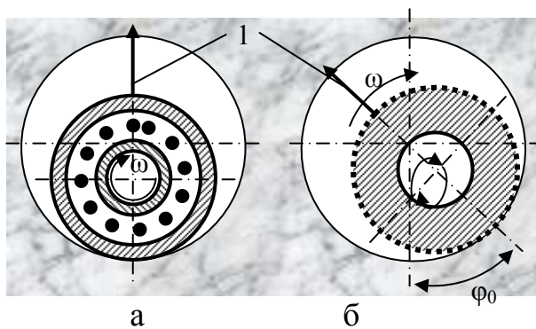
Рис.4. 26. Схемы шарнирных компоновок с уменьшенным (а) и увеличенным эффектом накатывания (б) на стенку скважины: 1 – направление искривления скважины
