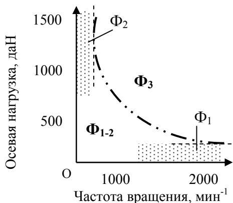
Рис.2.12. Области существования видов движения деформированных бурильных колонн и компоновок
