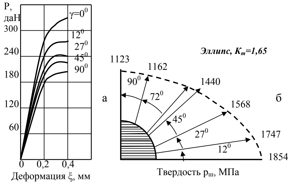
Рис.2. 23. Диаграмма деформирования (а) и полярная диаграмма твердости туфо-дацита (б) в плоскости перпендикулярной слойкам
