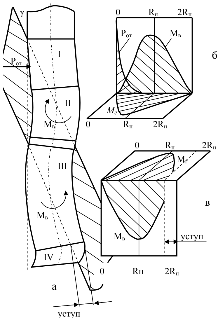
Рис.2.46. Схема формирования ствола (а) и соответствующие графики силовых величин, воздействующие на инструмент, при входе (б) и выходе (в) при пересечении пропластка твердой горной породы
