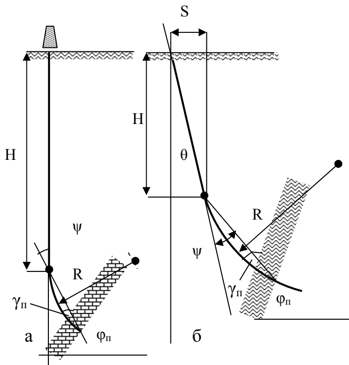
Рис.5.37. Схемы к расчету траекторий скважин
