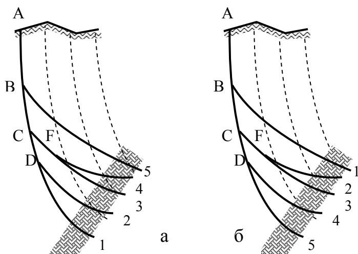
Рис.5.28. Схемы построения одной многоствольной скважины взамен четырех одноствольных: а – по методике «снизу-вверх» - основной ствол – АВ, дополнительные по порядку бурения – В1, D2, C3, F4, В5; б – по методике «сверху-вниз» - основной ствол – АВ, дополнительные по порядку бурения- В1,В2,С3,С4, D5.
