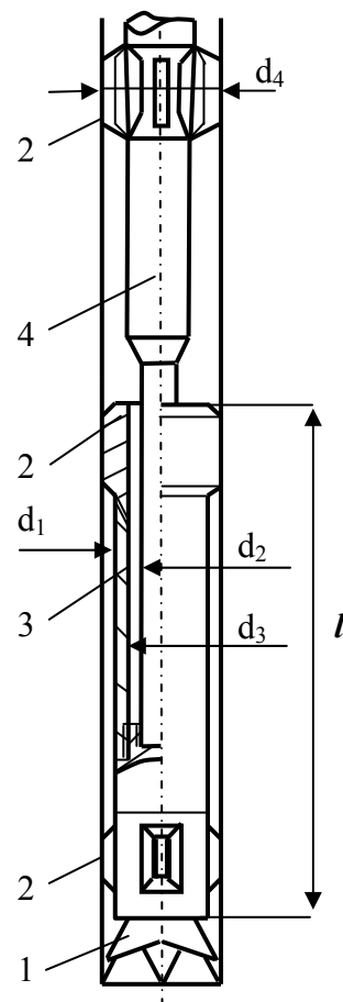
Рис.4.12. Схема компоновки НСУ: 1 – долото; 2 – центратор; 3 – кожух; 4 – УБТ
