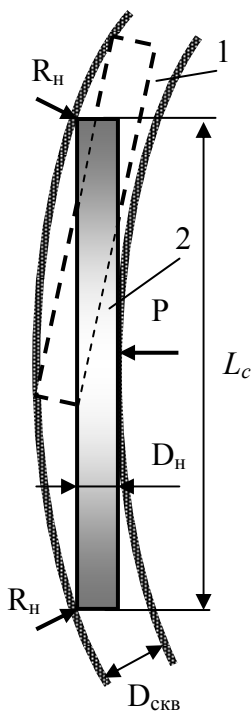
Рис.5.25. Схема для анализа условий вписываемости снаряда в искривленный ствол скважины
