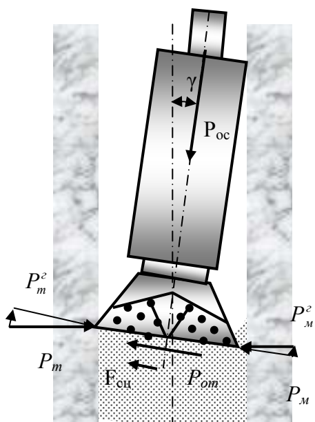
Рис.5.31. Схема для определения условий образования уступа в стенке скважины ОНД
