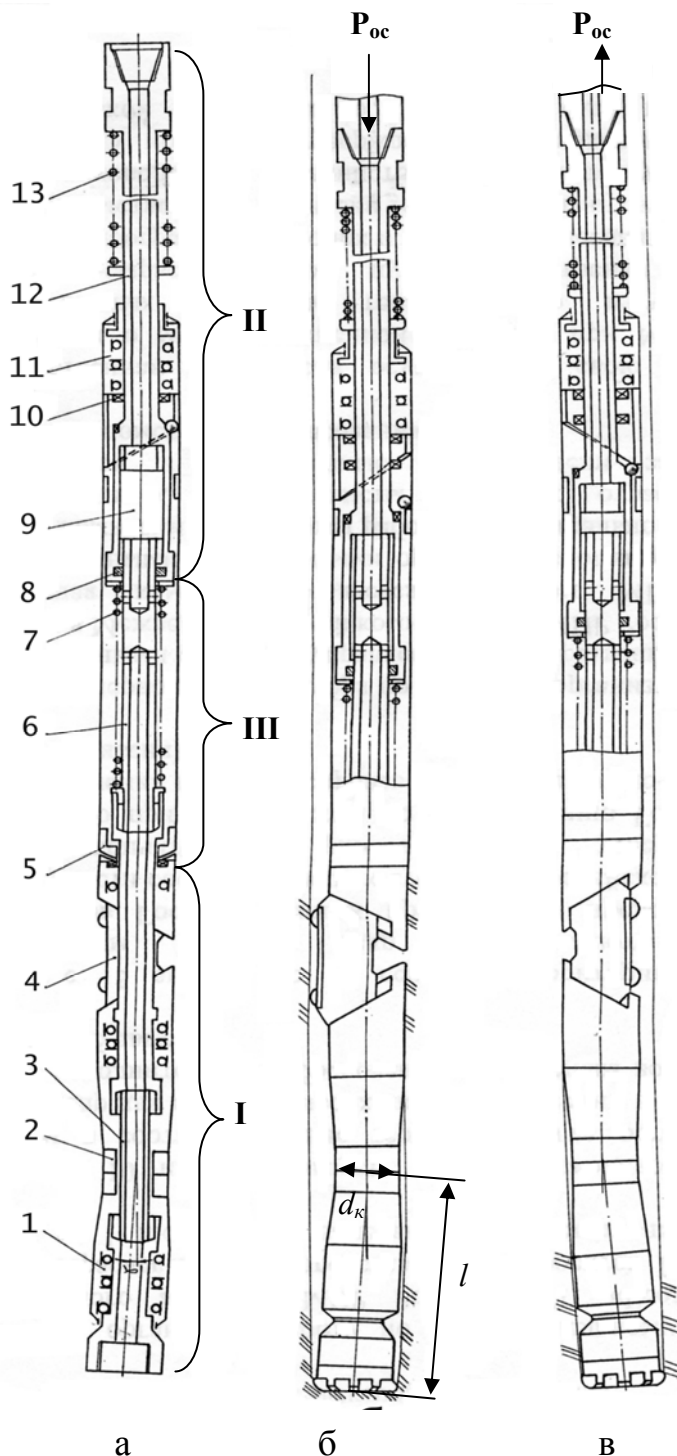
Рис.4.47. Отклонитель «КЕДР»: а - транспортное положение; б – постановка отклонителя на забой и создание осевой нагрузки (рабочее положение); в – ориентирование (отрыв отклонителя от забоя)
