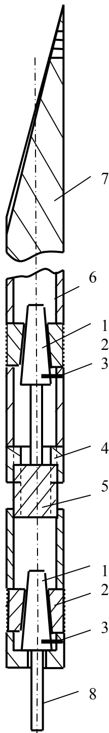
Рис.4.35. Схема распорного механизма стационарного клина
