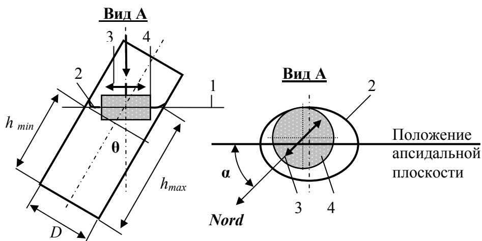
Рис.3.2. Схема определения зенитного \theta и азимутального \alpha углов скважины в приборе Мааса: 1 –горизонтальная линия; 2 – уровень застывшего желатина; 3 – магнитная стрелка; 4 – поплавок из пробкового дерева
