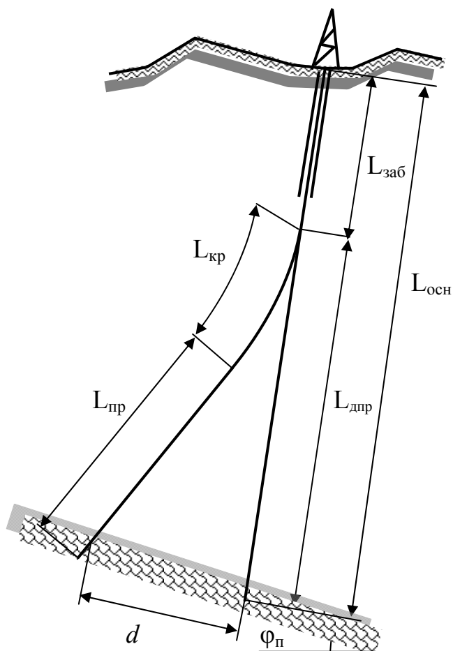
Рис. 5. 39. Схема для расчета параметров дополнительного ствола
