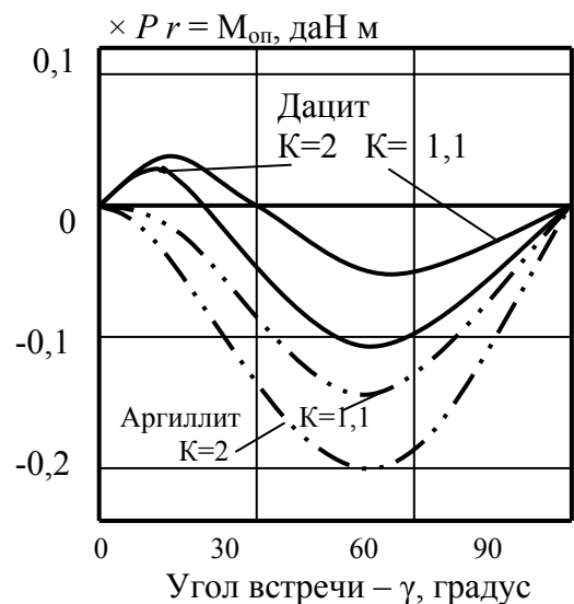
Рис.2.27. Графики M_{on} в зависимости от угла встречи \gamma для осадочной (аргиллит) и эффузивной (дацит) горных пород
