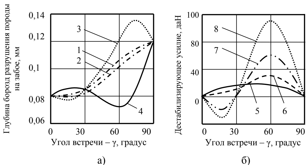
Рис.2. 33. Зависимости глубин борозд разрушения анизотропной породы (а) и дестабилизирующего усилия \Delta F от угла встречи: 1,2 - глубина борозд при v_{\phi}/v_{\delta} = 0,0001 при перемещении реза в направлении и навстречу слоистости соответственно; 3,4 - тоже при v_{\phi}/v_{\delta} = 1 ; 5 - \Delta F при v_{\phi}/v_{\delta} = 0,0005 ; 6 - \Delta F при v_{\phi}/v_{\delta} = 0,005 ; 7 - \Delta F при v_{\phi}/v_{\delta} = 0,05 ; 8 - \Delta F при v_{\phi}/v_{\delta} = 0,1
