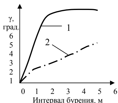
Рис.4.38. Результаты набора кривизны различными компоновками с СНБ-КО
