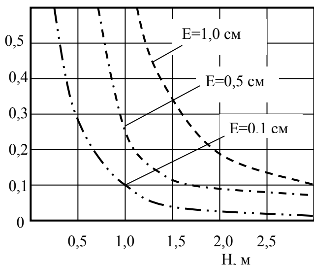
Рис.4.78. Зависимость интенсивности искривления при внецентренном приложении ударов к инструменту от расстояния H и эксцентриситета приложения ударов E
