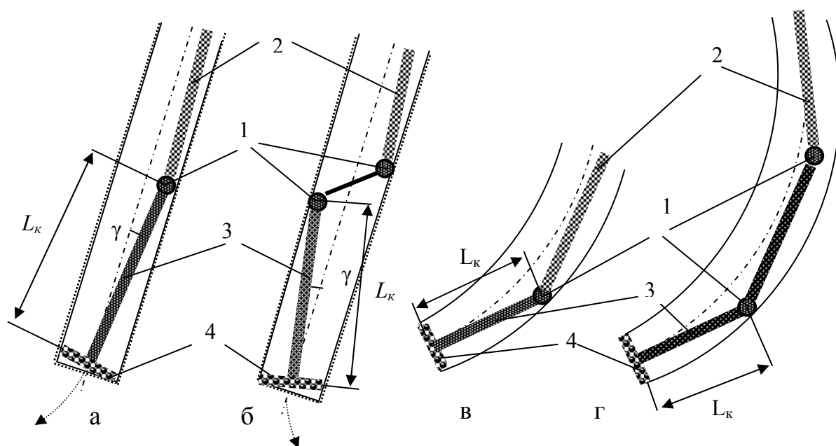
Рис.4.22. Схемы работы шарнирных компоновок в прямолинейном наклонном и криволинейном стволе скважины.
