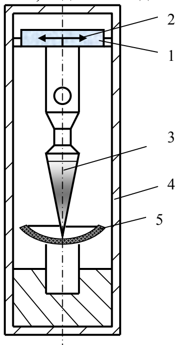
Рис. 3.3. Схема устройства инклинометра МИ-42У
