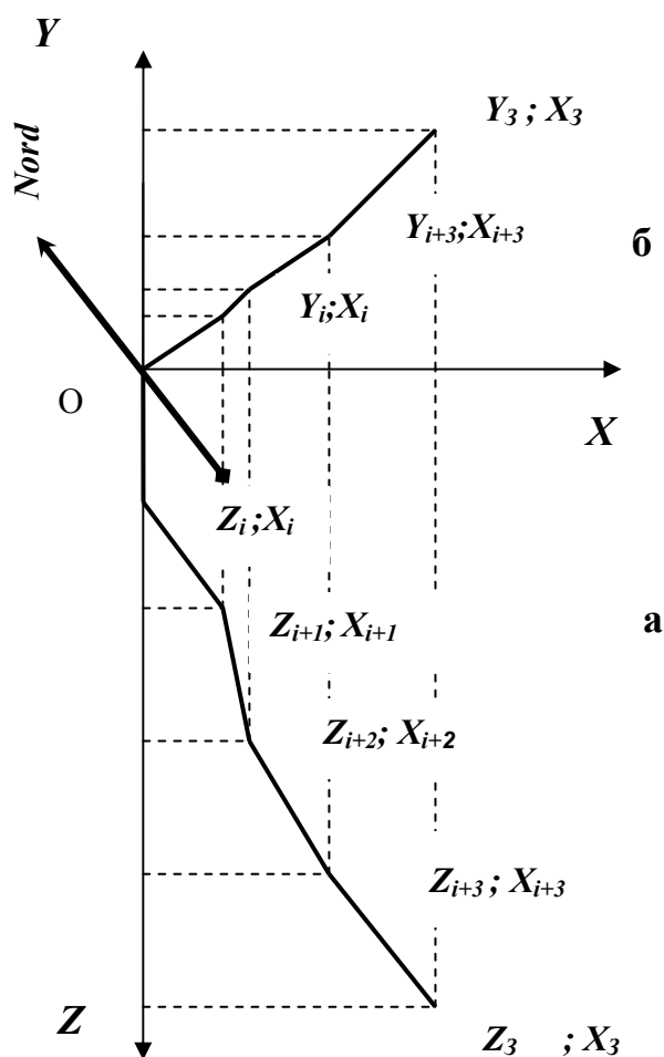
Рис. 1.3 Профиль и инклинограмма (план) скважины
