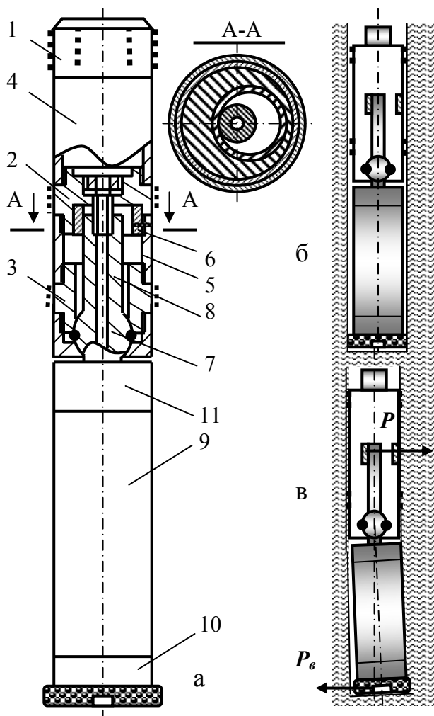
Рис.4.17. Компоновка «Стабит»: а – схема конструкции снаряда; б – положение компоновки в прямолинейном стволе; в – положение снаряда в искривленном стволе
