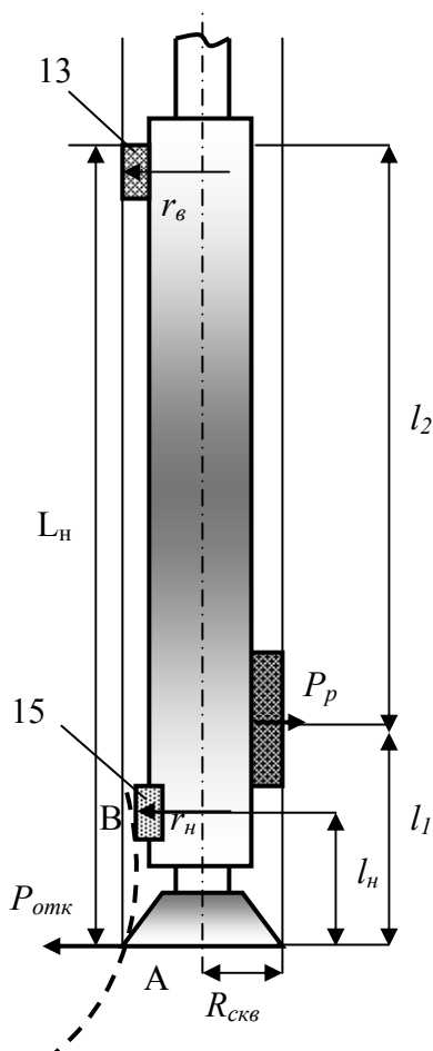
Рис.4.52. Схема параметров отклонителя ОГМ
