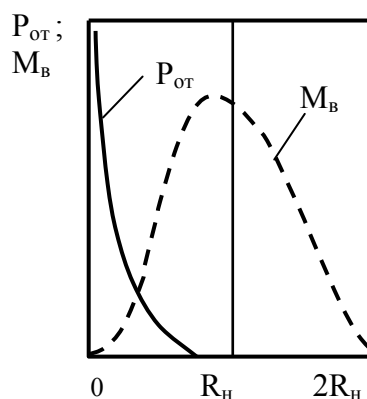
Рис.2.43. Графические зависимости P_{от} и M_e на интервале пересечения контакта буровым инструментом с торцом радиусом R_n
