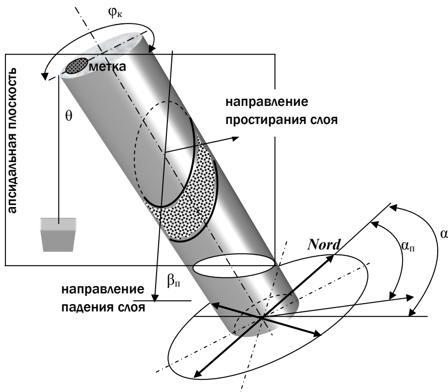
Рис.7.10. Схема ориентирования керна по метке и определение элементов залегания горных пород по ориентированному керну
