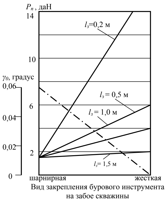
Рис.2. 8. Зависимости усилия P_n и угла перегиба \gamma_0 от условий закрепления нижнего конца буровой компоновки
