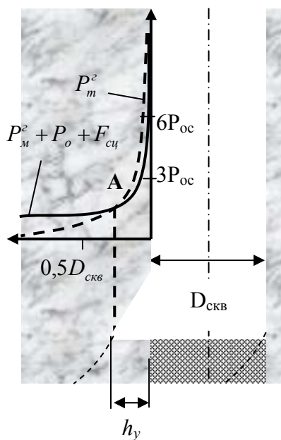
Рис.5.32. Графическое решение уравнения равновесия сил при забурировании, определяющее ширину уступа h_y
