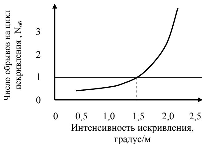
Рис.5.22. Зависимость числа обрывов бурильной колонны от величины интенсивности искривления
