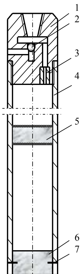
Рис.5.29. Контейнер для доставки твердеющей смеси в скважину
