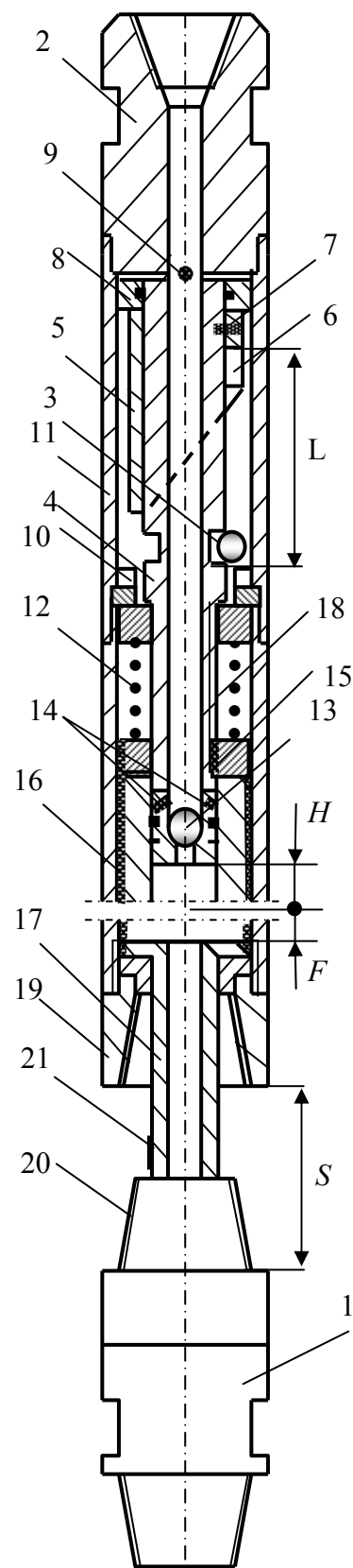
Рис.5. 20 . Схема конструкции ориентатора АЗОР
