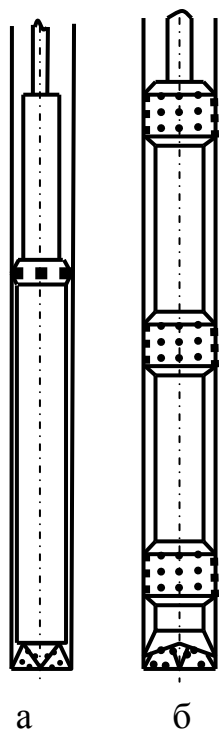
Рис.4.11. Схемы «маятниковой» и жесткой буровых компоновок
