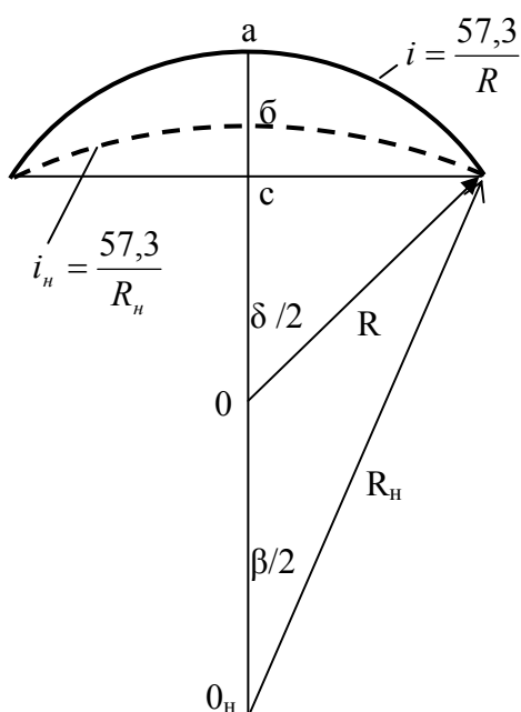
Рис.4. 72 . Схема для расчета толщины снимаемого слоя породы для преобразования кривизны стенки скважины после искривления i в кривизну после проработки интервала искривления i_n
