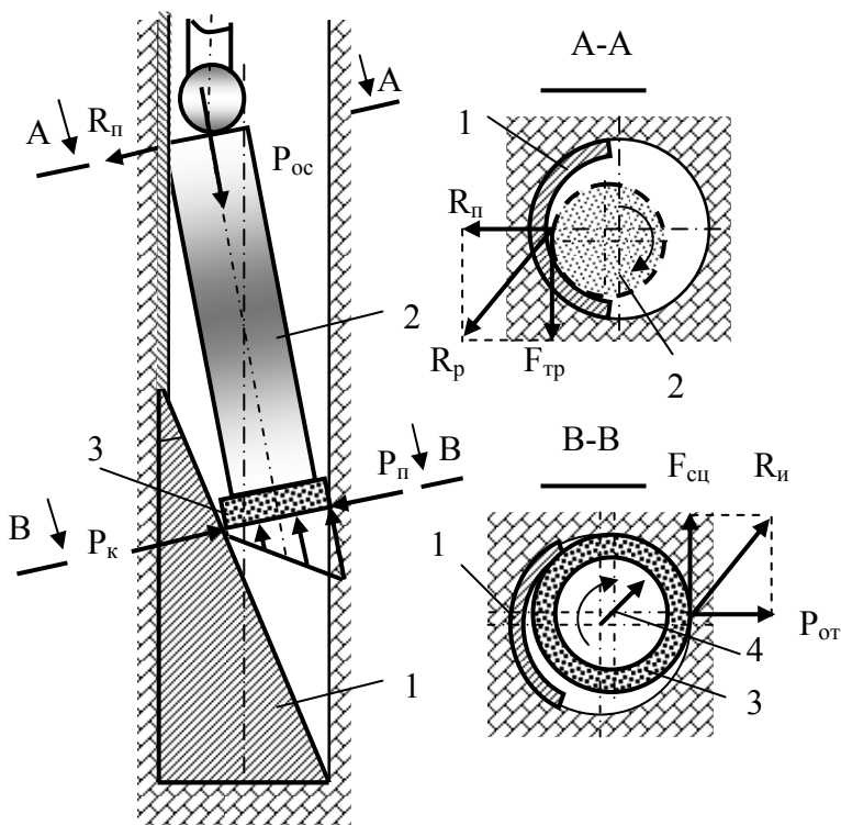
Рис. 4.66. Схема сил при забурировании пилот-скважины с использованием клинового отклонителя: 1 – ложка клина; 2 – отбурочный набор; 3 – коронка; 4 – направление забуривания
