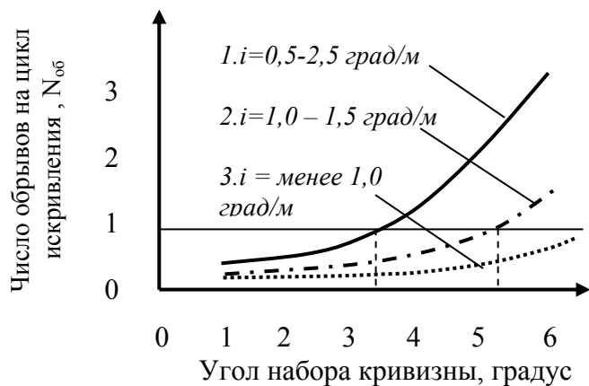
Рис.5.21. Зависимость числа обрывов бурильной колонны от величины угла набора кривизны при различных значениях интенсивности искривления
