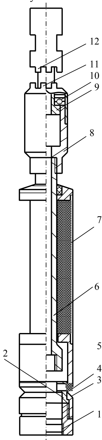
Рис.5. 6. Ориентатор ОП
