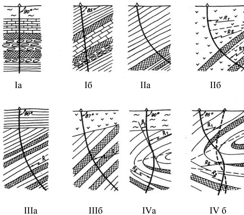
Рис.1.6. Типовые профили одноствольных скважин: (по С.С.Сулакшину). I – прямолинейный; II – искривленный; III – комбинированный; IV- сложноискривлённый
