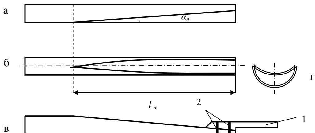
Рис.4.29. Схемы, поясняющие процесс изготовления стационарного клина: а,б - разметка линия отреза, при изготовлении ложка; в - схема клина с установочным патрубком 1 и срезными штифтами 2; г – поперечное сечение ложка клина
