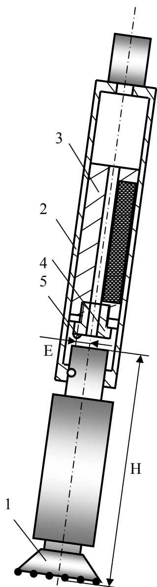
Рис.4.77. Схема отклонителя на базе забойного ударного механизма
