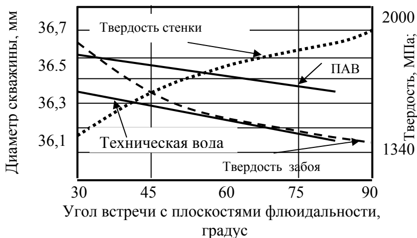
Рис. 2.40. Зависимости диаметров скважины от угла встречи с плоскостями флюиальности туфо-дацита при бурении водой с ПАВ и технической водой
