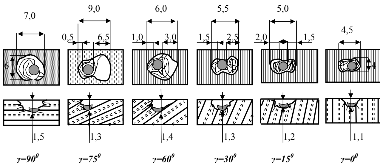
Рис. 2.28. Формы лунок разрушения в анизотропных горных породах при различных углах встречи \gamma плоскости сланцеватости
