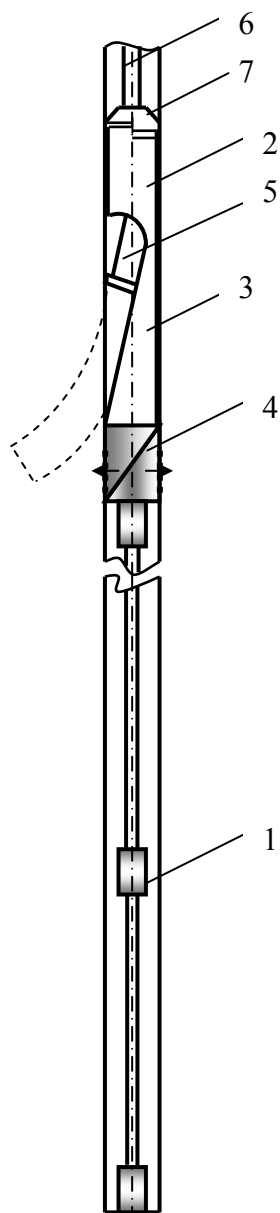
Рис.4.41. Схема бурения дополнительного ствола клином КПП
