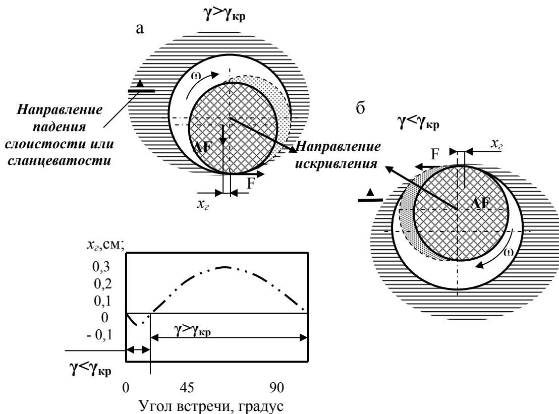
Рис. 2.50. Схемы для анализа механизма азимутального искривления при бурении анизотропной породы при углах встречи больше критического (а) и меньше критического (б) и график изменения расстояния x_2 в зависимости от угла встречи
