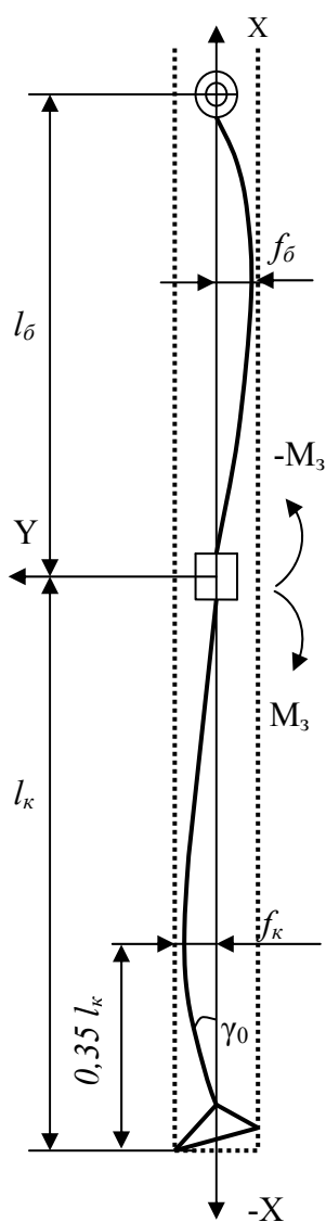
Рис.2.4. Схема для анализа работы буровой компоновки
