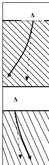
Рис. 2. 49. Зависимость интенсивности искривления скважин в анизотропных породах от угла встречи со слоистостью, сланцеватостью
