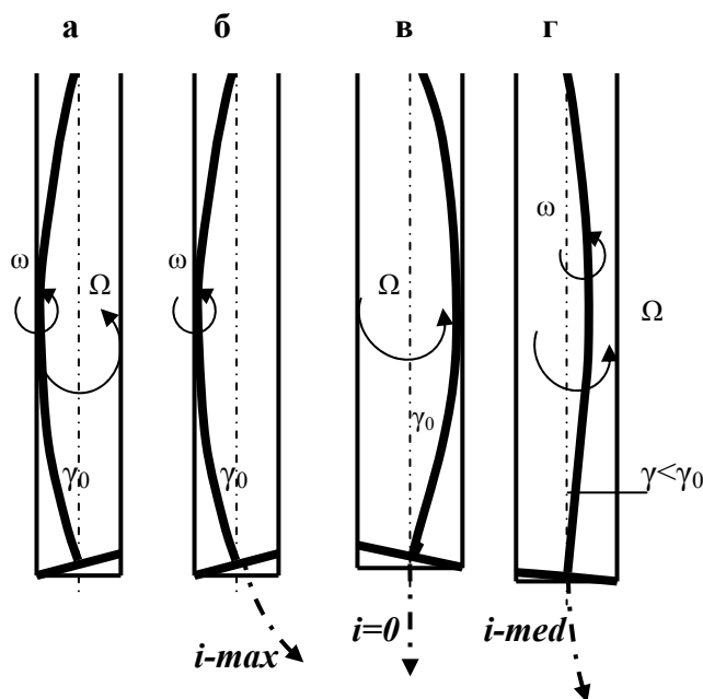
Рис.2.10. Схемы к анализу влияния вида движения деформированной компоновки на интенсивность естественного искривления скважин
