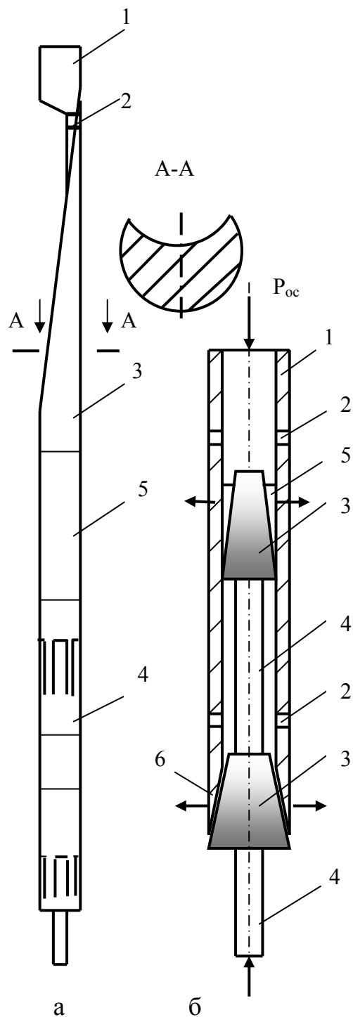
Рис.4.31. Схемы компоновки стационарного клина КОС (а) и распорного механизма клина КОС (б)
