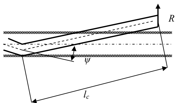
Рис. 5.26. Деформация компоновки с угловой несоосностью \psi в прямолинейном стволе скважины
