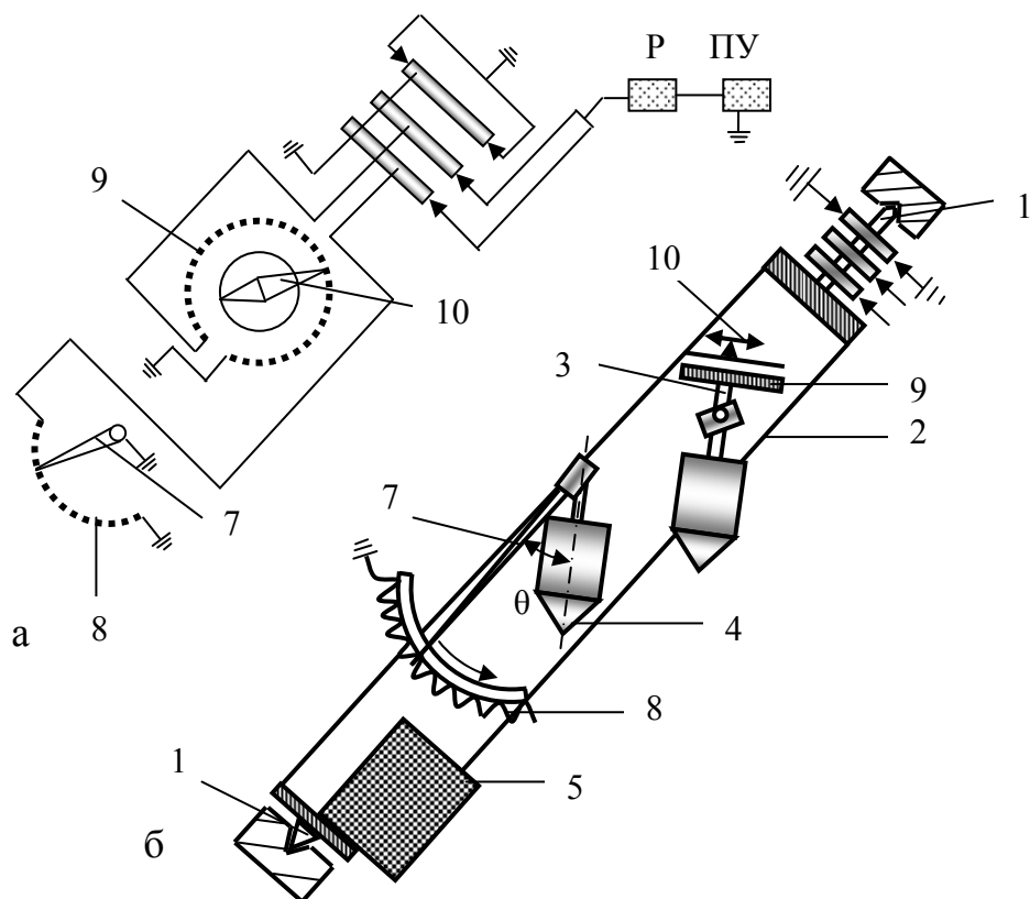
Рис.3. 4 . Электрическая (а) и механическая (б) схемы инклинометра типа ИШ
