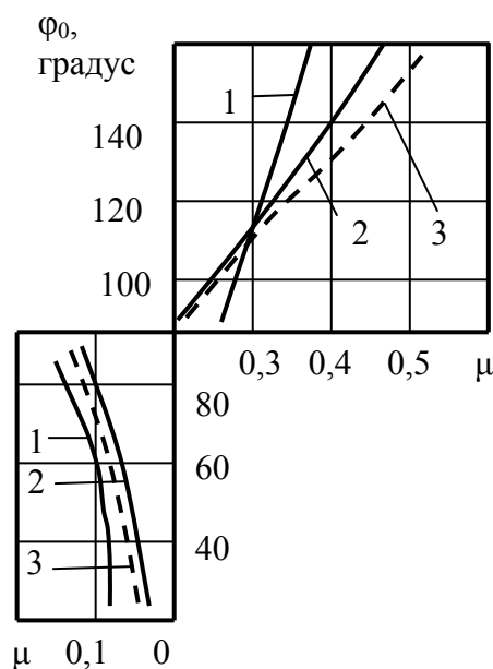
Рис.2.21. Расчетные значения угла накатывания компоновки с пневмоударником в зависимости от коэффициента трения на контакте забойной машины и колонны бурильных труб со стенкой скважины 1 – СБТМ-50 ( P_{oc}=800 даН); 2 – СБТМ-50 ( P_{oc}=400 даН); 3 – ЛБТН-54 ( P_{oc}=400 даН)
