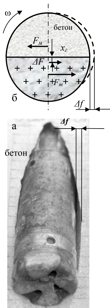
Рис.2.45. Фото бурового инструмента в скважине (а) на интервале пересечения контакта различной твердости (пластина гранита в бетоне) и схема распределения усилий на резцах усилий при разрушивании контакта пород различной твердости (б)
