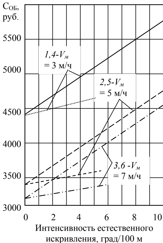
Рис.6.2. Зависимость стоимости метра бурения от интенсивности естественного искривления при различных значениях механической скорости бурения при устранении отклонения скважины только отклонителями: линии 1,2,3 и с применением методики проектирования трасс скважин с учетом закономерностей естественного искривления при достоверности «типовой» кривой 80%: линии 4,5,6
