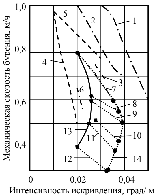
Рис.4.2. Производственные данные (Кривой Рог), отражающие связь интенсивности искривления и механической скорости бурения
