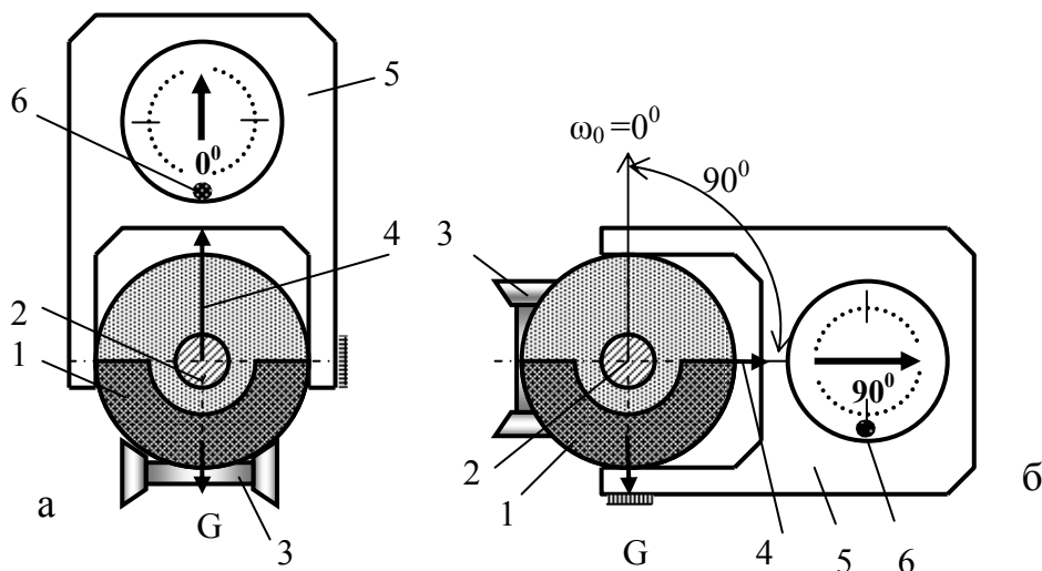
Рис.5.7. Схемы, поясняющие процесс настройки самоориентатора ОП и отклонителя типа ТЗ на угол установки отклонителя \omega_0 = 90^\circ
