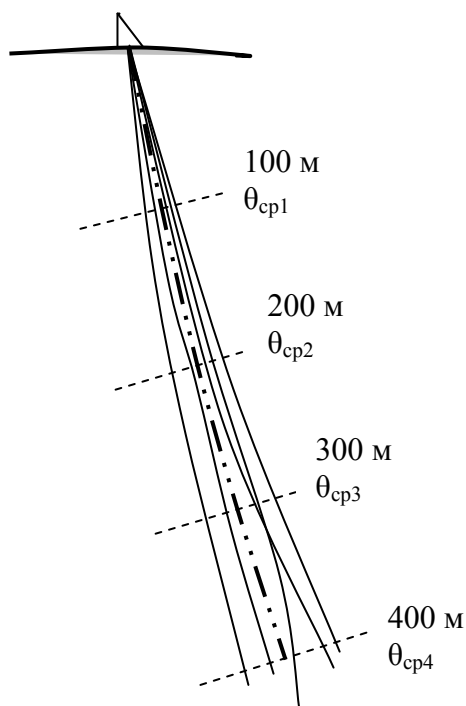
Рис.2.56. Схема расчета «типовой» кривой графическим методом
