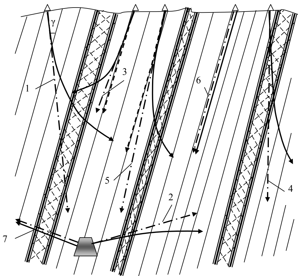
Рис. 2.48. Возможные варианты искривления скважин в апсидальной плоскости: \dashrightarrow проектное направление скважины; \rightarrow фактическое направление скважины; \dashrightarrow возможное направление скважины [ 28]
