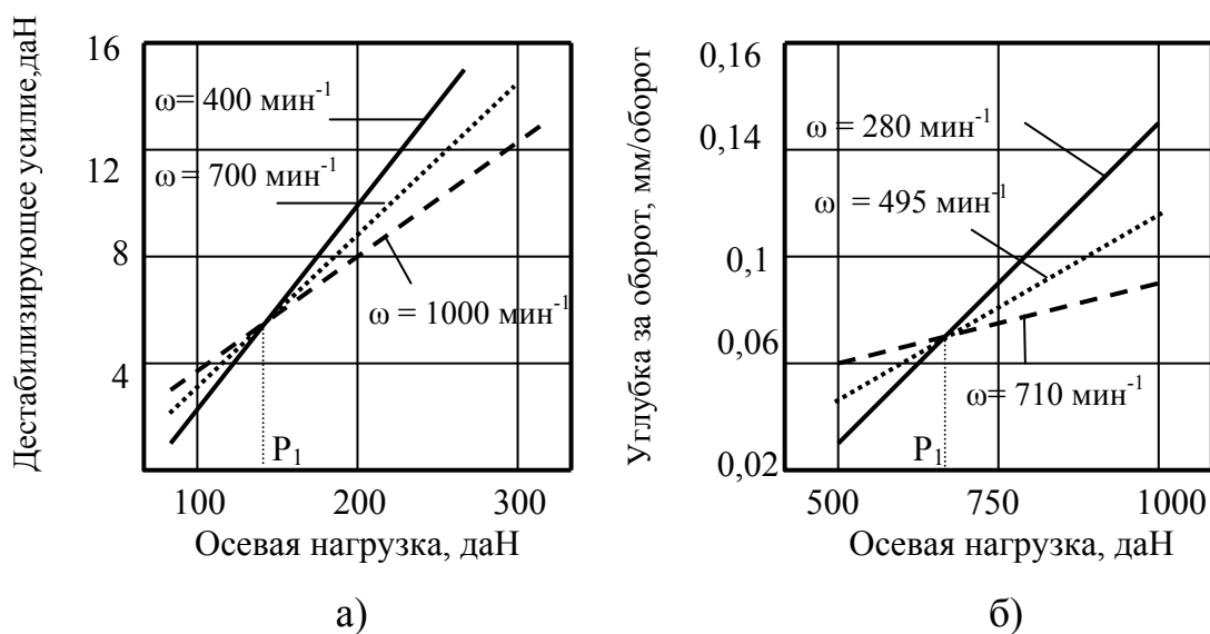
Рис.2.35. Экспериментальные зависимости дестабилизирующего усилия \Delta F (а) и углубки за оборот коронки на забое h (б) от осевого усилия при различных значениях частоты вращения инструмента
