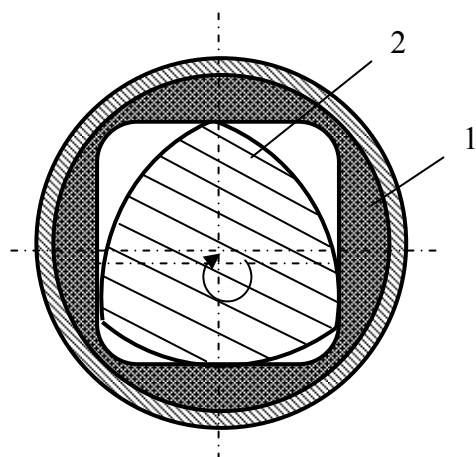
Рис.4.61. Схема поперечного сечения объемного двигателя при соотношении пары статор: ротор – 4:3
