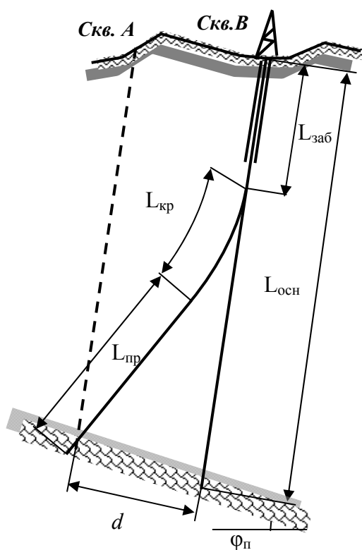
Рис. 6.3. Схема для расчета эффективности бурения скважины с дополнительным стволом
