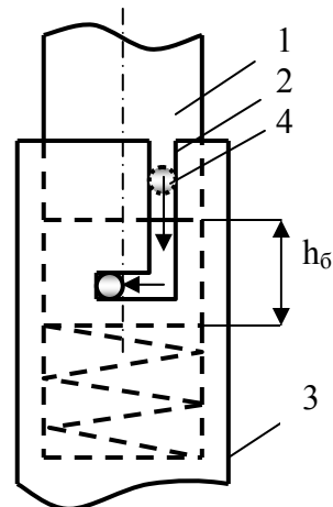
Рис.5.34 . Схема байонетного замка
