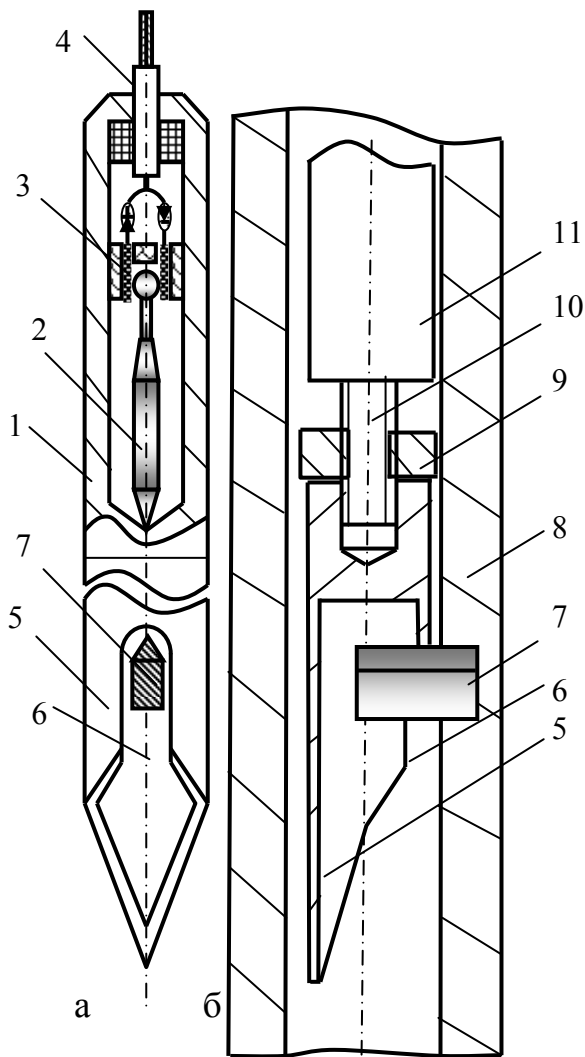
Рис.5.12 . Схема устройства ориентатора УШО (а) и положение наконечника ориентатора в переходнике над отклонителем при его ориентировании (б)
