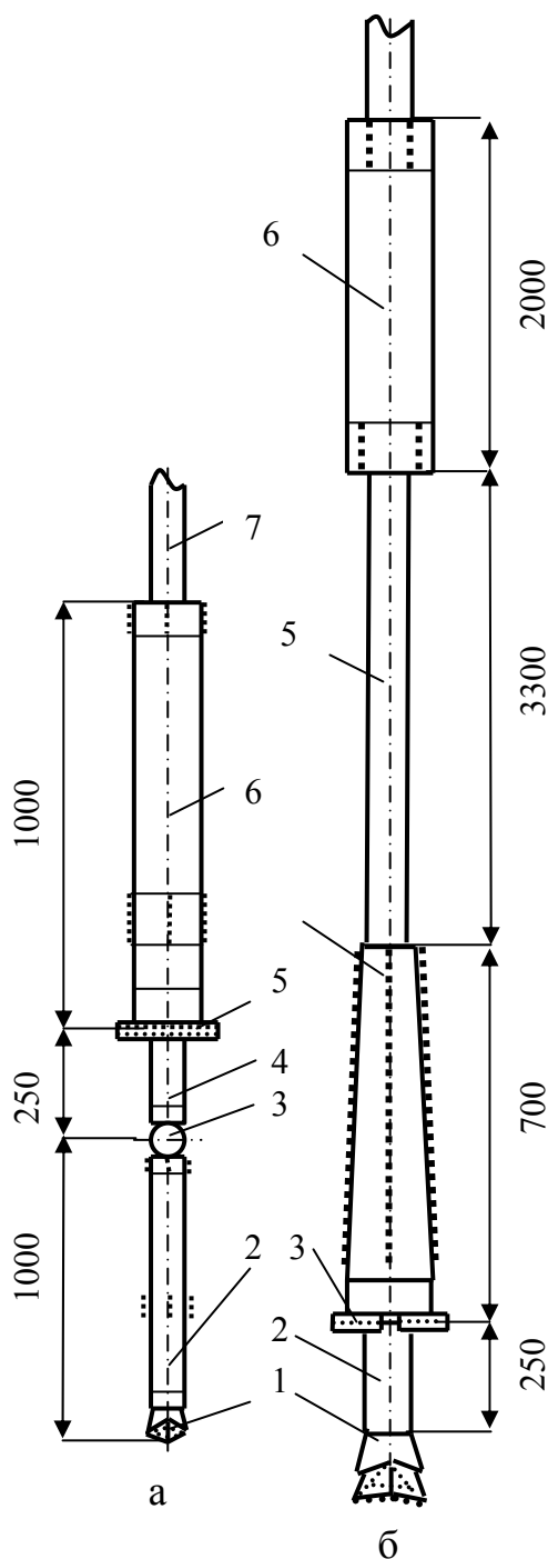
Рис.4.37. Технологические снаряды а – РШС-59/46; б- КЖК-59
