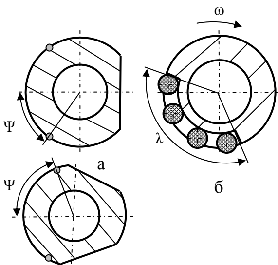
Рис. 4.5. Компоновки КСМ с опорами качения
