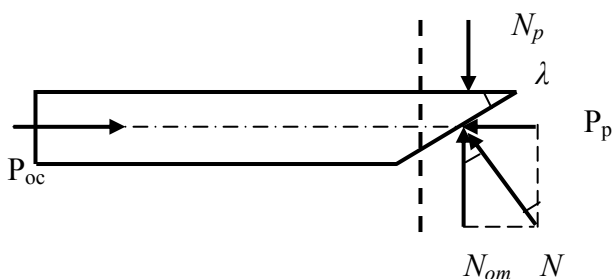
Рис.4.27. Схема сил при задавливании в грунт инструмента со скосом торца
