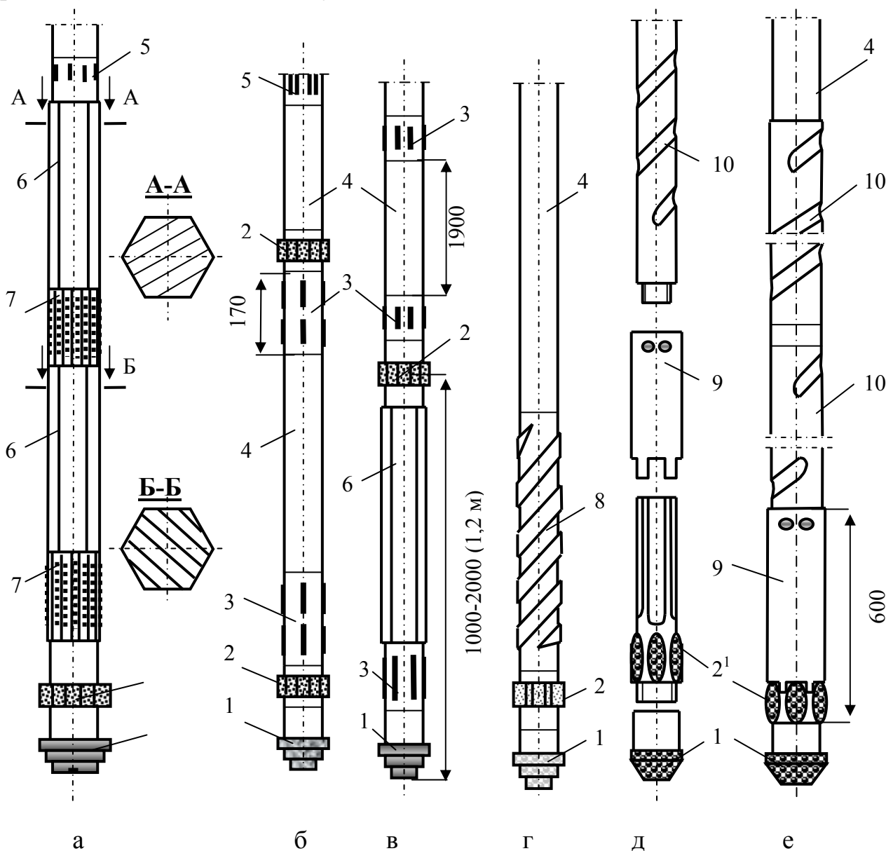
Рис.4. 7 . Схемы центрирующих (жестких) компоновок ССК
