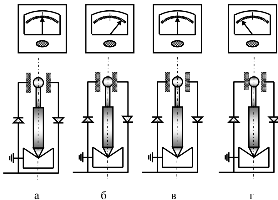
Рис.5.13. Схемы положений датчика ориентатора УШО и соответствующие этим положениям показания наземного миллиамперметра (а-г) и диаграмма, отражающая диапазоны углов поворота ориентатора вокруг своей продольной оси, соответствующие означенным положениям датчика и стрелки миллиамперметра (д)
