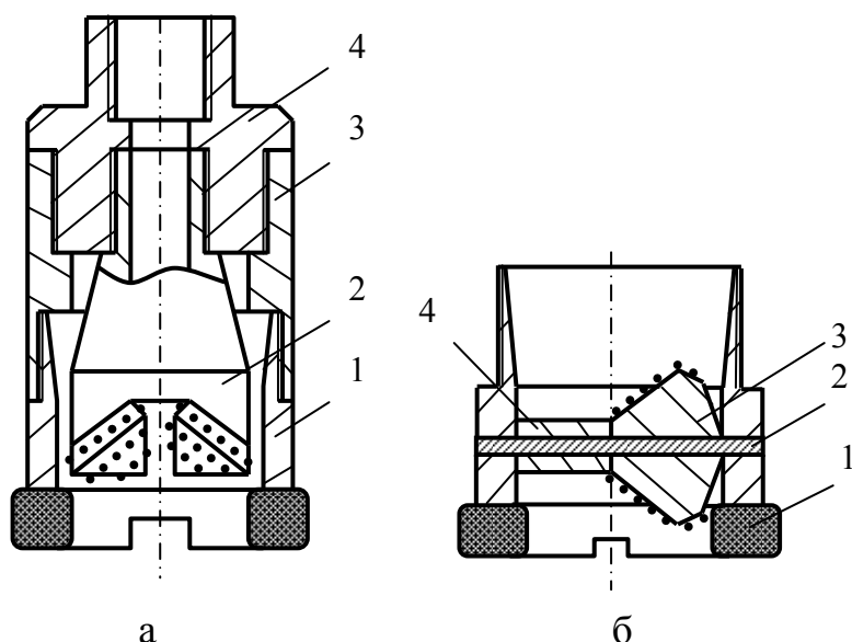
Рис.4.69. Комбинированные шарошечно-алмазные долота для искусственного искривления скважин: ДША (а) и АШК (б)
