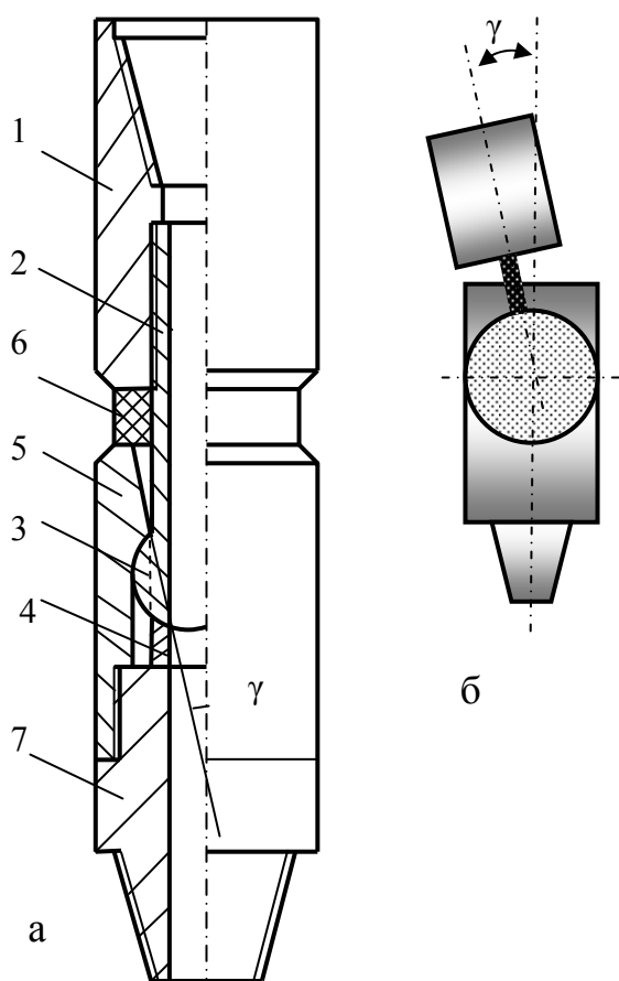
Рис.4. 23. Устройство шлицевого шарнирного соединения (переходника) - (а) и схема, поясняющая существо работы шарнирного переходника (б)
