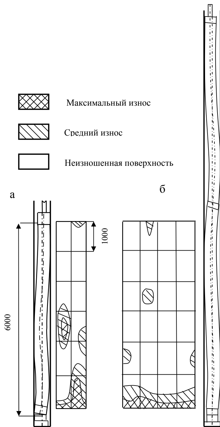
Рис. 2.9. Схемы форм деформации колонковых наборов, построенные с учетом износа колонковых труб при длине набора: а - 6 м; б - 12 м
