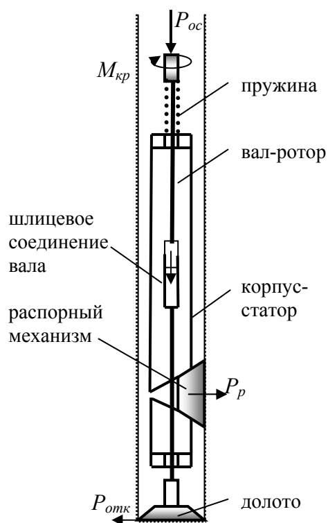
Рис.4. 42.Схема ОНД
