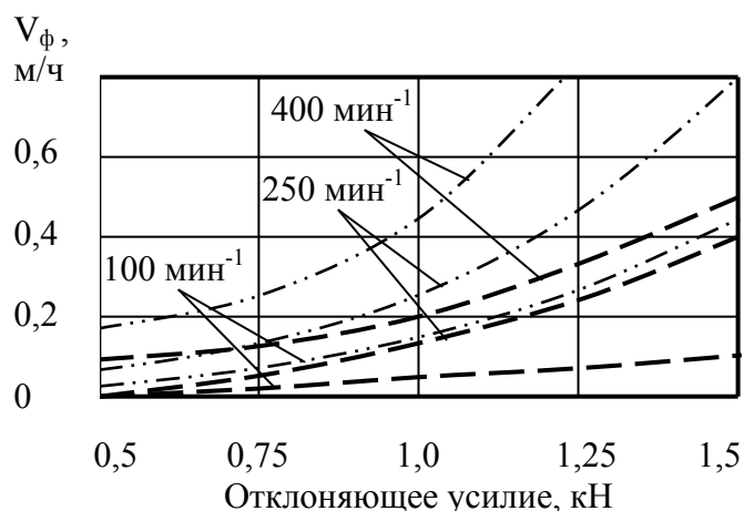
Рис.4. 70. Зависимости скорости фрезерования от отклоняющего усилия при различных значениях частоты вращения долота: штриховые линии -графики для шарошечного долота ПШ-59К-ЦА; штриховая линия с точками – графики для алмазного долота АДН-59
