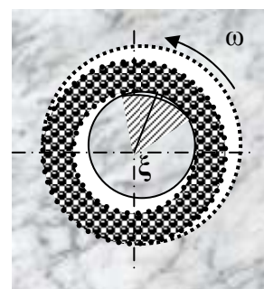
Рис.7.7. Схема нанесения метки на керн резцами коронки (вид с торца) в горизонтальной скважине
