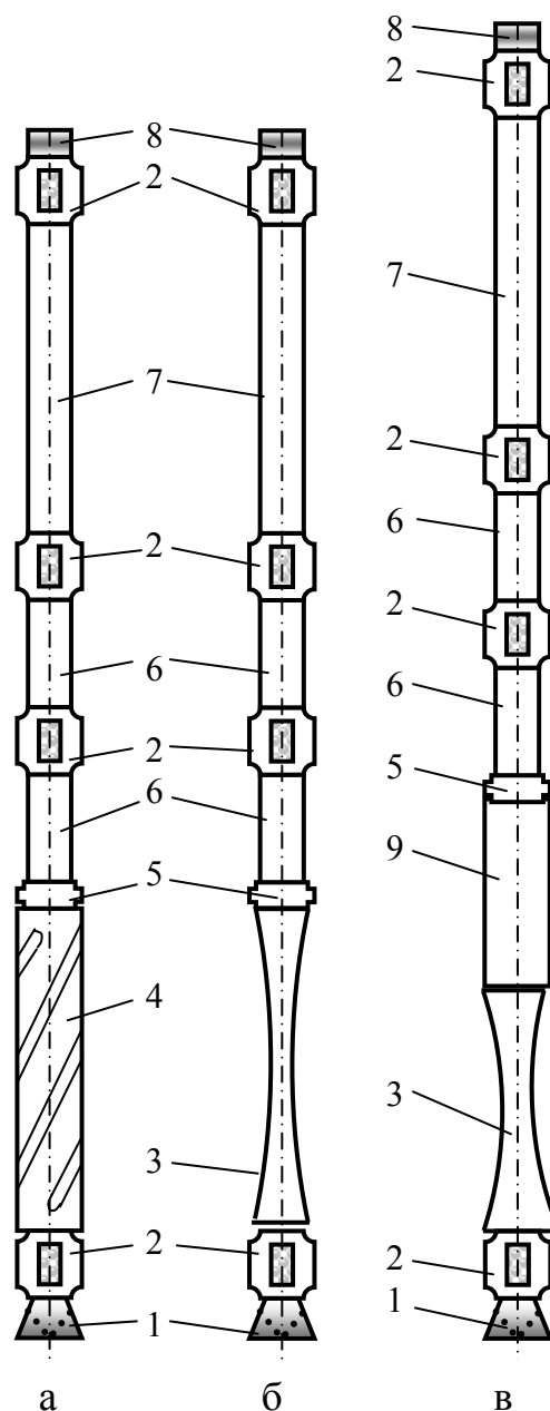
Рис.4. 15 . КНБК, применяемые при бурении скважины СГ-3: 1 – долото; 2 – центратор КЛС; 3 – ЭУБТ; 4 – УБТ со спиральной формой наружной поверхности (СУБТ); 5 –сигнализатор предельного зенитного угла СПЗУ-1; 6 – редуктор; 7 – забойный двигатель; 8 – забойный датчик частоты вращения забойного двигателя; 9 – керноотборочный снаряд
