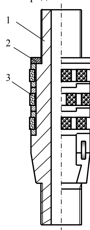
Рис.4.74. Калибратор КАНБ: 1 – корпус; 2 – зажимная шайба; 3 – кольцо с алмазосодержащими штабиками
