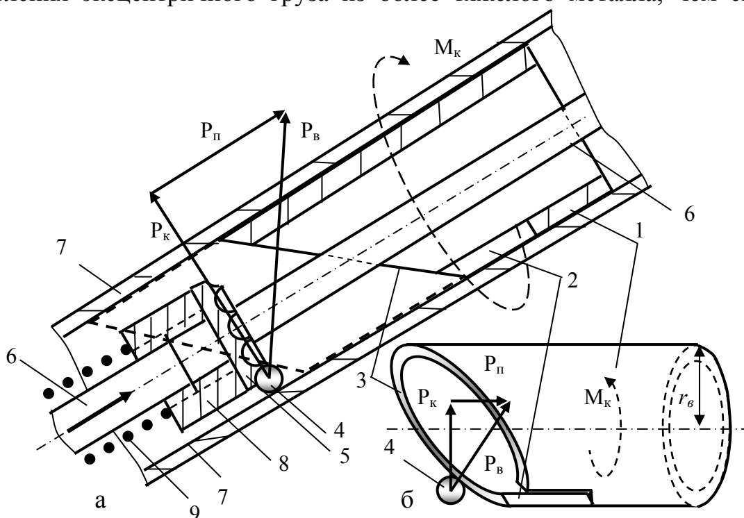
Рис.5.10. Примерная схема ориентирующего узла отклонителя «КЕДР»: а – момент ориентирования при отрыве отклонителя от забоя наклонной скважины (корзина 5 с шариком 4 под действием пружины 9 перемещается вверх и надвигается на винтовую поверхность 3 стакана 1, проворачивая стакан 1 и корпус 6 отклонителя в заданное при настройке ориентатора и отклонителя угол установки; б – стакан 1 с пазом 2 и винтовой поверхностью 3 рабочего торца при взаимодействии с шариком 4
