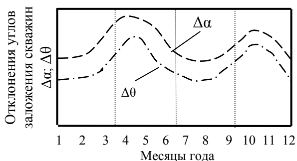
Рис.2.1. График сезонных колебаний величин отклонений от проектных значений углов заложения скважин
