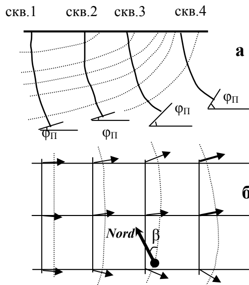
Рис. 2.57. Геологический разрез (а) и план (б) участка работ с траекториями пробуренных на участке скважин
