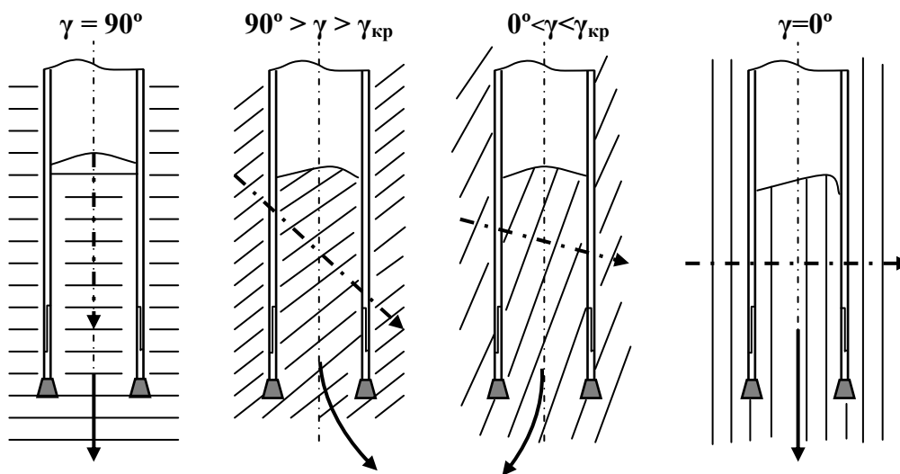
Рис. 2. 47. Схемы направлений зенитных искривлений скважин в анизотропных горных породах в зависимости от угла встречи \gamma со слоистостью или сланцеватостью [18].
