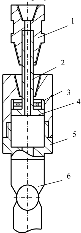
Рис.4.34. Приставка для ориентации стационарного клина в наклонной скважине
