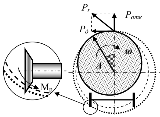
Рис.4.67. Схема, поясняющая процесс отклонения плоскости набора кривизны под действием дезориентирующего усилия P_d
