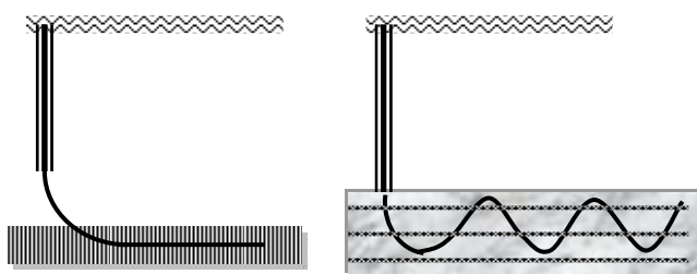
Рис.8.3. Варианты вскрытия коллекторов горизонтальным и волнообразным стволами
