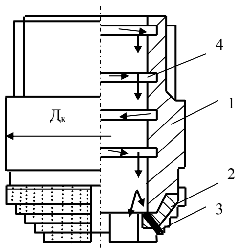
Рис.2.19. Виброактивная коронка К16-0 и схема движения потока промывочной жидкости в ней: 1 – корпус; 2 – матрица; 3 – отверстие в матрице с генерирующей ультразвуковые колебания пластиной; 4 – проточка
