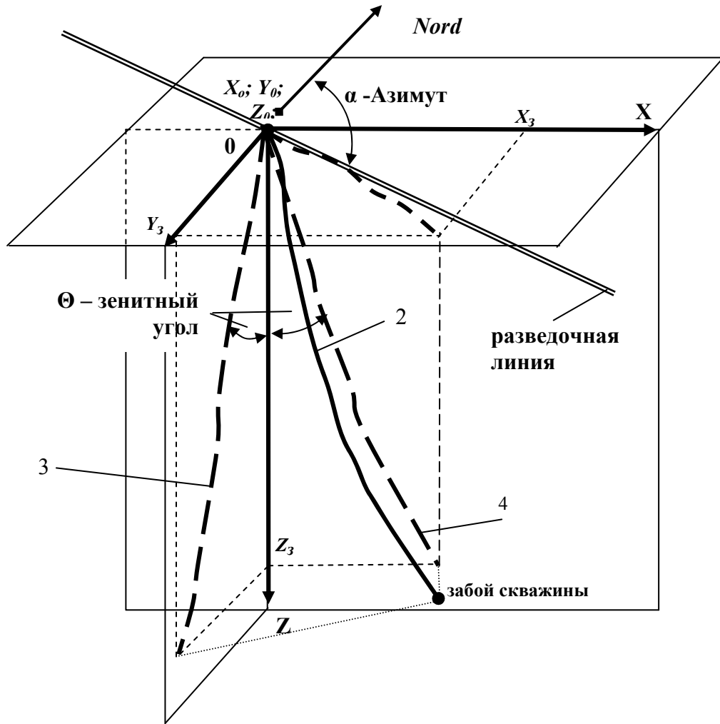
Рис.1.1. Графическое изображение скважины в декартовой системе координат:
