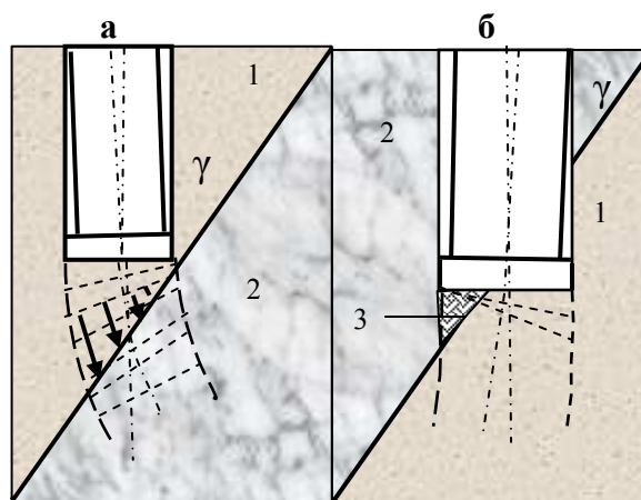
Рис.2.44. Схемы перехода инструмента из мягкой (1) в твердую (2) породу (а) и наоборот (б): 3 – участок скальваемой твердой породы и образование уступа
