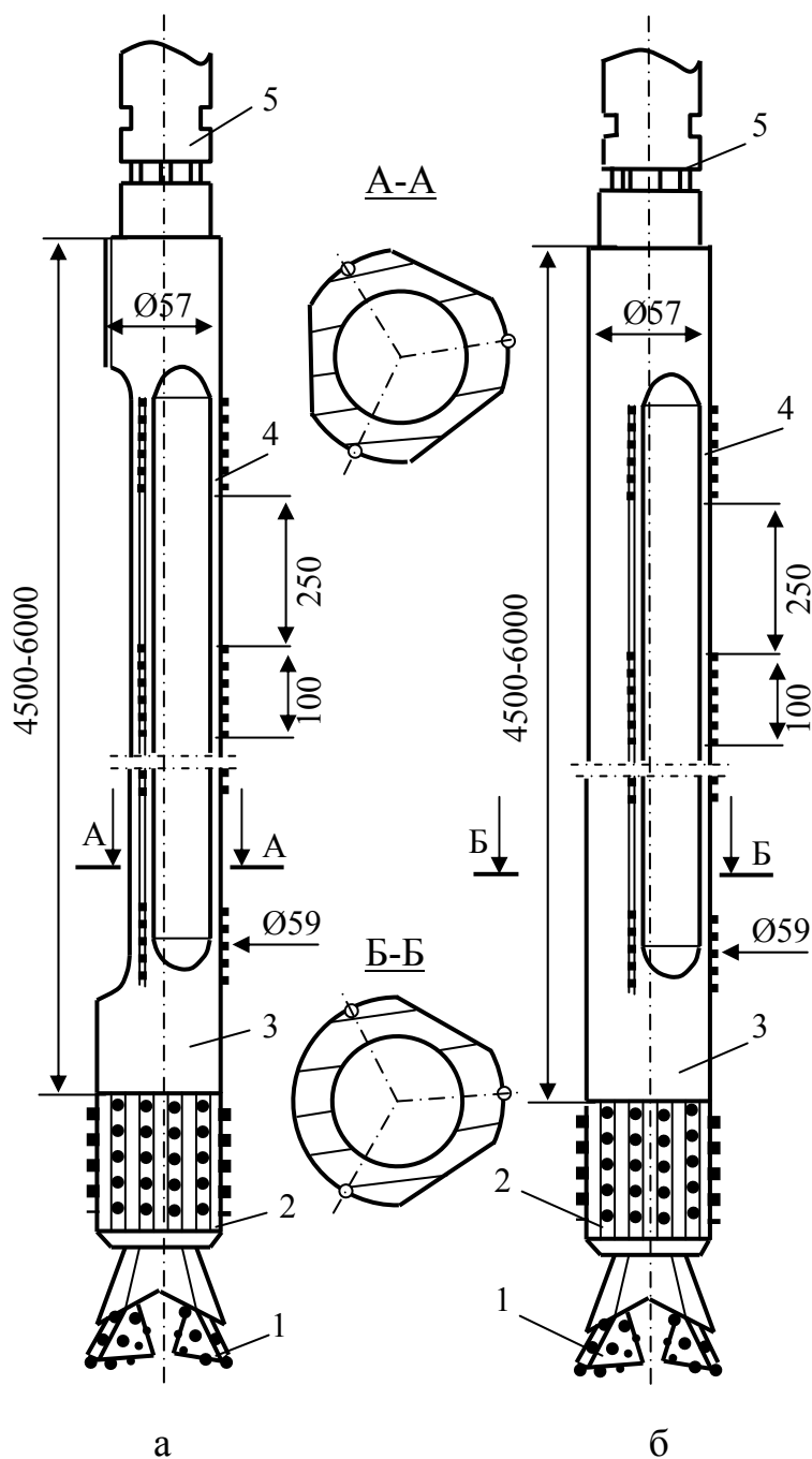
Рис. 4.16. Схемы компоновок для бурения шарошечными долотами: 1 - долото; 2 - центратор; 3 – трехгранный стабилизатор (сечение А-А) или труба со смещенным центром тяжести поперечного сечения (сечение Б-Б); 4 – центрирующие элементы; 5 – гидроударник ГВ
