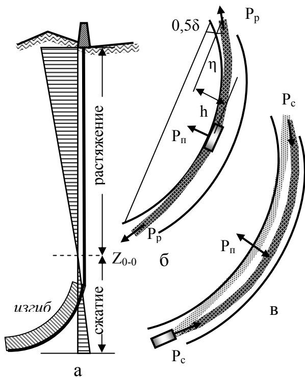
Рис.5. 27 . Схемы для анализа условий работы бурильной колонны в искривленном стволе скважины: а – эпюры напряжений материала бурильной колонны; б – положение растянутого; в – сжатого участка колонны в искривленном стволе
