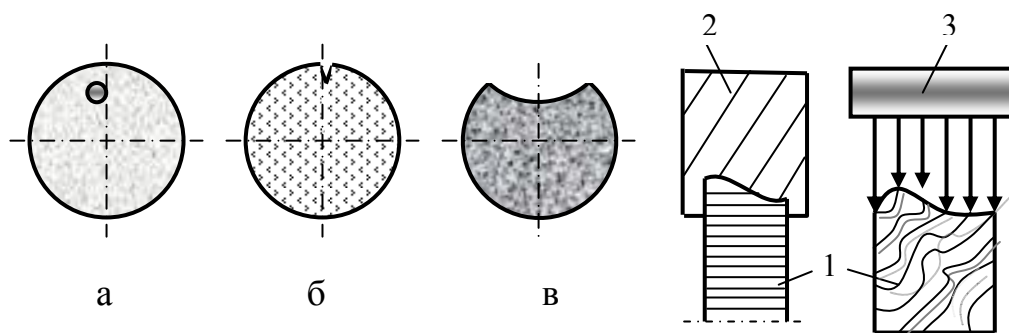
Рис. 7.2. Схемы кернов с метками: 1 – керн; 2 – печать; 3 – механический копир
