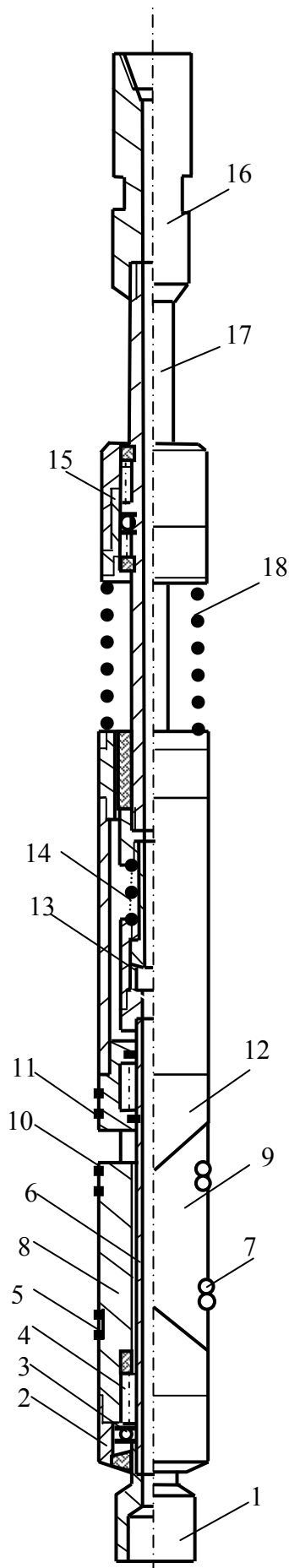
Рис.4.48. Отклонитель ТЗ-3П-59
