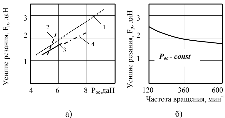
Рис.2.34. Экспериментальные зависимости усилия резания единичным алмазным резцом от соевого усилия на резец (а) и частоты вращения (б): 1 - частота вращения \omega = 120 \text{ мин}^{-1} ; 2 - 375; 3-500; 4 - 700 \text{мин}^{-1}
