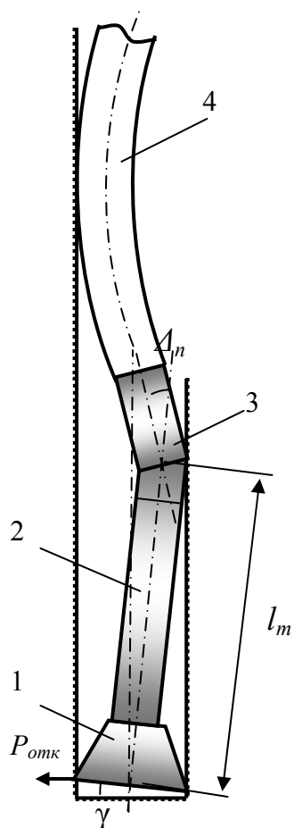
Рис.4.46. Схема, поясняющая процесс искривления скважины при совпадении направлений фрезерования стенки скважины под действием P_{отк} и перекоса породоразрушающего инструмента на примере ОНД на базе забойного двигателя с кривым переходником:
