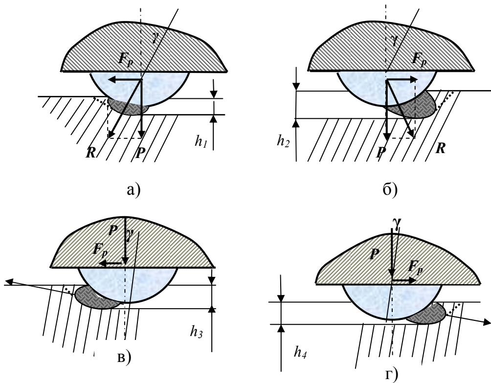
Рис.2.32. Схема для анализа процесса резания-скалывания-раздавливания анизотропной горной породы алмазными резцами при перемещении их по забою навстречу восстания слоистости или сланцеватости (а, в) и в направлении слоистости или сланцеватости породы (б,г) при угле встречи \gamma > \gamma_{кр} (а,б) и угле встречи \gamma \leq \gamma_{кр} (в,г)
