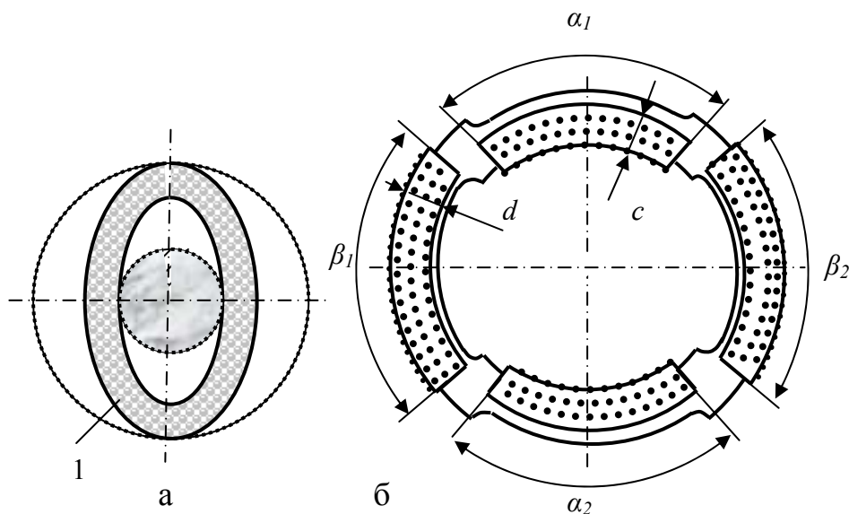
Рис.4.18. Торцевые формы эллиптической коронки 1 (а) и коронки с наружными и внутренними секторами матрицы (б)
