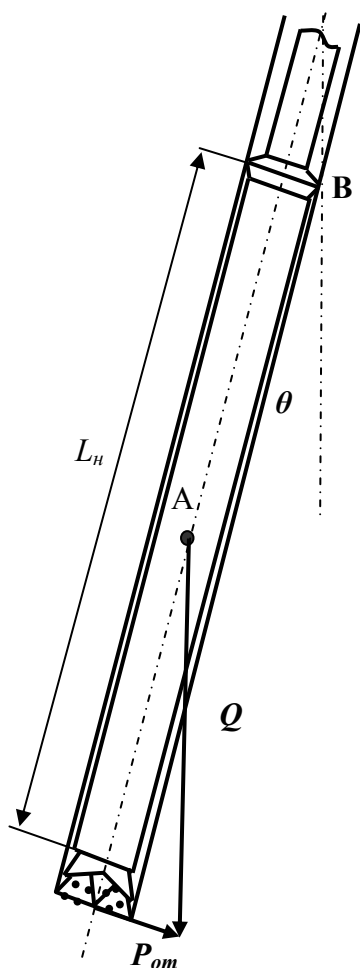
Рис.4.10. Схема для пояснения работы «маятниковой» компоновки по уменьшению зенитного угла
