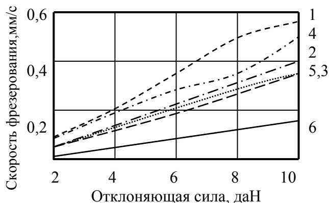
Рис.2.16. Зависимость скорости фрезерования от отклоняющей силы при частоте вращения 645 мин -1 коронкой 01АЗД40К40 диаметром 46 мм горных пород: 1 – известняк, V категория; 2 – аргиллит, VI кат.; 3 – алевропесчаник, VII кат.; 4 – туф, VIII кат.; 5 – окварцованный алевролит, IX кат.; 6 – окварцованный песчаник X кат
