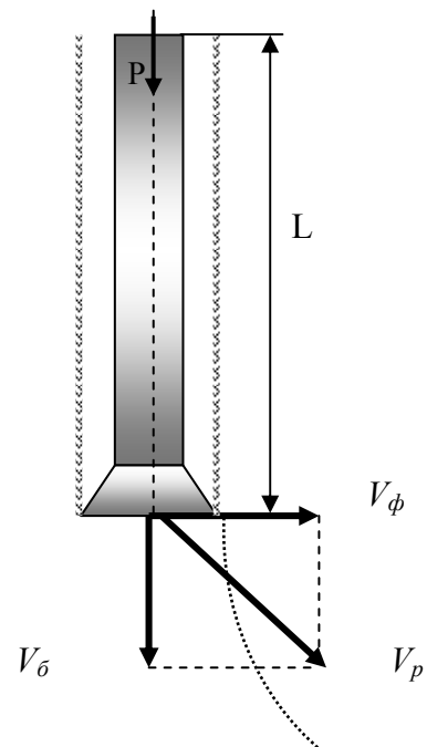
Рис.2.14.Схема, поясняющая процесс фрезерования стенки скважины
