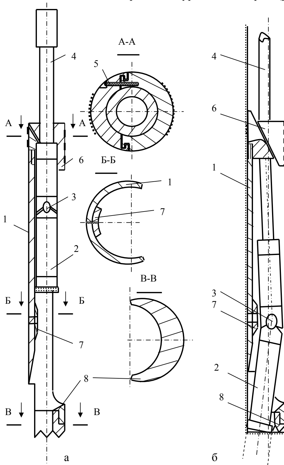
Рис. 4. 39. Конструктивная схема отклонителя СОАЭРУ-59/46 а – при спуске в скважину; б – в рабочем положении
