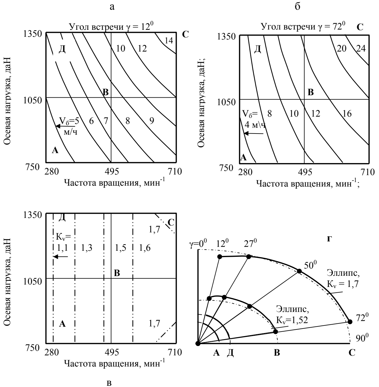
Рис.2.24. Результаты бурения анизотропного туфо-дацита:
