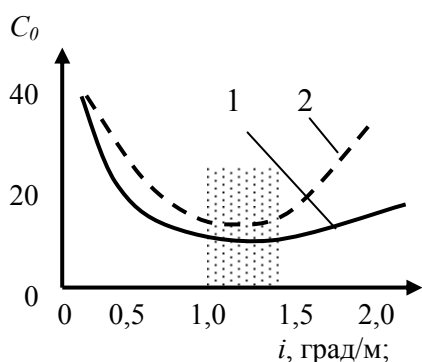
Рис.5.23. Зависимость стоимости градуса искривления ( C_0 ) от интенсивности искривления ( i ): 1 – СБТ; 2 – ЛБТ
