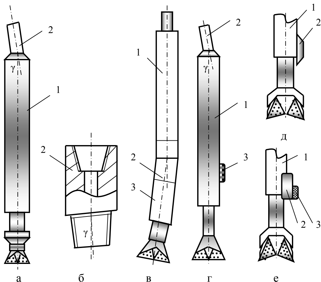
Рис.4.60. Схемы отклонителей на базе забойных гидродвигателей
