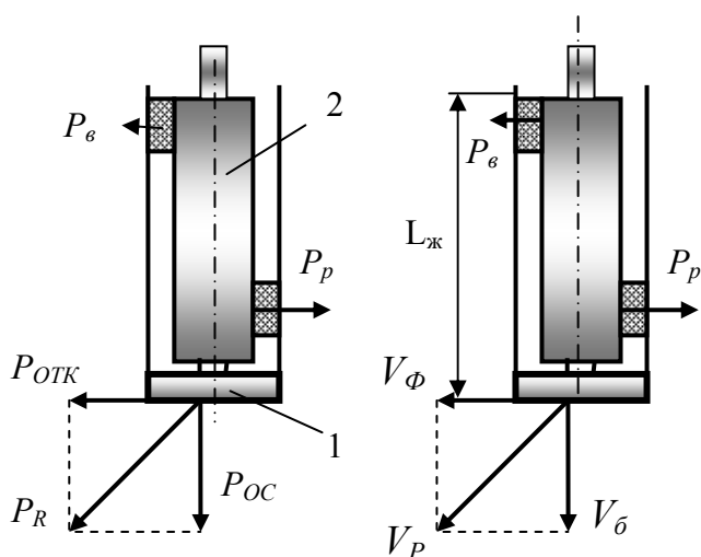
Рис.4.44. Схемы, поясняющие процесс набора кривизны фрезерованием стенки скважины под действием отклоняющего усилия P_{OTK} 1 – породоразрушающий инструмент; 2 – корпус ОНД
