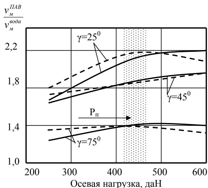
Рис.2.38. Экспериментальные зависимости прироста механической скорости бурения от осевого усилия и угла встречи \gamma с плоскостями флюидалности туфо-дацита: при частоте вращения 560 мин -1 (сплошные линии); 355 мин -1 (пунктирные линии)
