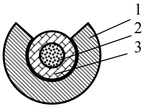
Рис.3. 5. Схема размещения кабеля внутри труб при доставке инклинометра в горизонтальную скважину
