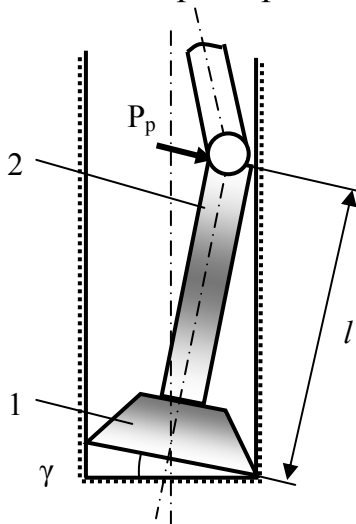
Рис.4.43. Схема набора кривизны ОНД асимметричного разрушения забоя 1 – породоразрушающий инструмент; 2 – корпус ОНД
