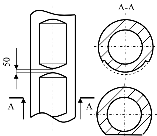
Рис.4. 8 . Варианты выполнения колонковой трубы со смещенным центром тяжести поперечного сечения
