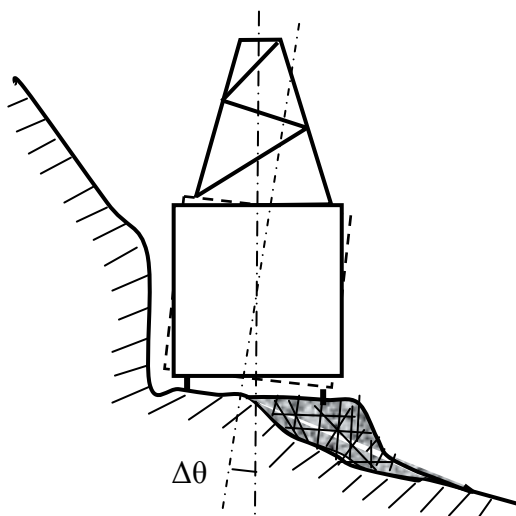
Рис.2.2. Схема, поясняющая одну из причин отклонений углов заложения скважин от проектных значений
