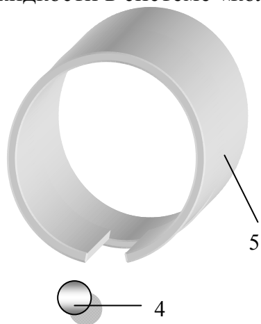
Рис.5.18. Втулка с шариком ориентатора ОШГ
