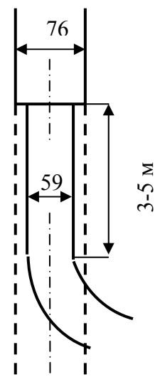
Рис.5.35. Схема забуривания дополнительного ствола спрямлением
