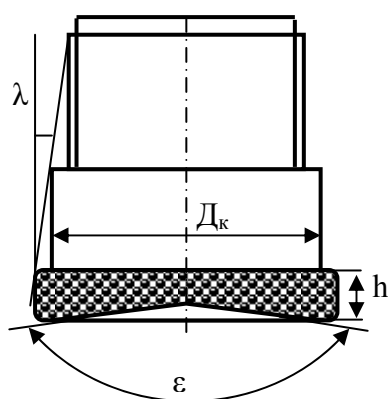
Рис.4.68. Параметры алмазного долота
