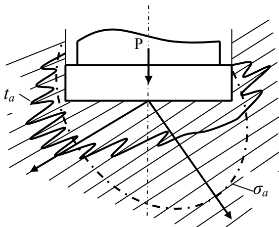
Рис.2.51. Схема для оценки влияния термомеханического бурения на искривление скважин в анизотропных породах
