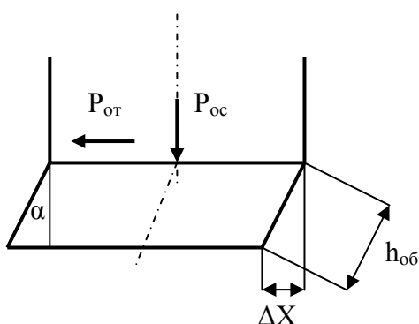
Рис. 2.15. Схема для расчета угла отклонения скважины под действием усилия P_{от}
