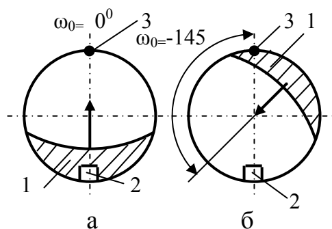
Рис.5.19. Схемы установки ложка 1 клинового отклонителя относительно нулевой метки ориентатора ОШГ (2 – паз втулки; 3 – метка на корпусе) под углами установки 0^\circ (а) и -145^\circ (б)
