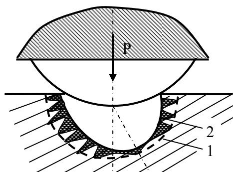
Рис.2.37. Схема формирования зоны предразрушения в анизотропной породе: 1 – границы ядра сжатия в породе; 2 – зона предразрушения
