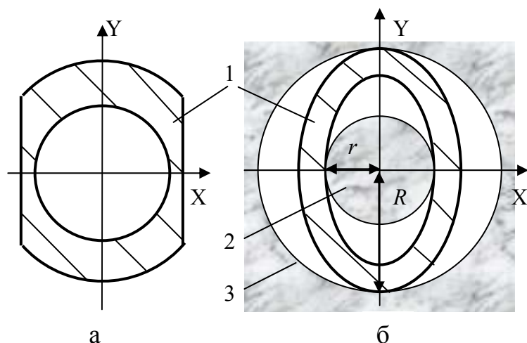
Рис. 4.6. Схемы поперечных сечений компоновок с неравной жесткостью по осям поперечного сечения – 1; 2 – керн; 3 – ствол скважины
