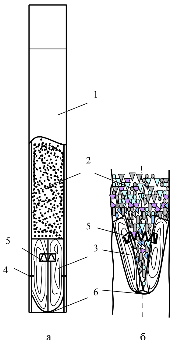
Рис.4.30. Контейнер с щебнем и деревянной пробкой для создания временного забоя (а) и положение деревянной пробки в скважине после выдавливания из контейнера (б)
