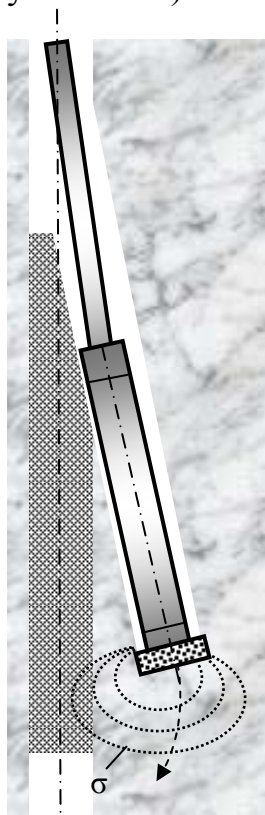
Рис.5. 30. Схема забуривания дополнительного ствола
