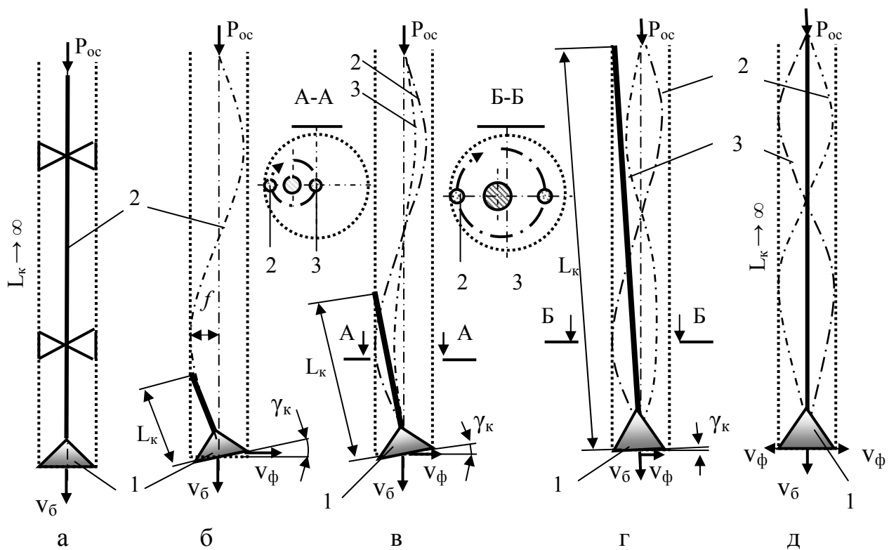
Рис.2. 18. Схемы для анализа влияния основных факторов на процесс естественного искривления скважины при вращательном бурении
