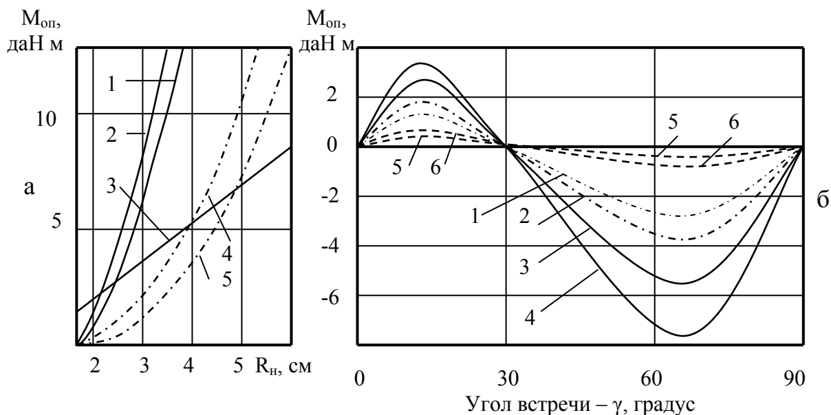
Рис. 2.30. Зависимости опрокидывающего момента от технико-технологических и геологических условий
