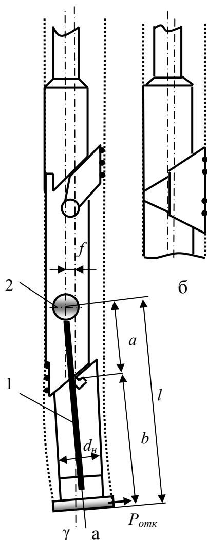
Рис.4.55. Схема отклонителя СБС в рабочем состоянии (а) и схема верхнего распорного узла отклонителя СБС (б)
