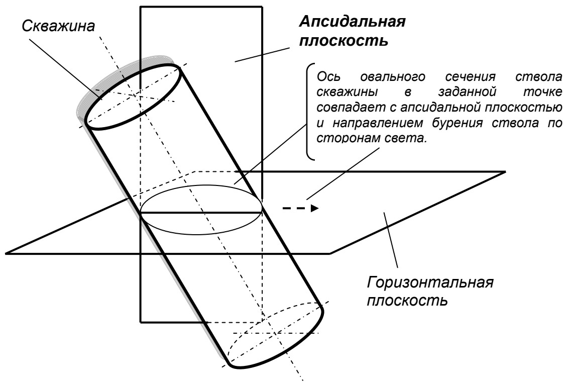
Рис.1.5. Графическое определение апсидальной плоскости.
