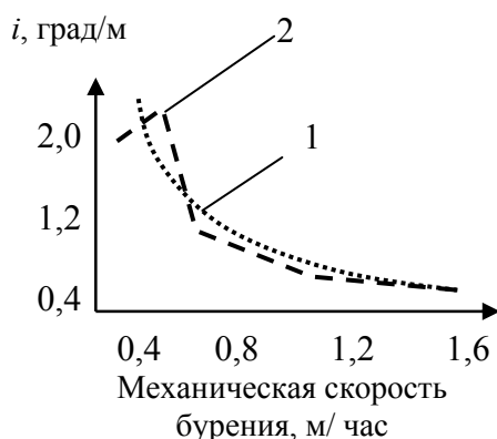
Рис.4.56. Зависимость интенсивности искривления от механической скорости бурения отклонителем СБС: 1 – теоретическая зависимость; 2 – зависимость, полученная по данным бурения
