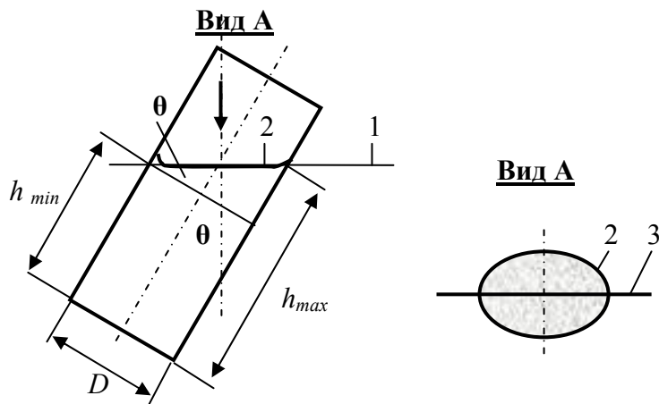
Рис.3.1. Схема определения зенитного угла \theta и положения апсидальной плоскости скважины в жидкостном стеклянном асидоскопе: 1 – горизонтальная линия; 2 – след уровня плавиковой кислоты, зафиксированный в точке замера в скважине; 3 – положение апсидальной плоскости
