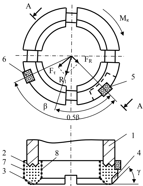
Рис.4. 21. Базированная алмазная коронка
