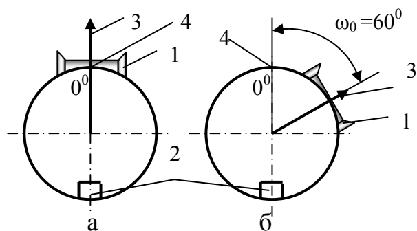
Рис.5.11. Схемы настройки отклонителя «КЕДР» на угол установки 0° (а) и 60° (б):
