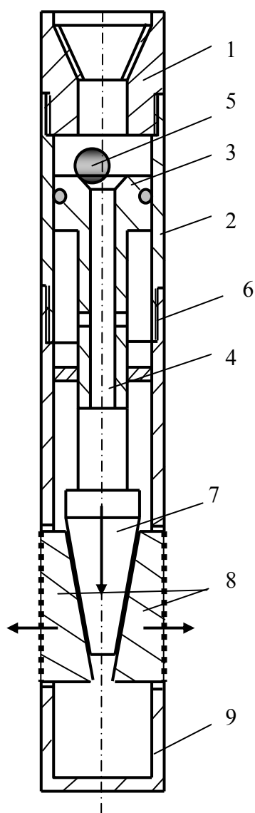
Рис.4.32. Пробка-забой
