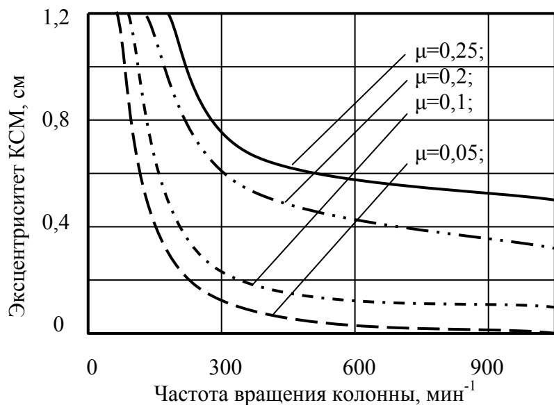
Рис. 4.4. Расчетные графические зависимости эксцентриситета буровой компоновки от частоты вращения колонны, коэффициента трения колонны о стенку скважины и величины опрокидывающего момента M_{оп}
