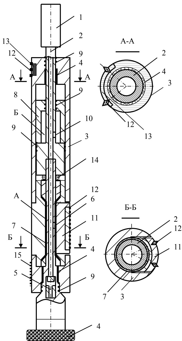
Рис.4. 51. Отклонитель ОГМ-59
