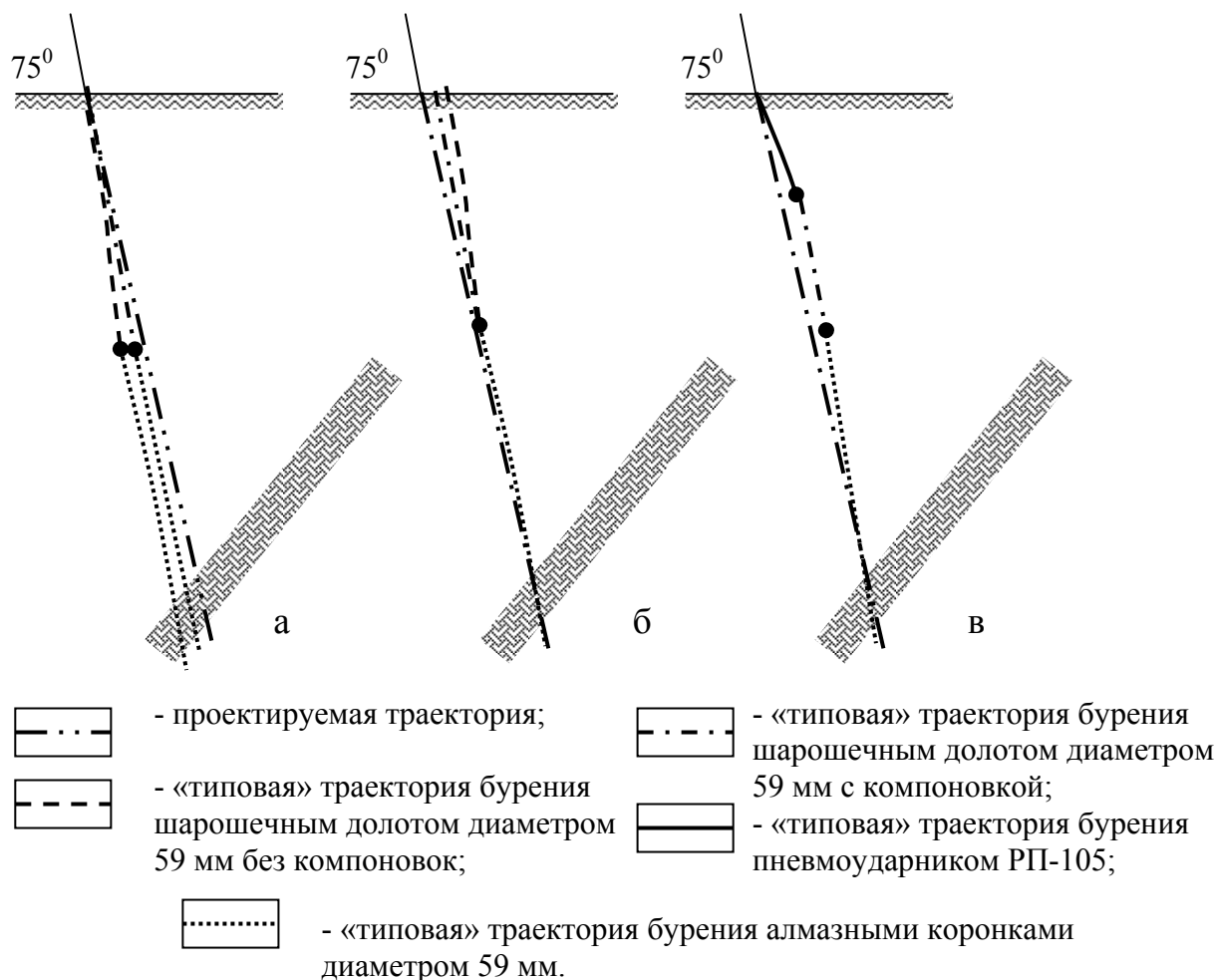
Рис.5. 38. Схемы вариантов проектирования траекторий наклонно-направленных скважин: а – исходная, с «типичными» траекториями шарошечно-алмазного бурения и корректировкой отклонителями (корректировки отклонителями не показаны); б – заложение скважины с учетом «типичных» траекторий шарошечно-алмазного бурения с применением и без применения буровых компоновок для снижения искривления при бурении шарошечными долотами; в – бурение скважины с применением пневмударника РП-105, шарошечно-алмазного бурения и соответствующей технологий управления направлением скважины
