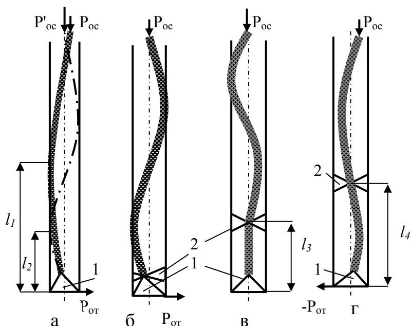
Рис.4.13. Схемы, поясняющие принцип работы КНБК с системой центраторов
