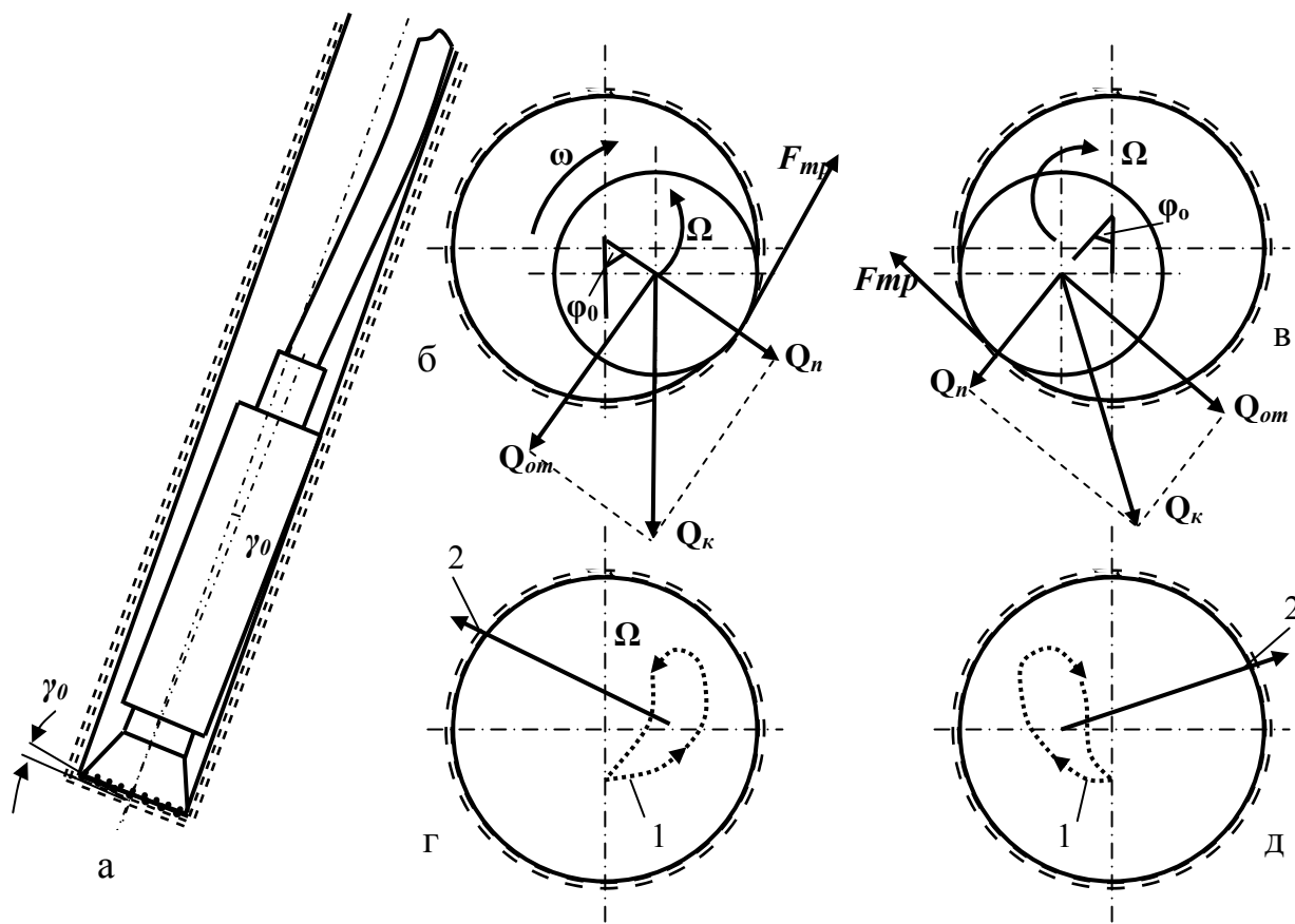
Рис.2.20. Схема к анализу механизма работы компоновки с пневмоударником в наклонной скважине:
