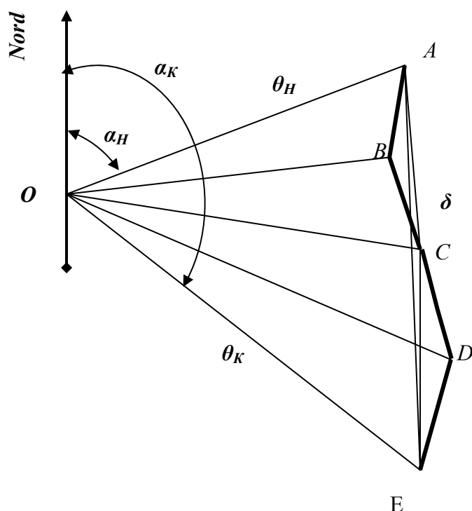
Рис.1.4. Векторная диаграмма (годограф) искривления скважины: OA , OB , OC , OD , OE - значения зенитных углов скважины, представленные в линейном масштабе, например, 1 см = 1°; AE - усредненный пространственный угол искривления скважины на интервале бурения от точки A до точки E
