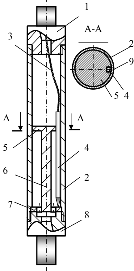
Рис.5.4. Ориентатор ШОК
