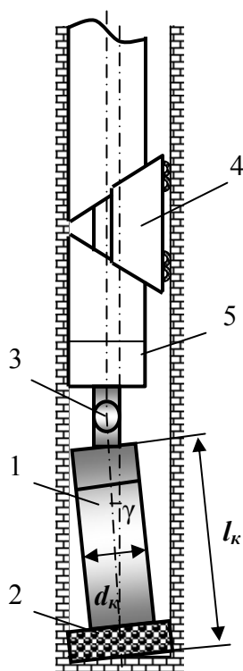
Рис.4.57. Схема отклонителя ТЗ-3 с колонковой трубой в скважине в рабочем положении
