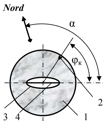
Рис.7.5. Схема для определения апсидального угла керноскопа \varphi_k и его соотношение с азимутальным углом \alpha : 1 – керн; 2 - метка; 3 – проекция следа уровня жидкости на стержне апсидоскопа на торцевую поверхность керна; 4 – направление апсидальной плоскости
