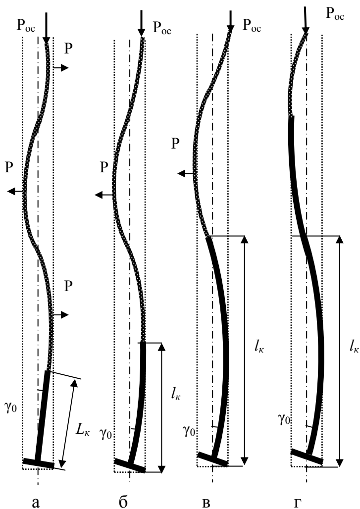
Рис.2.3. Схемы деформирования нижней части бурильной колонны при различной длине колонкового набора
