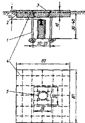
Рис. 38. Наружное оформление мест расположения пункты триангуляции, полигонометрии, триангуляции 2, 3, 4 класса на незастроенной территории.
